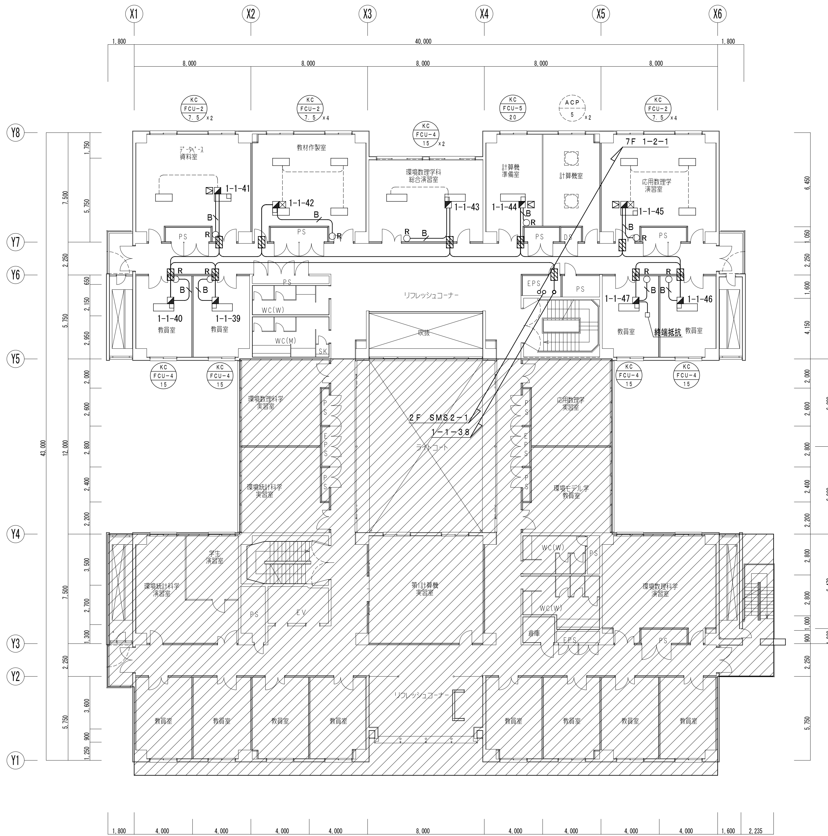
6階平面図 (改修後) 1/150
