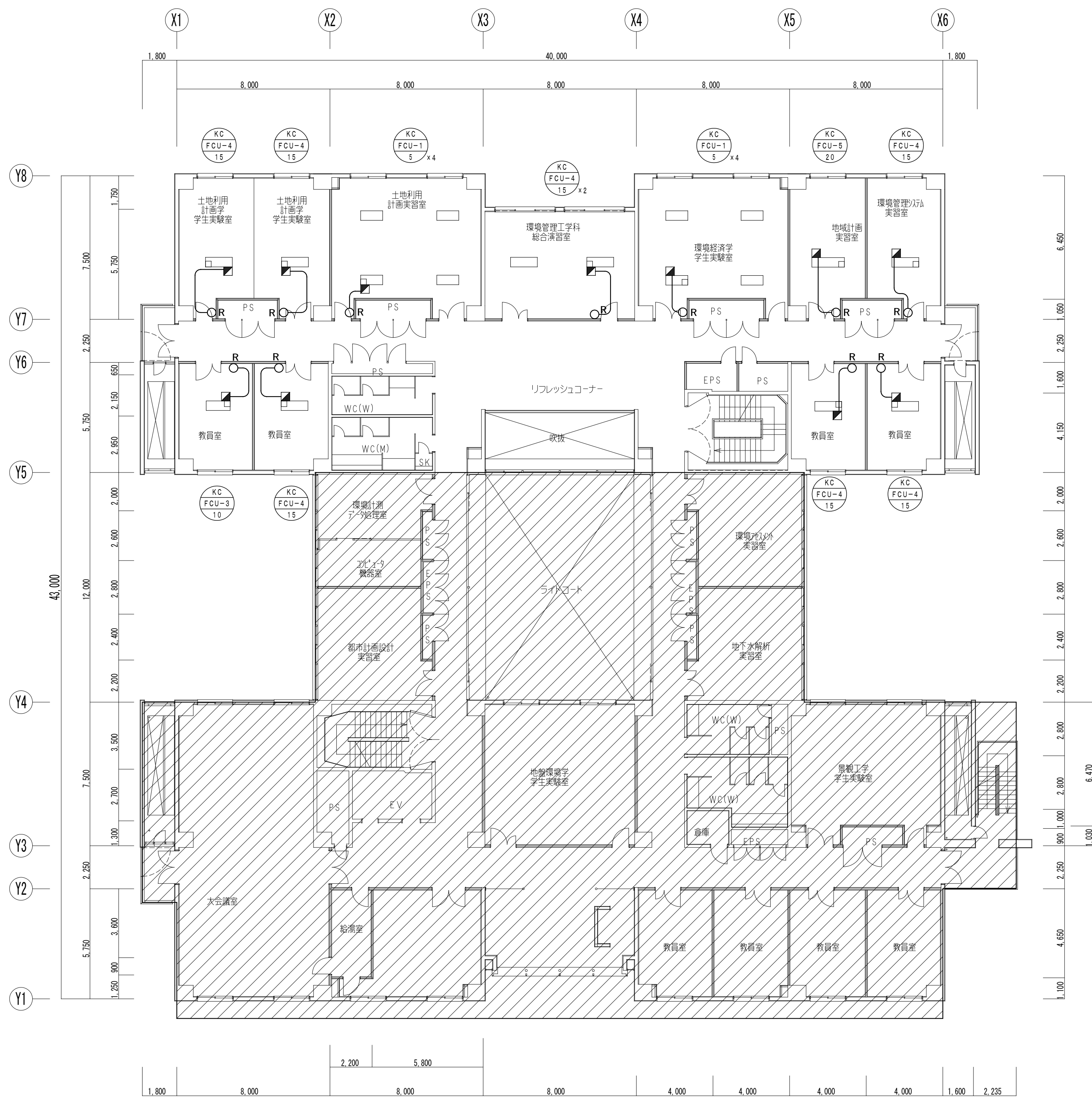
4階平面図 (改修前) 1/150
