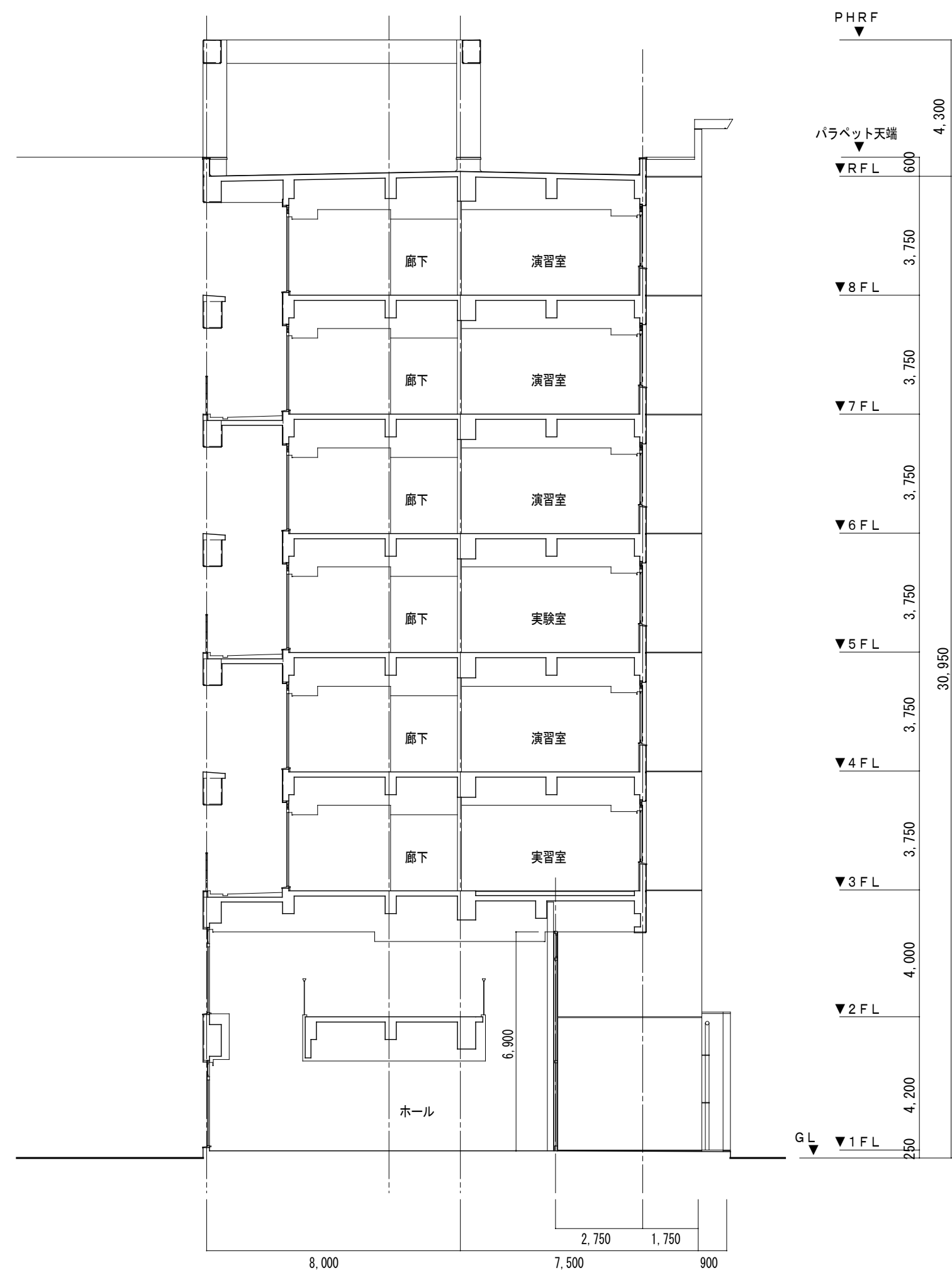
(B)-(B) 断面図 S=1/150
