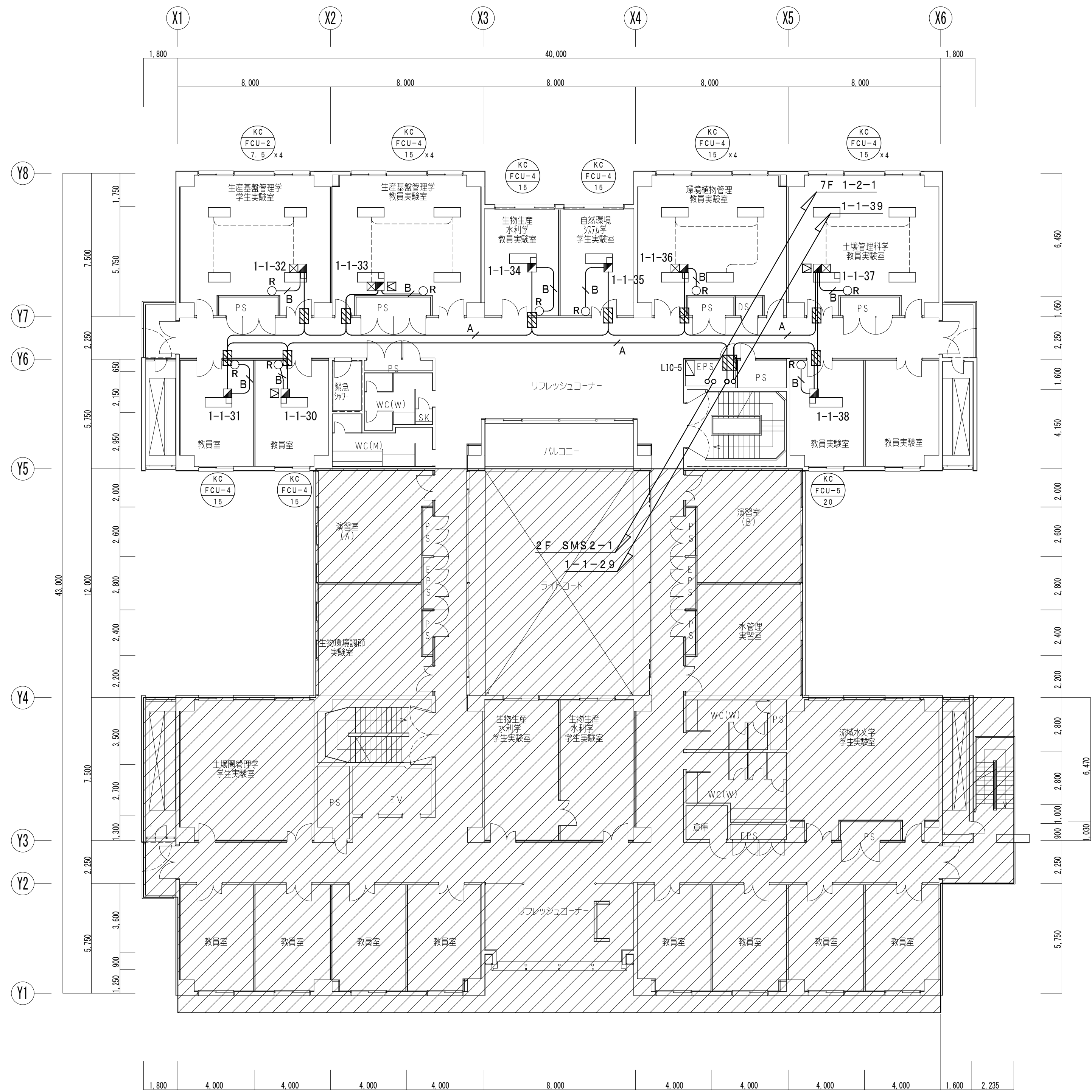
5階平面図 (改修後) 1/150
