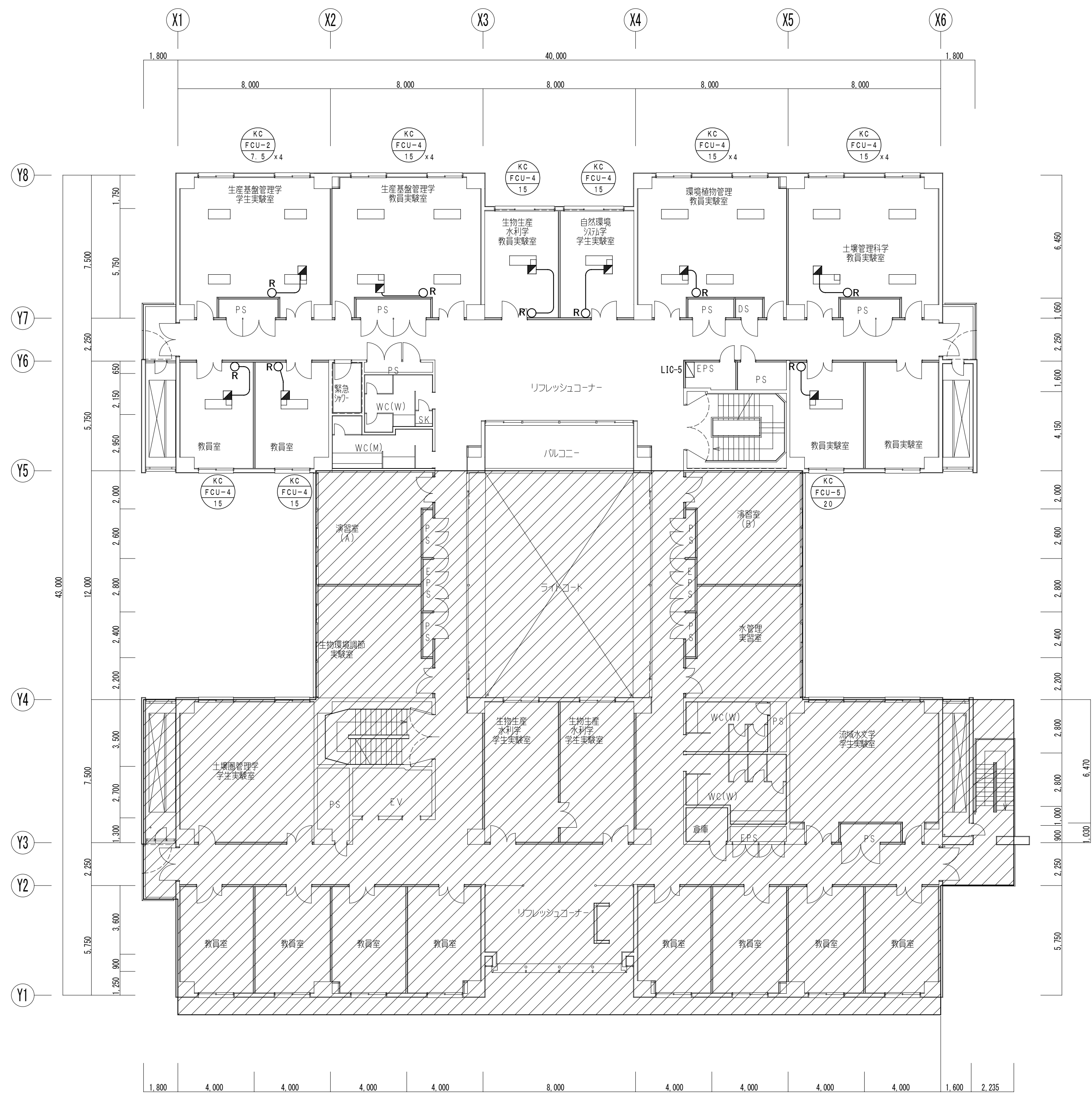
5階平面図 (改修前) 1/150
