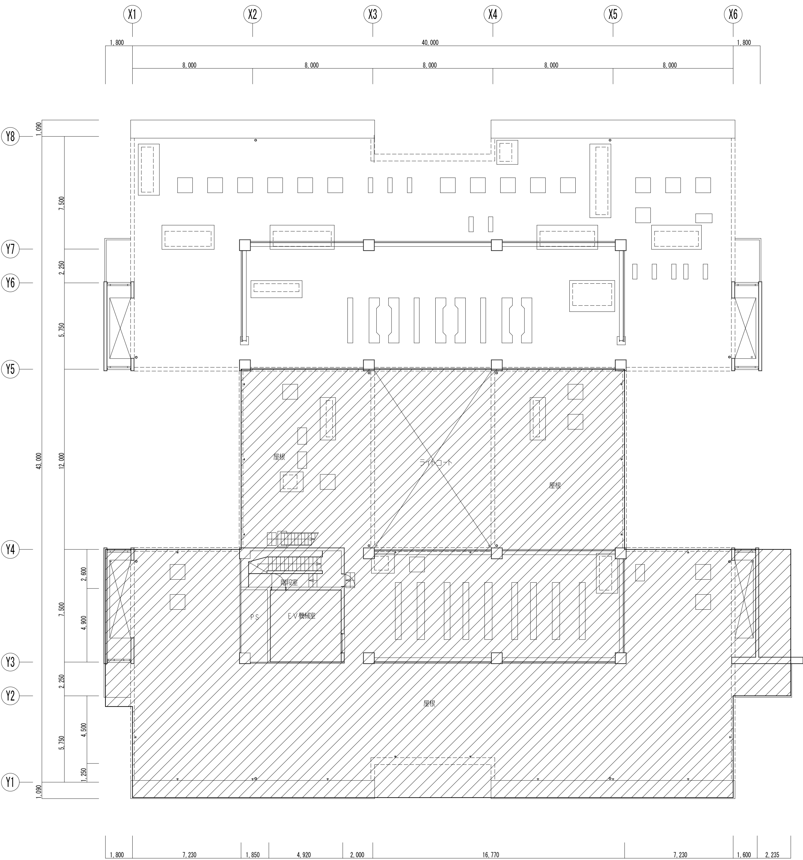
R階平面図 (改修前) 1/150
