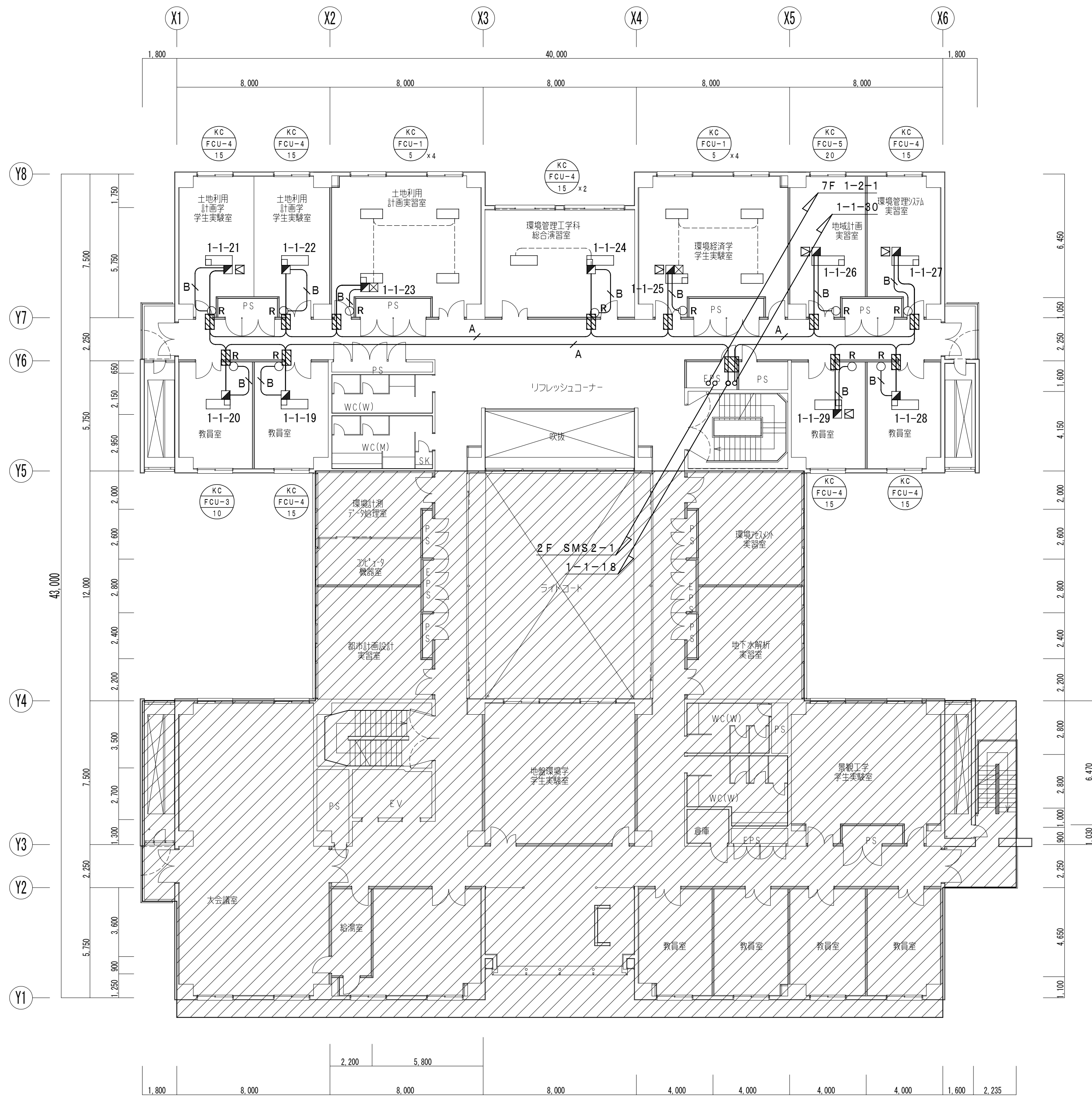
4階平面図 (改修後) 1/150
