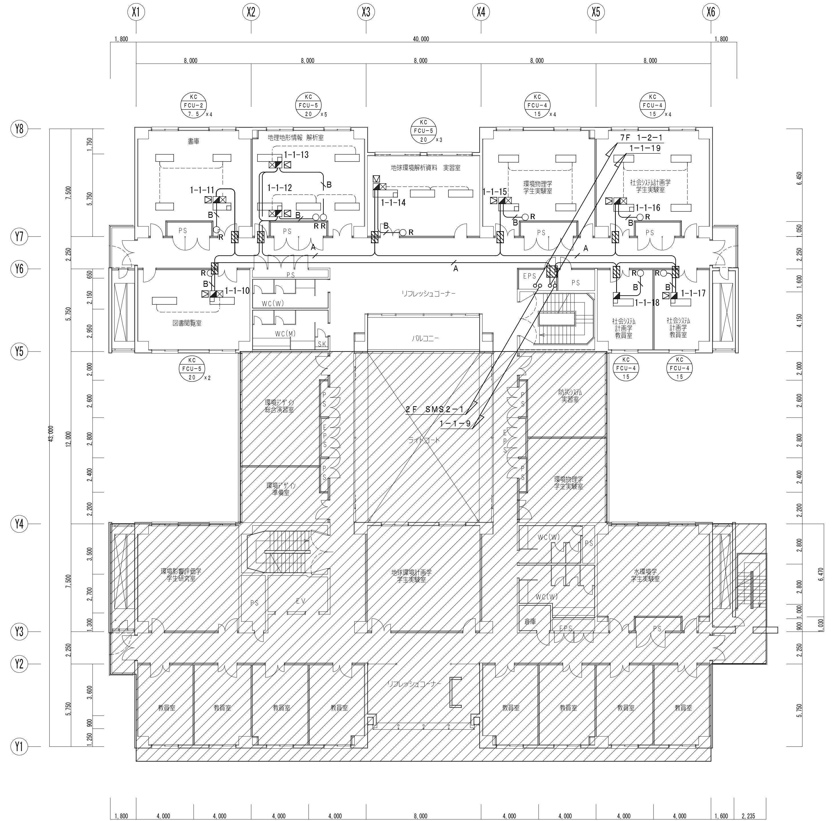
3階平面図 (改修後) 1/150
