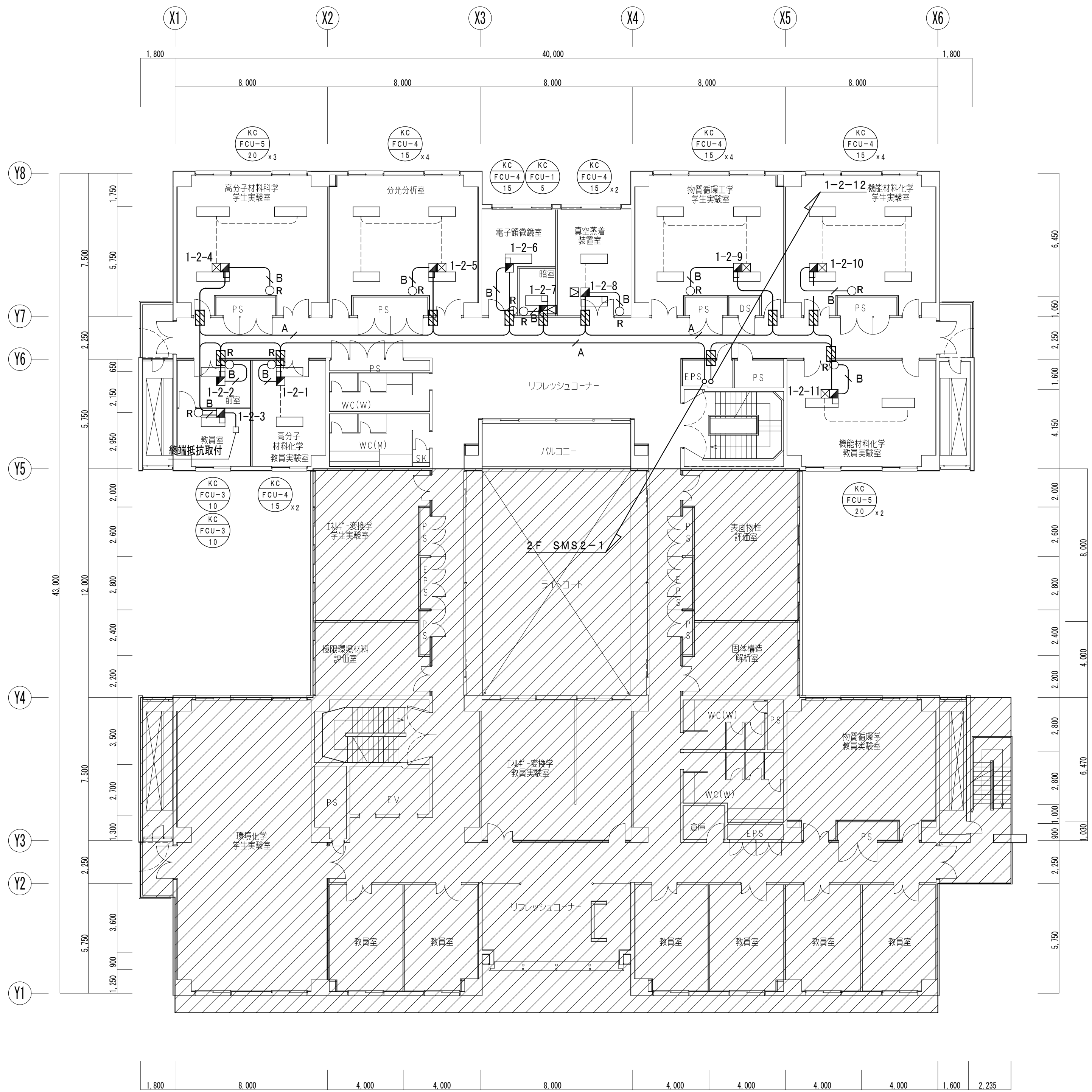
7階平面図 (改修後) 1/150
