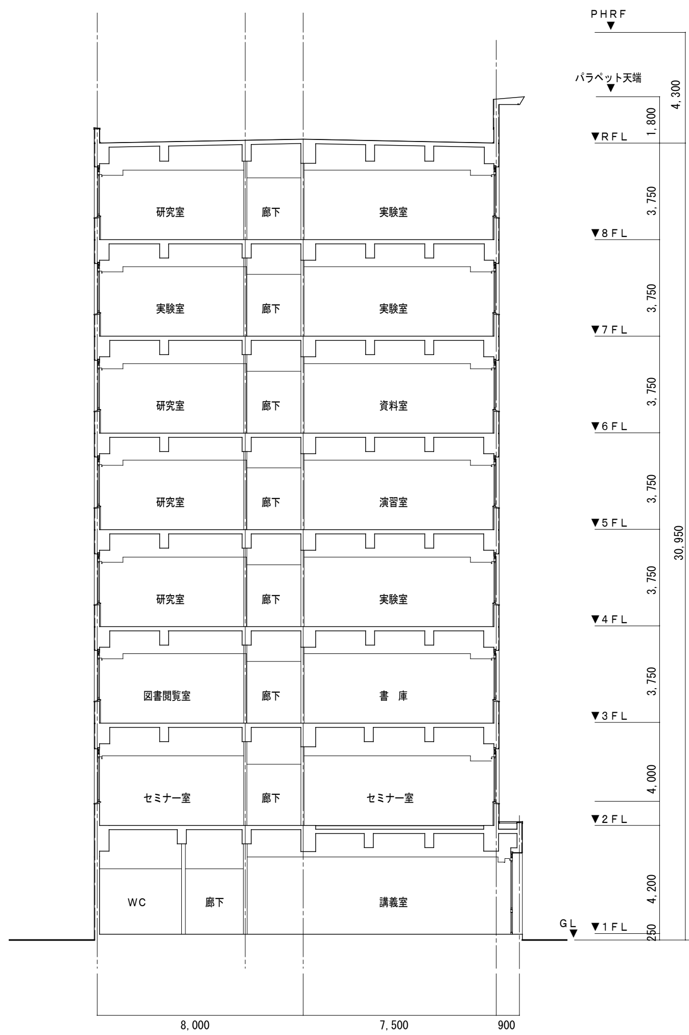
(A)-(A) 断面図 S=1/150
