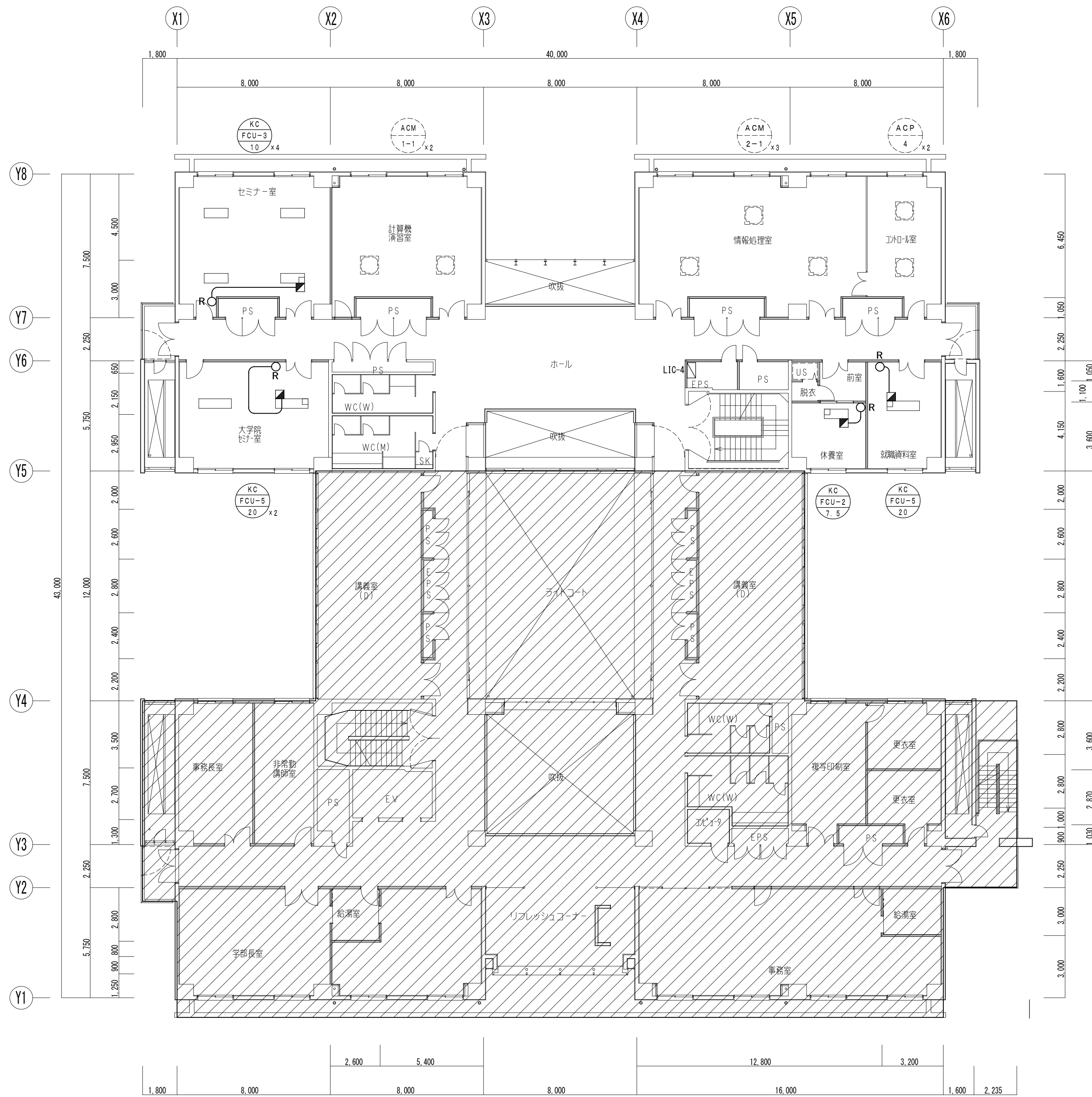
2階平面図 (改修前) 1/150
