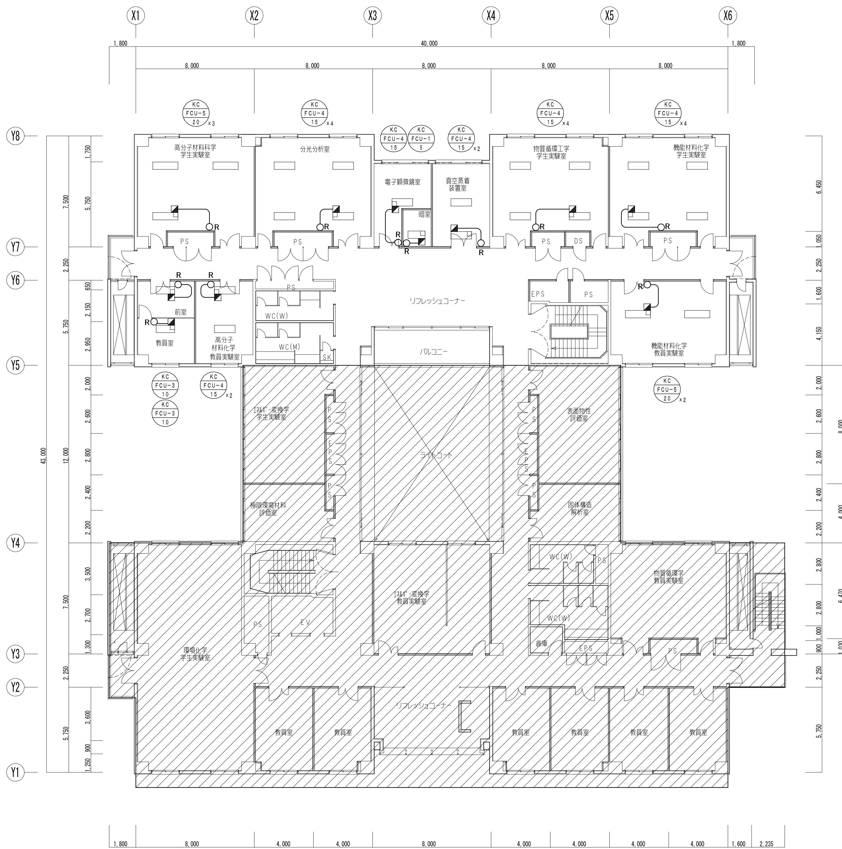
7階平面図 (改修前) 1/150
