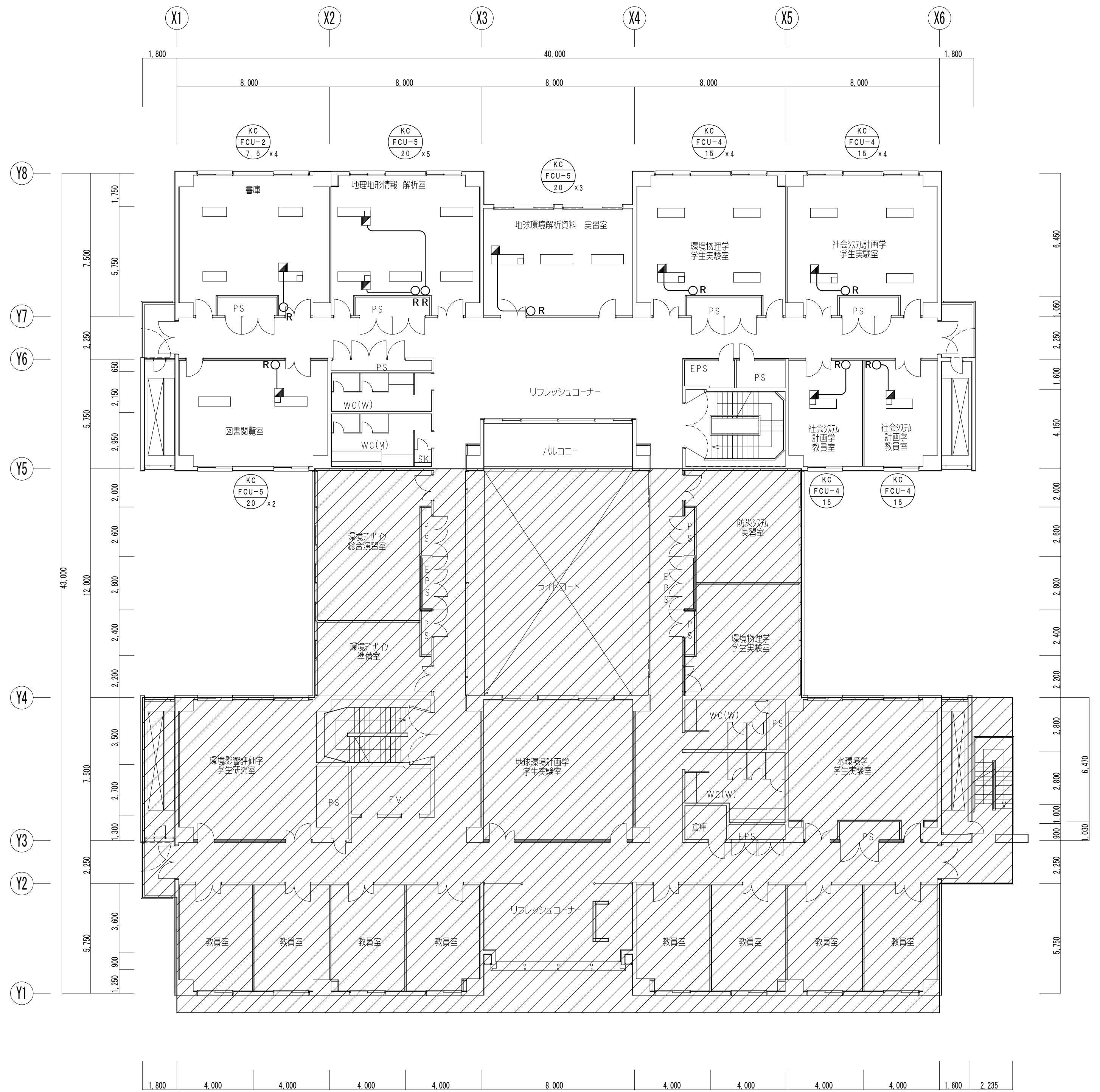
3階平面図 (改修前) 1/150
