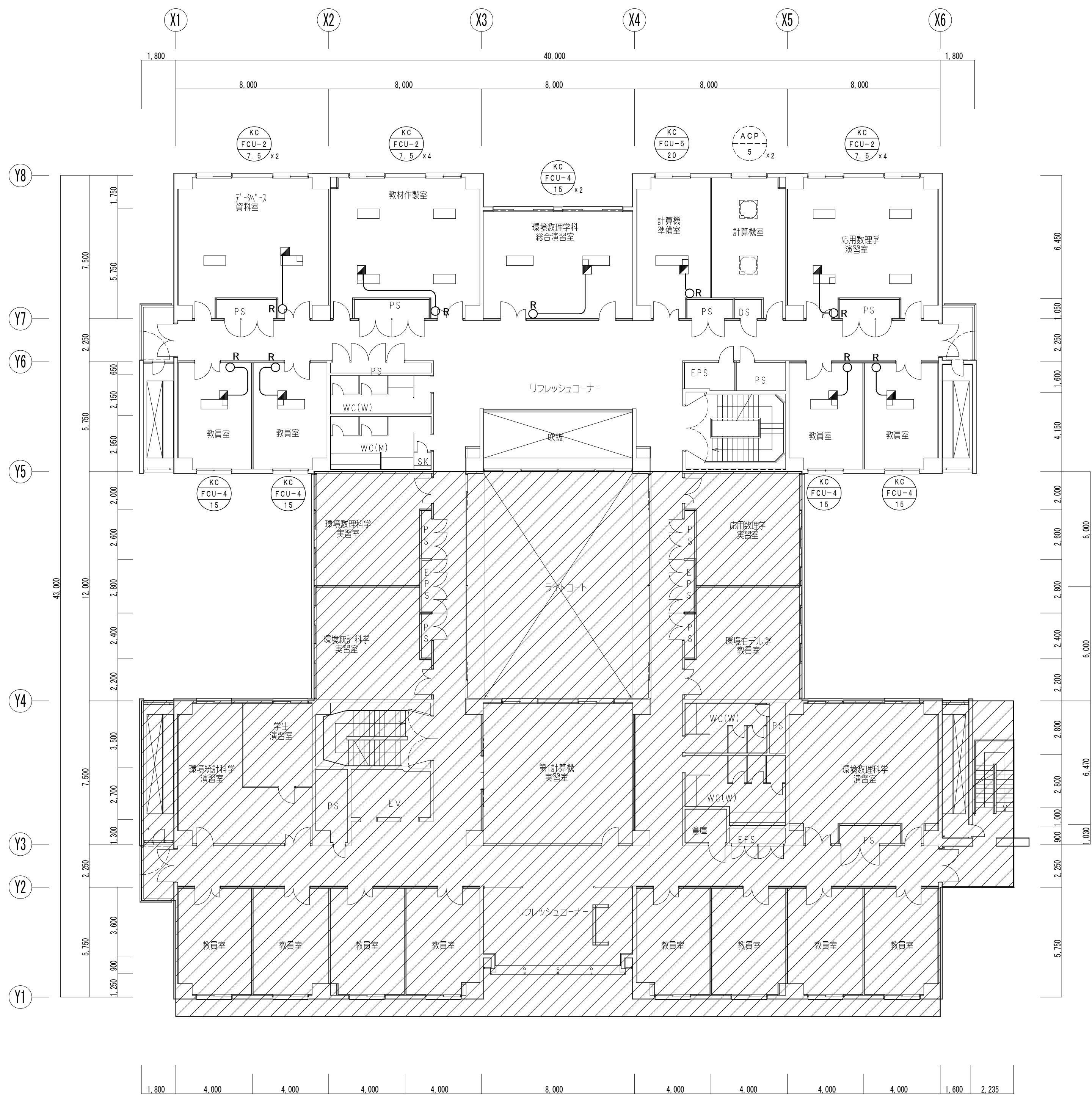
6階平面図 (改修前) 1/150
