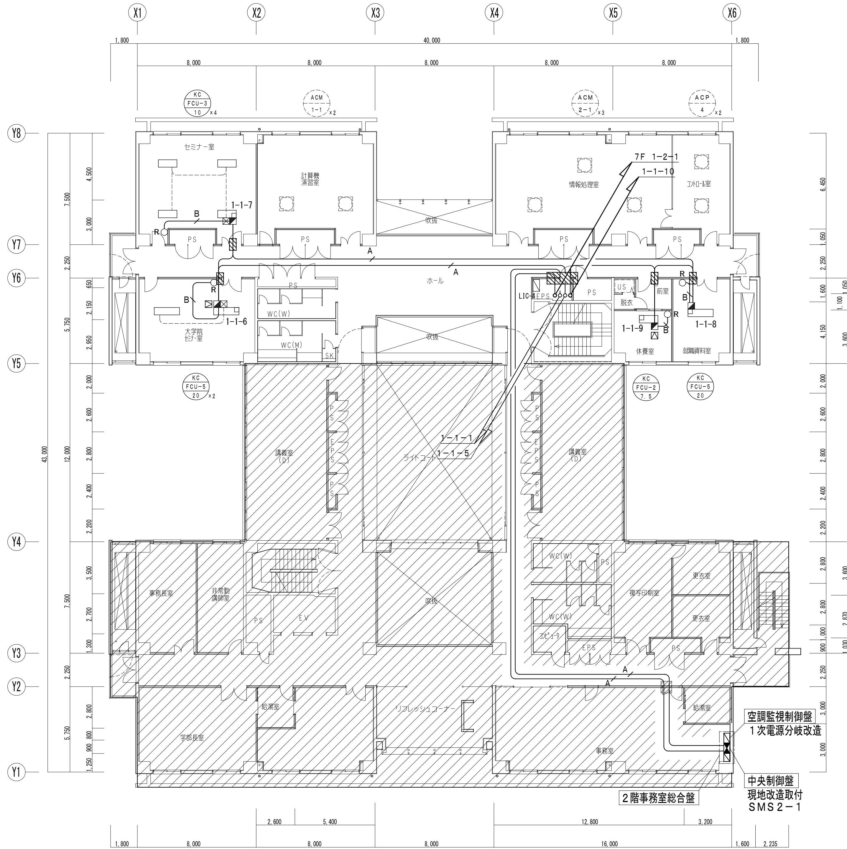
2階平面図 (改修後) 1/150
