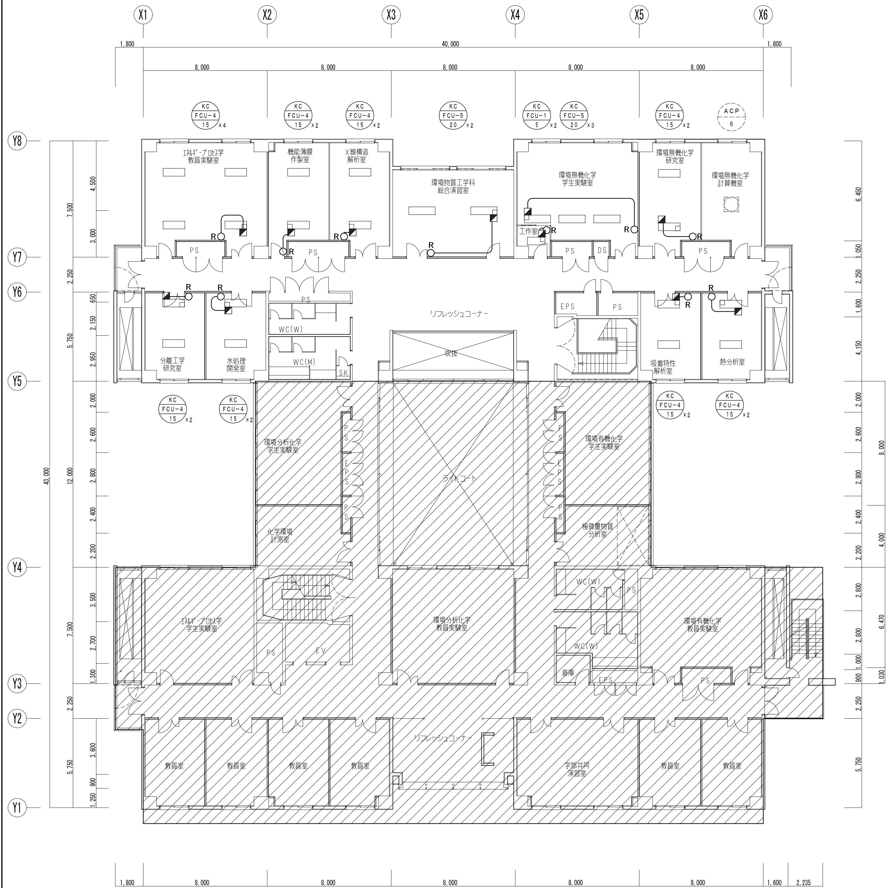
8階平面図 (改修前) 1/150
