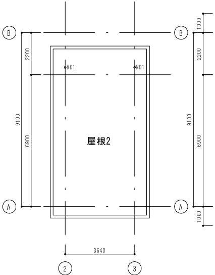
R階(PH)平面図(改修前)
