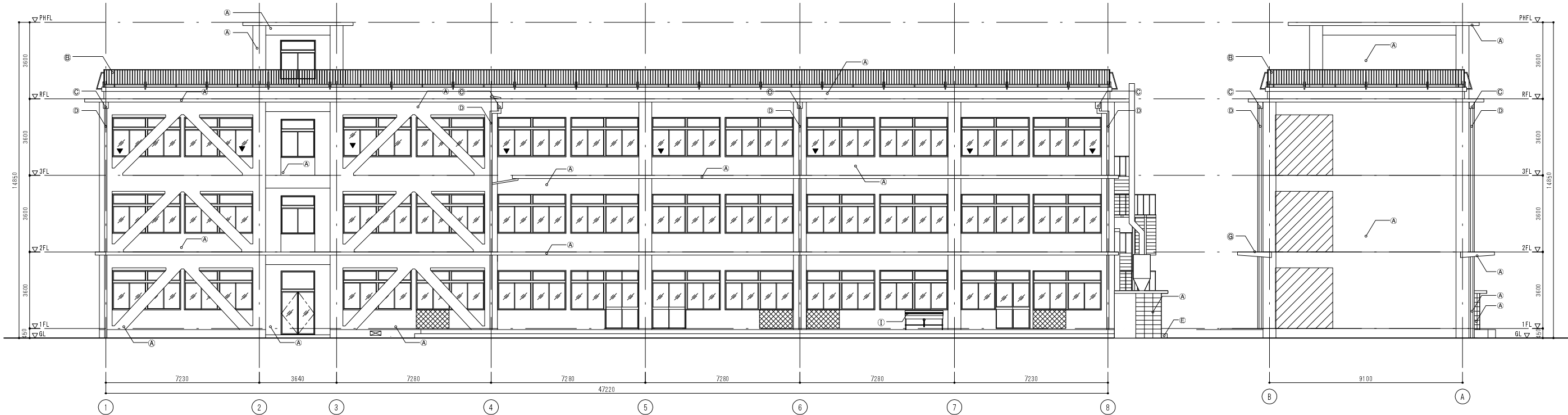
南面立面図
