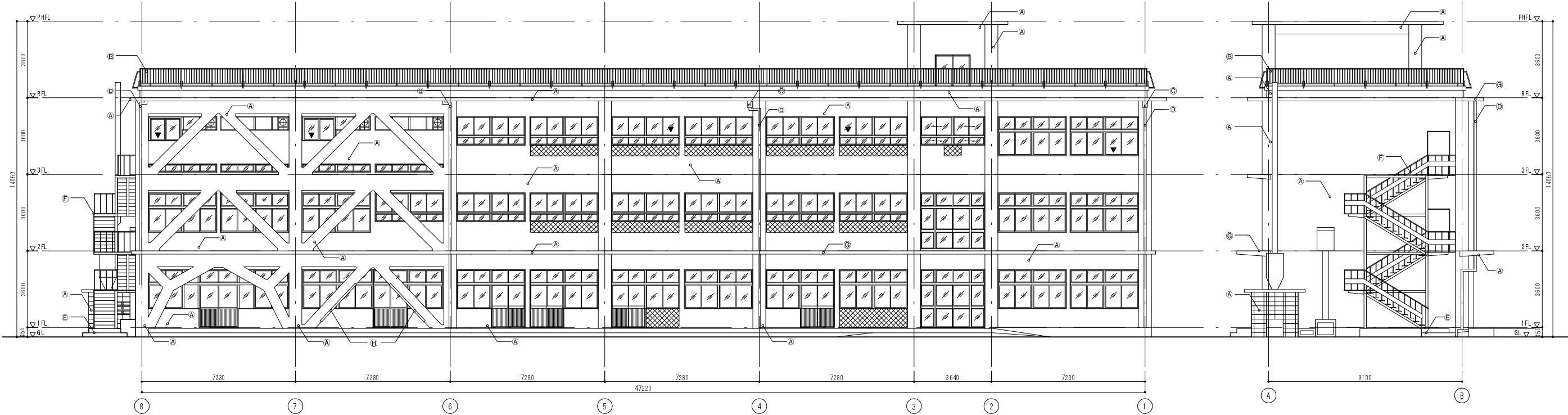
北面立面図
