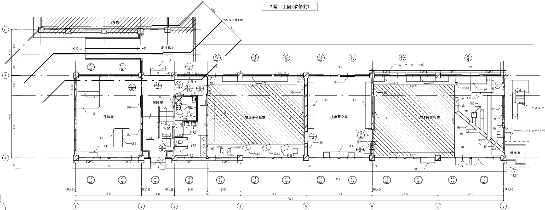
1階平面図 (改修前)
