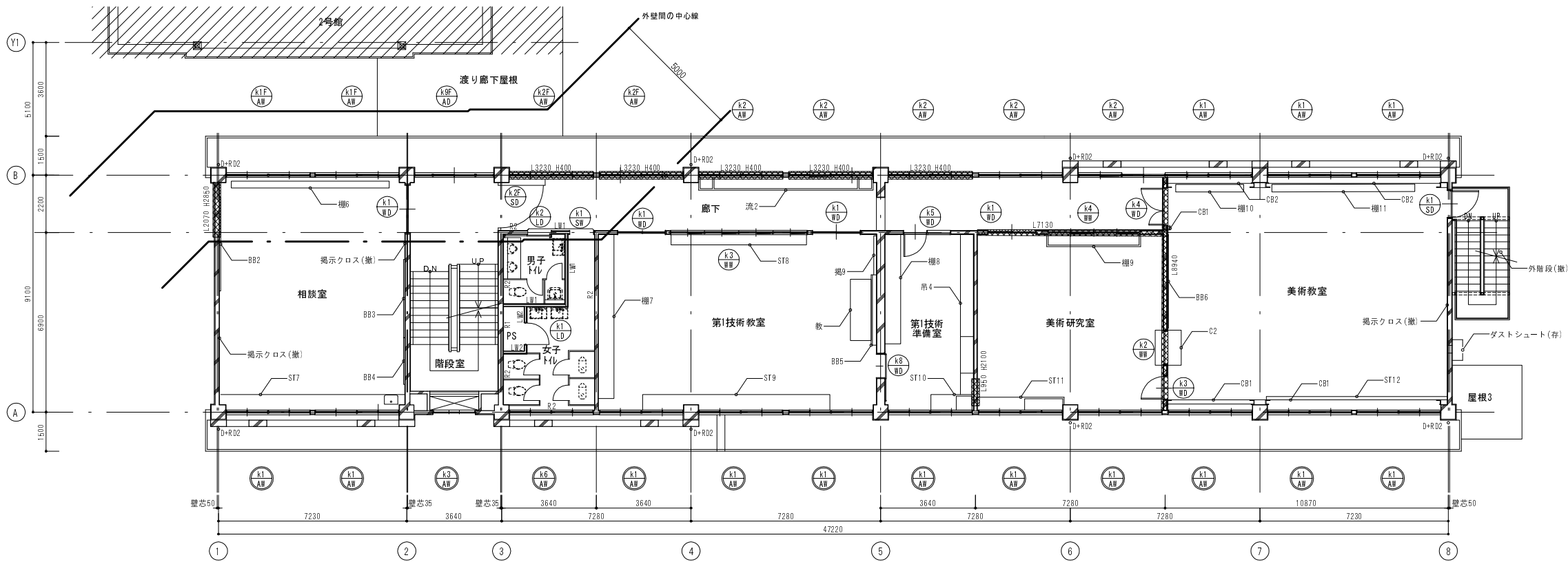
2階平面図 (改修前)
