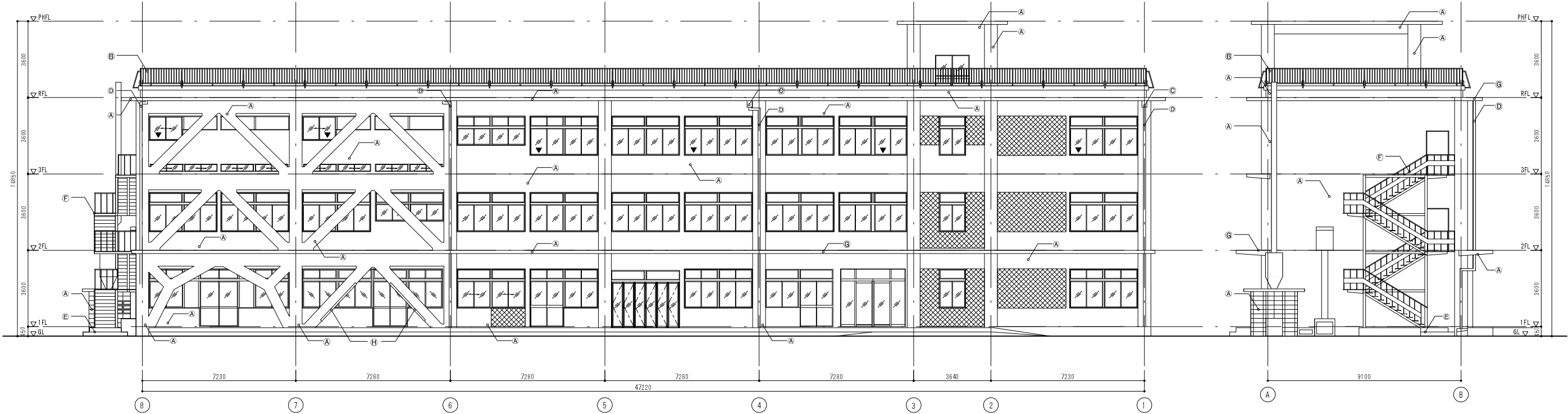
北面立面図
