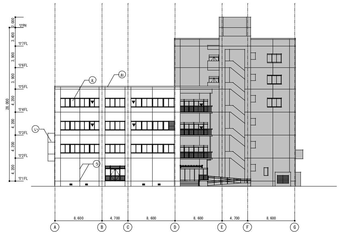
東立面図
