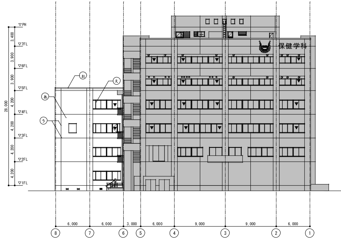
北立面図
