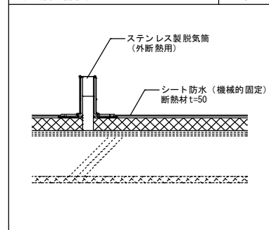
脱気筒 詳細図 S=1/10
