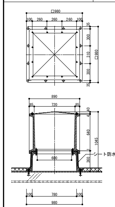
設備用基礎詳細図 S=1/10
