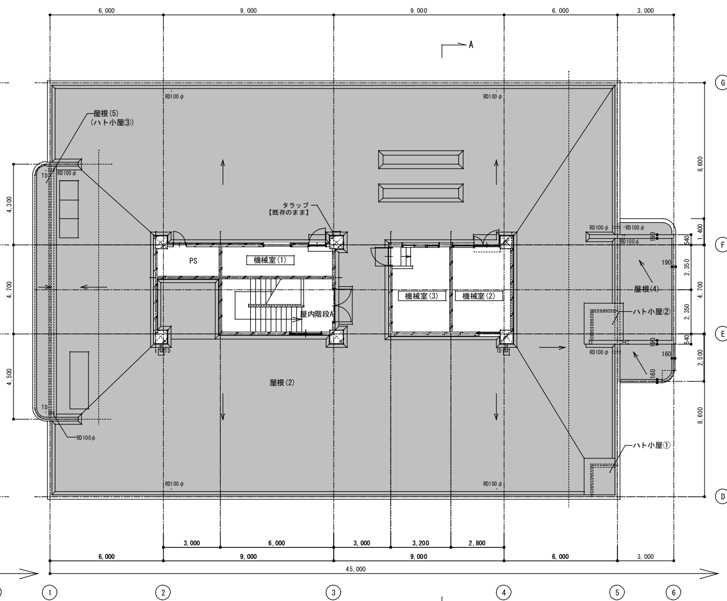
7階 平面図 S=1/100
