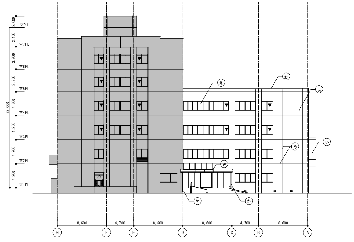
西立面図
