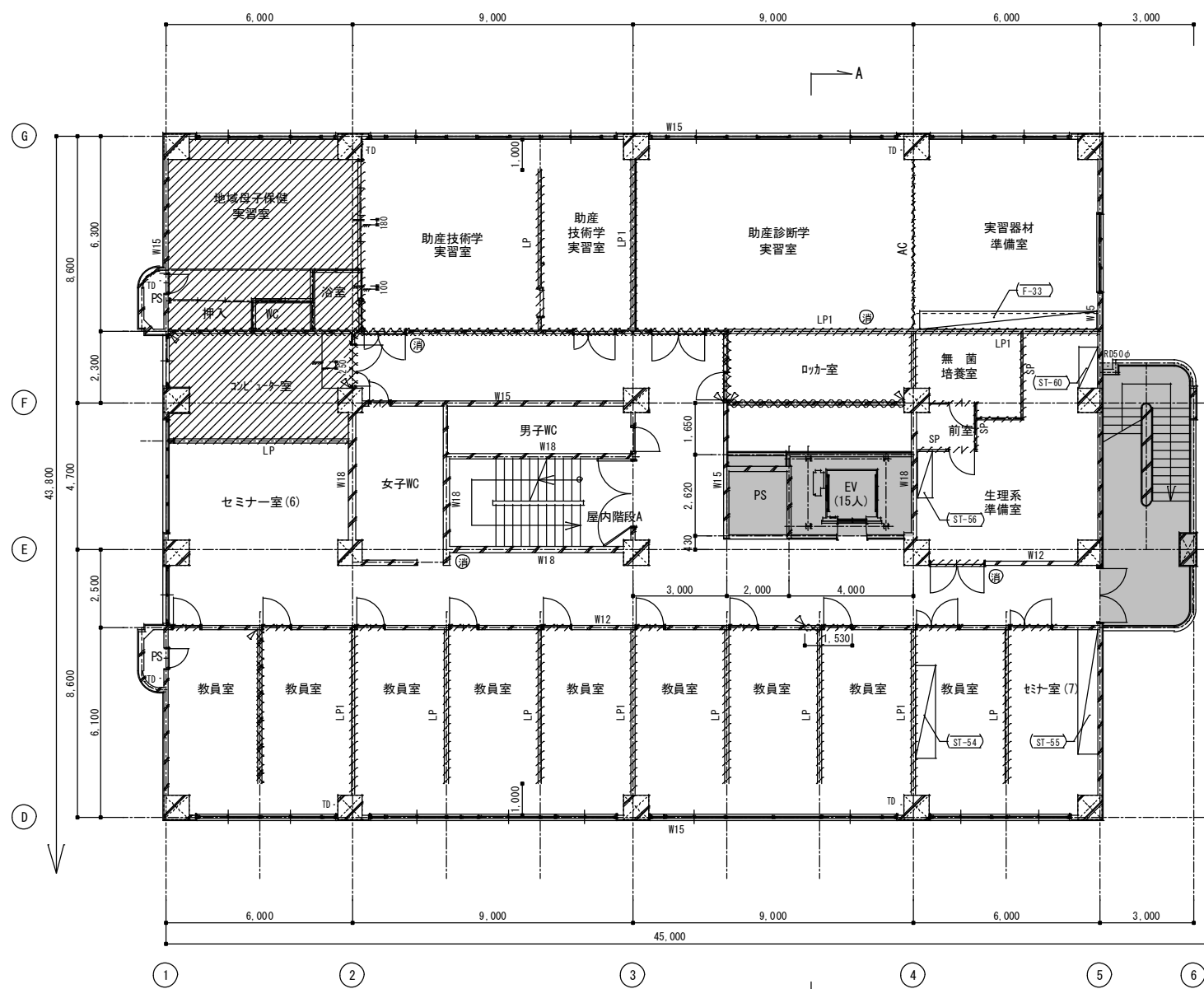
6階 平面図 S=1/100
