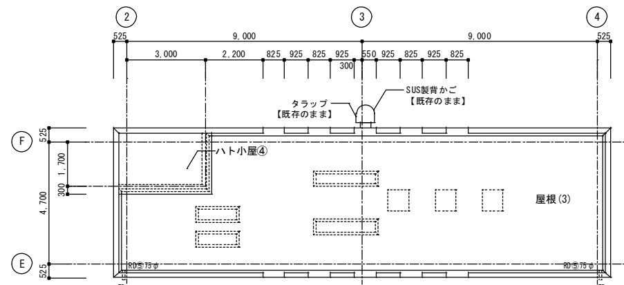
室外機置場 平面図 S=1/100
