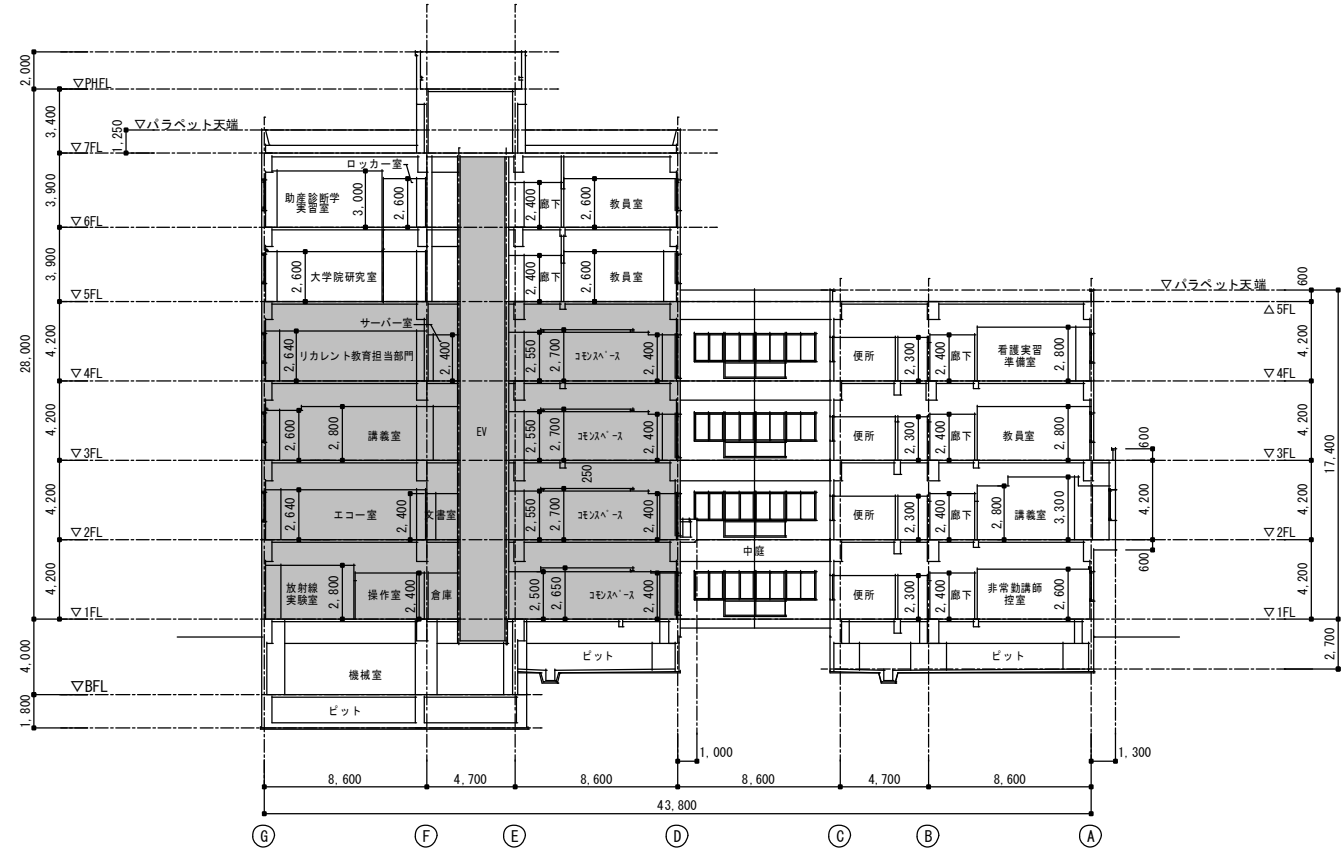
A-A 断面図 S=1/200
