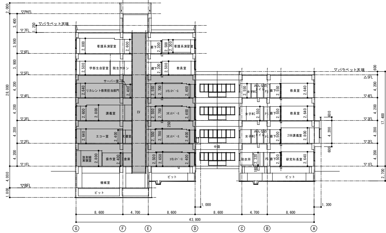
A-A 断面図 S=1/200
