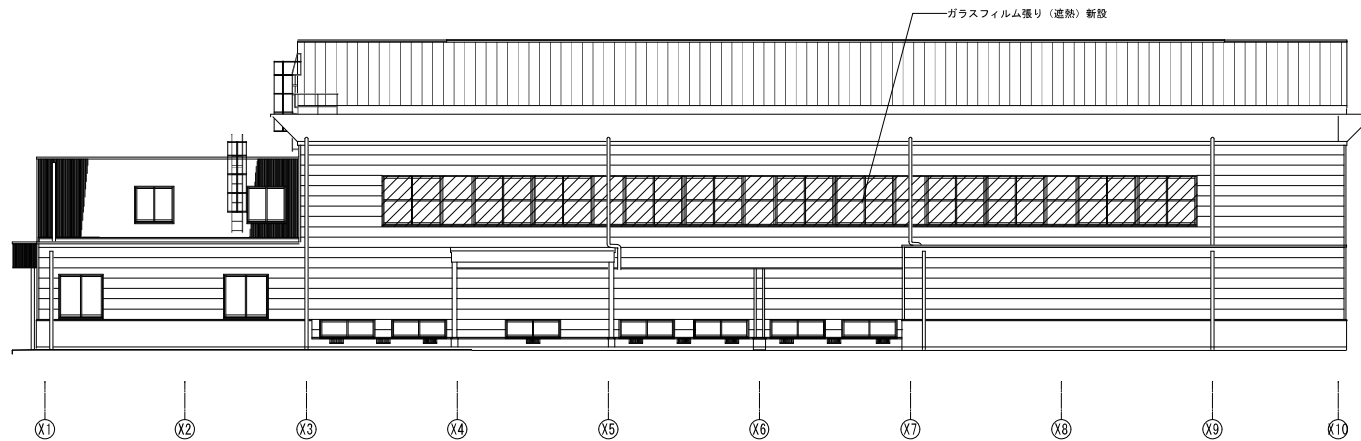
南立面図 1/100
