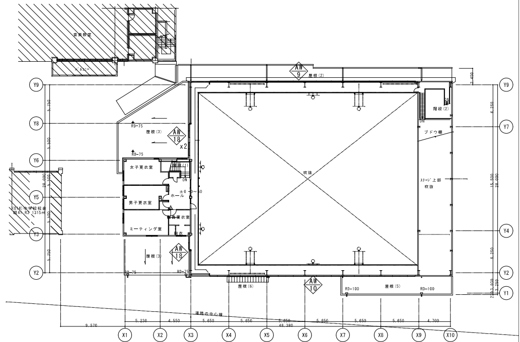
1階平面図 1:200
