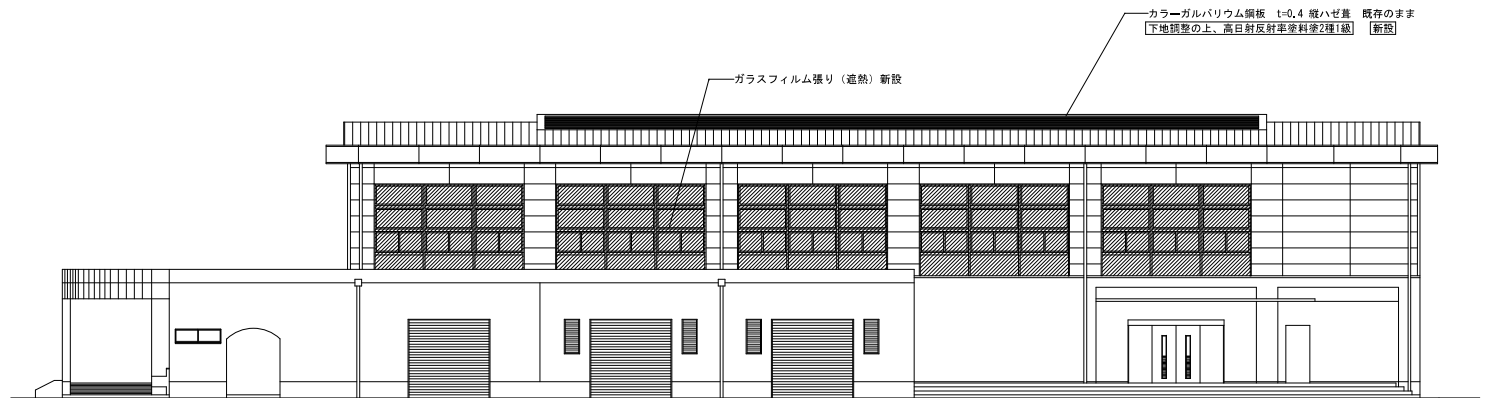
東面立面図 1:100
