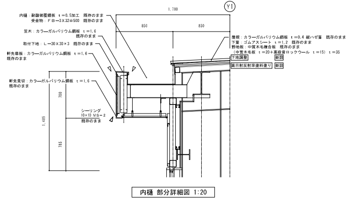
内種 部分詳細図 1:20
