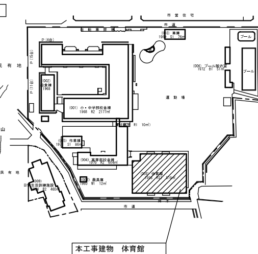
岡山大学平井団地配置図
