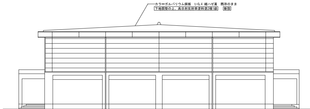
北面立面図 1:100
