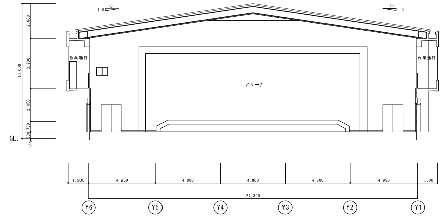
D-D' 断面図 1/100
