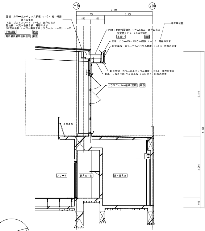
A-A' 矩計図 1:50
