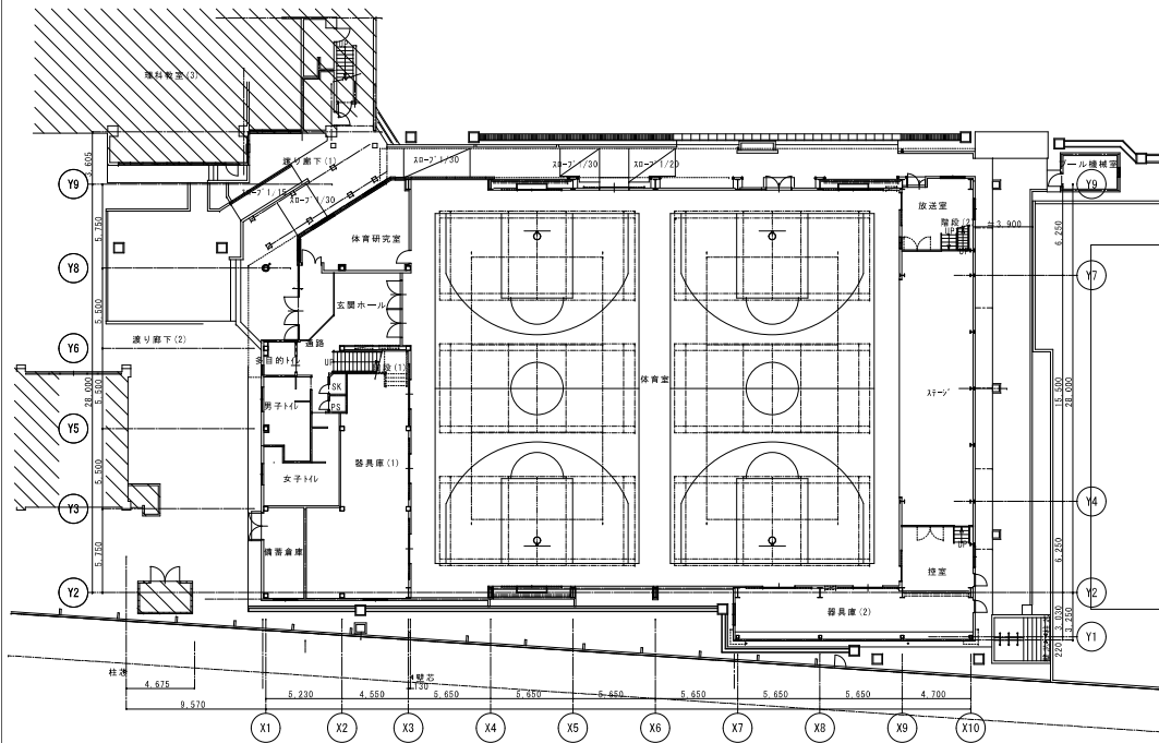
1階屋根伏図・2階平面図 1:200
