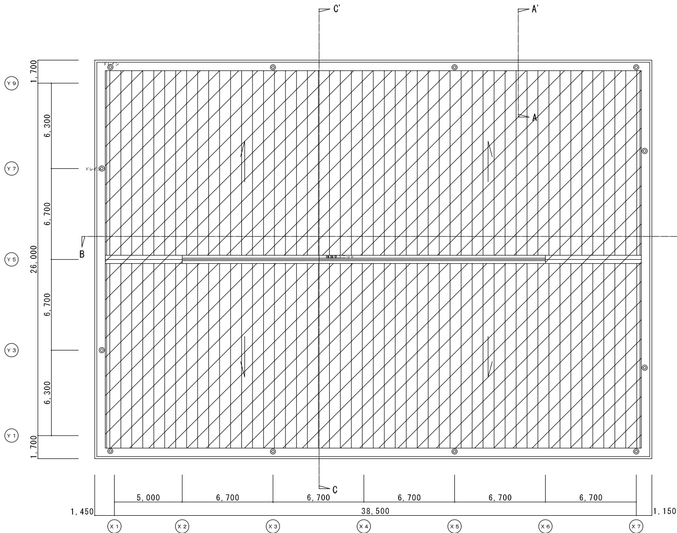
屋根伏図 1:100
