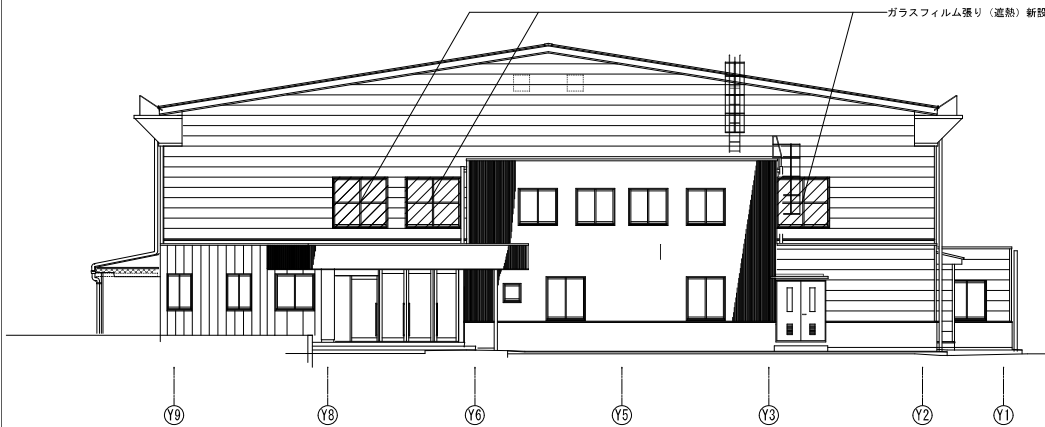
西立面図 1/100
