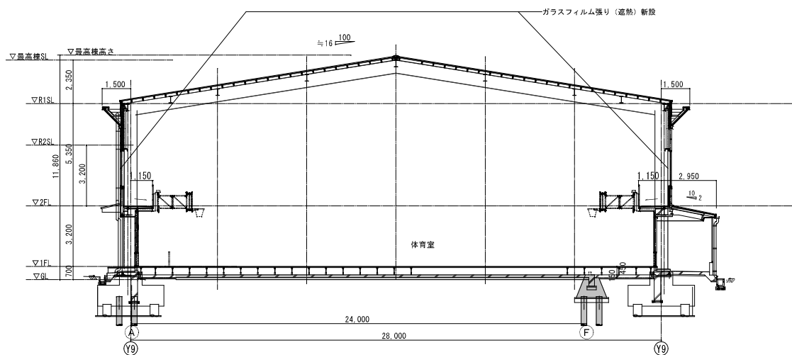
A-A断面図 1/100
