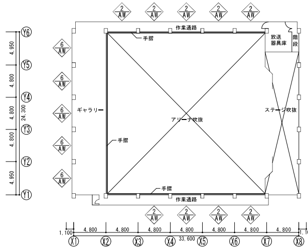
2階 平面図 1/200
