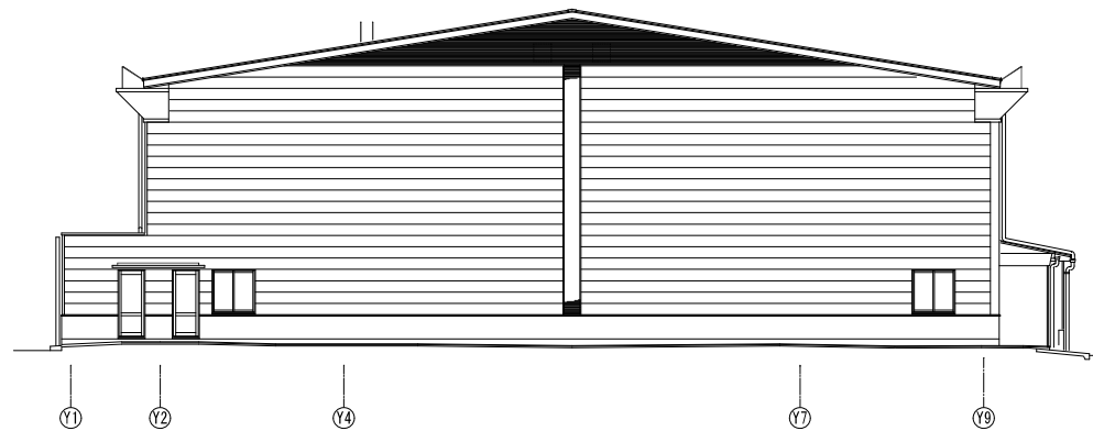
東立面図 1/100
