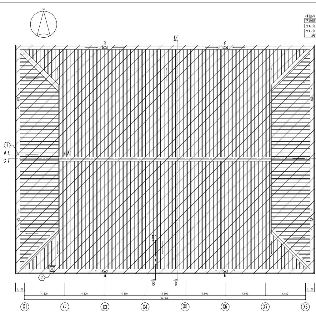
屋根伏図 1/100
