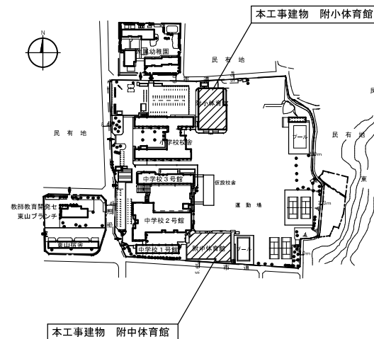
岡山大学東山（一）団地配置図
