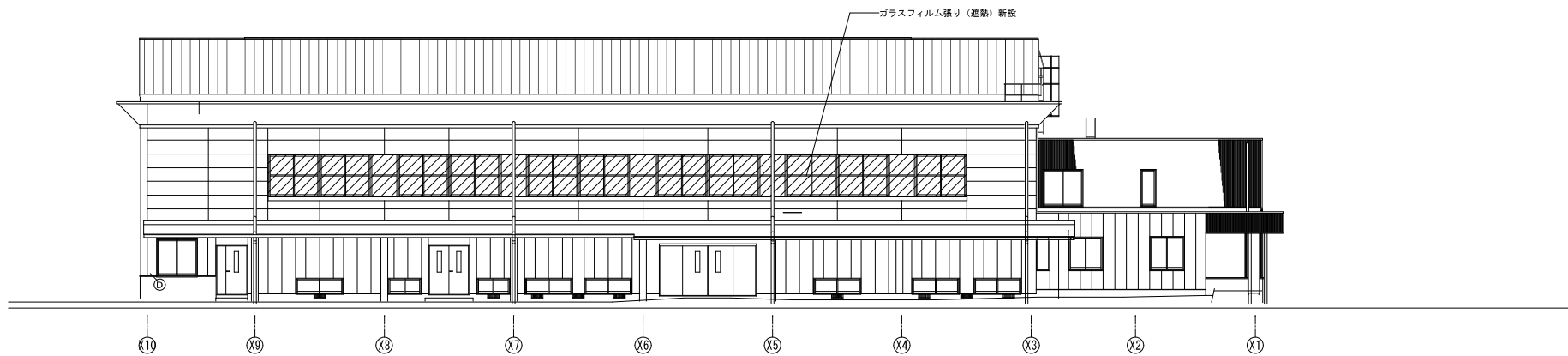
北立面図 1/100
