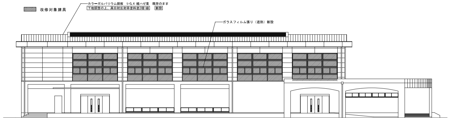
西面立面図 1:100
