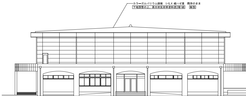
南面立面図 1:100
