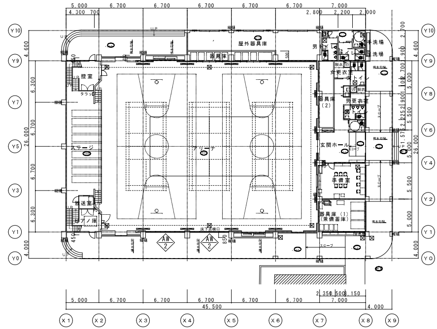
1階平面図 1:200
