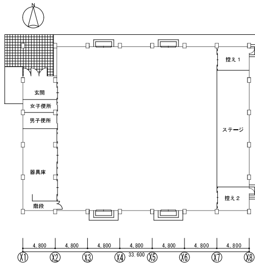
1階 平面図 1/200
