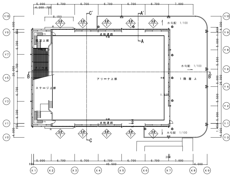
1階屋根伏図・2階平面図 1:200
