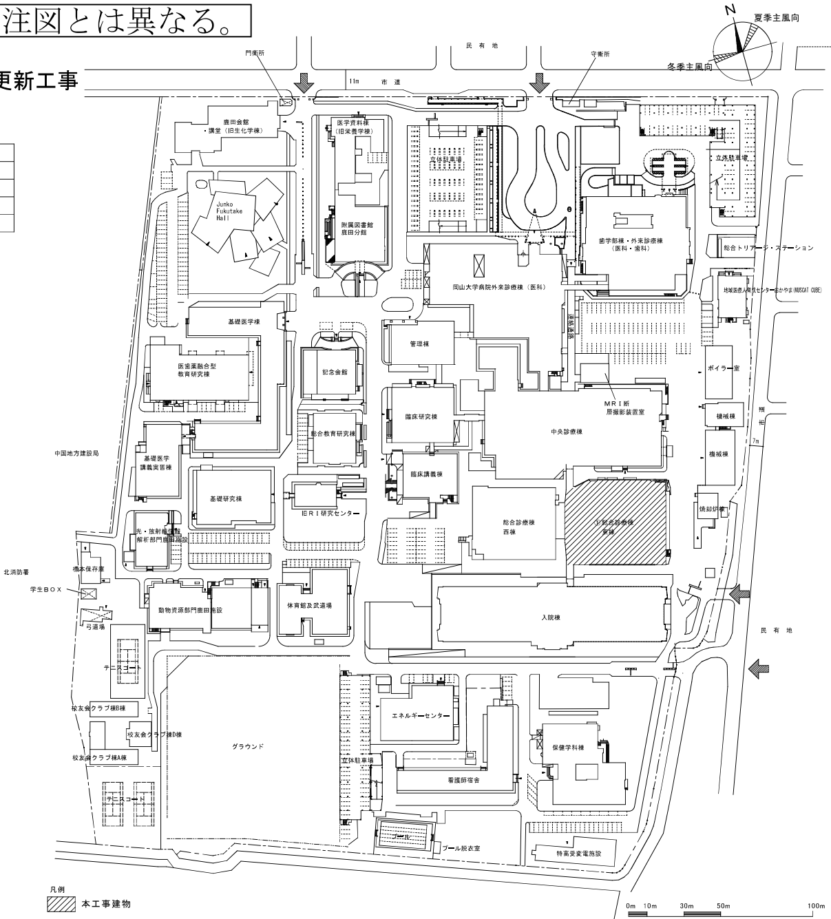
配置図 S=1/1000
