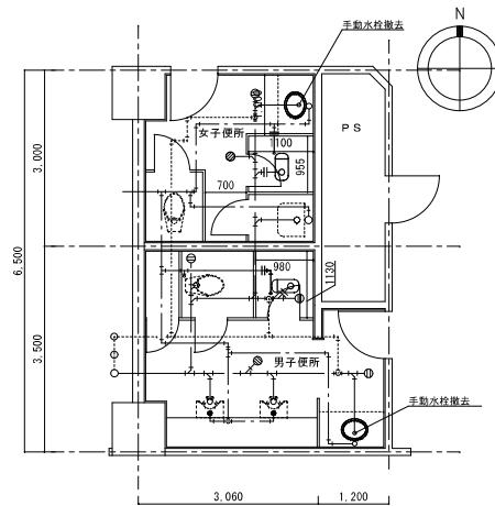
2～6階 トイレ平面詳細図 (改修前) S=1/50 ※細線は既設、太線は撤去を示す。
