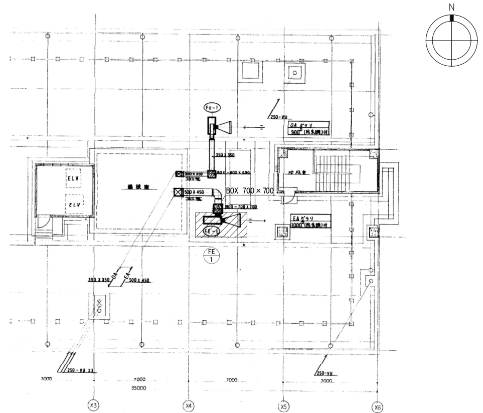
換気設備 屋上階平面図（改修前・後）S=1/100
