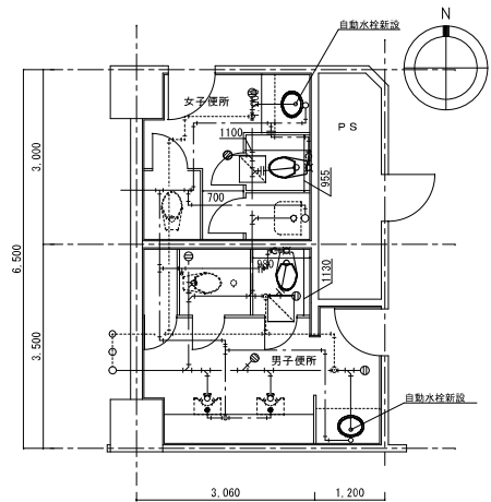
2～6階 トイレ平面詳細図 (改修後) S=1/50 ※細線は既設、太線は新設を示す。
