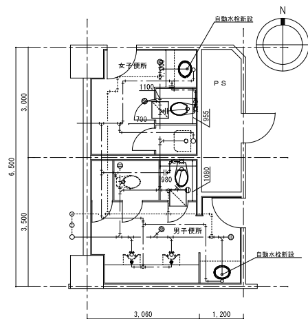
7、8階 トイレ平面詳細図 (改修後) S=1/50 ※細線は既設、太線は新設を示す。
