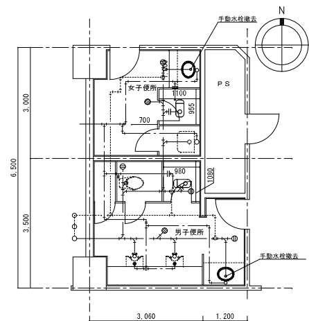
7、8階 トイレ平面詳細図 (改修前) S=1/50 ※細線は既設、太線は撤去を示す。
