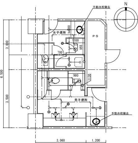
1階 トイレ平面詳細図 (改修前) S=1/50 ※細線は既設、太線は撤去を示す。
