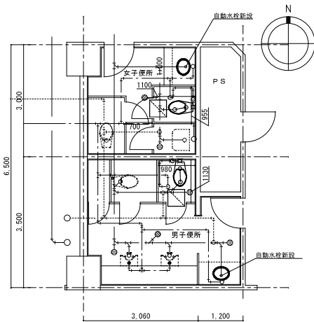
1階 トイレ平面詳細図 (改修後) S=1/50 ※細線は既設、太線は新設を示す。
