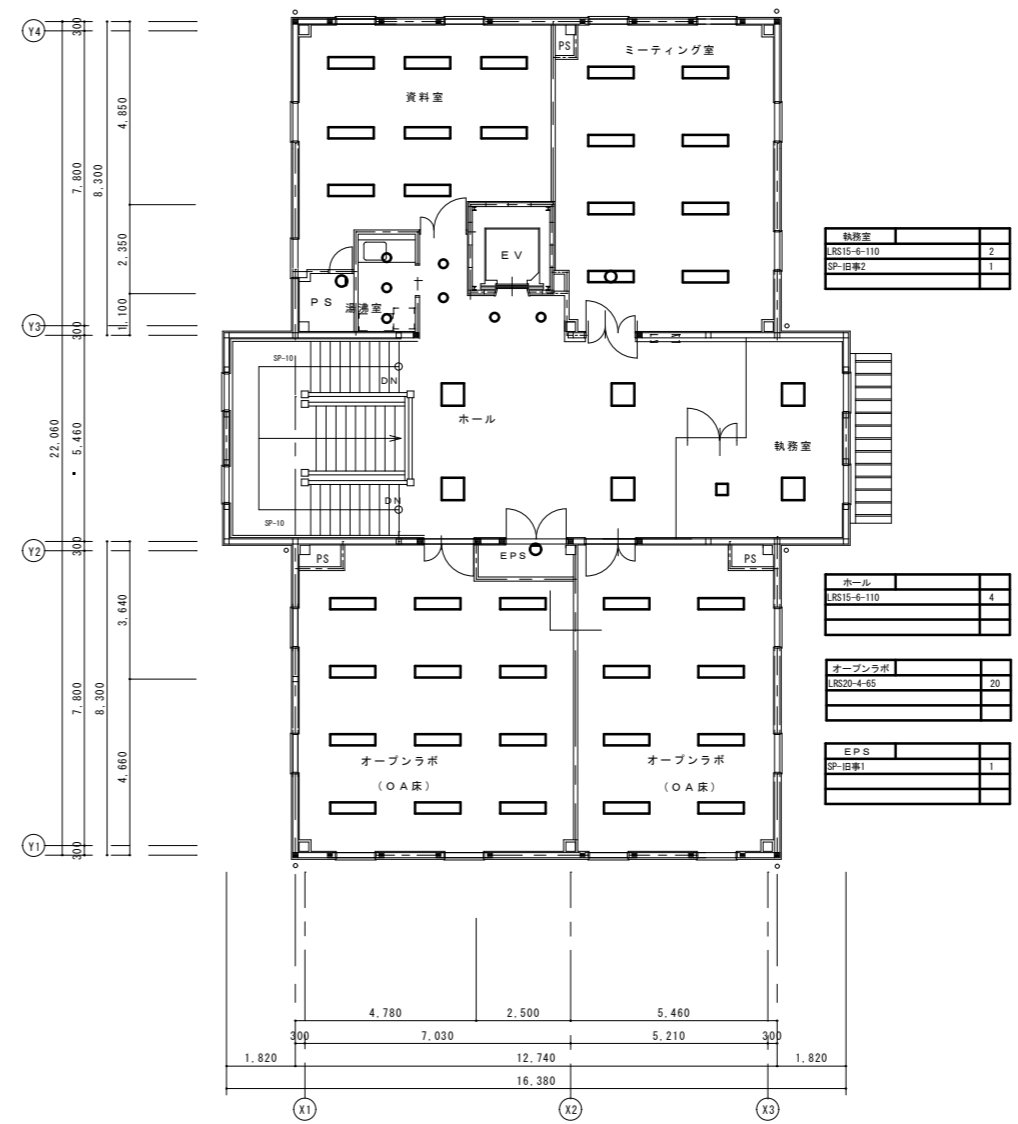
2階 平面図 1/100
