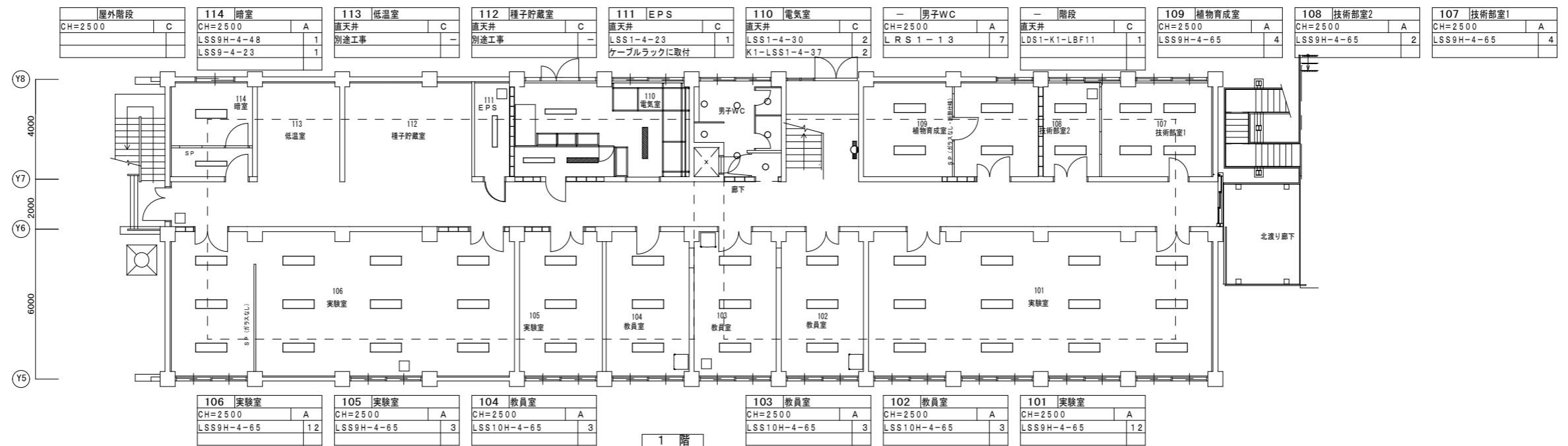
研究棟2号館電灯分岐改修配線図 S=1/100
