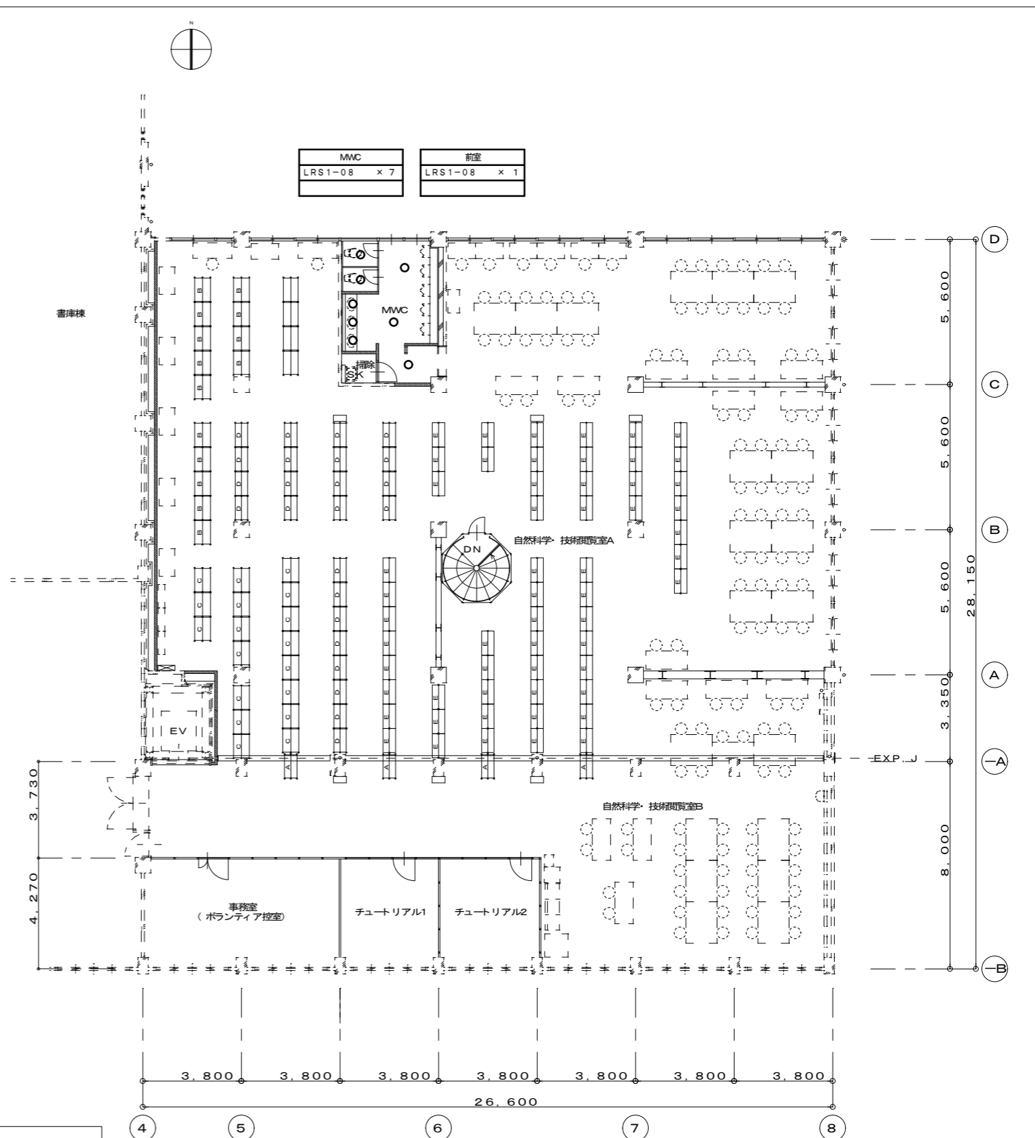
2階平面図 S=1/100
