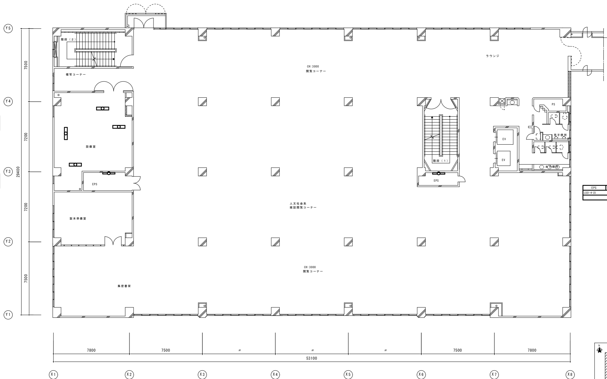
2 階 平面図 1 : 100
