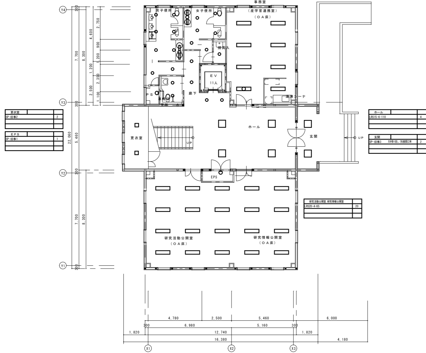
1階 平面図 1/100
