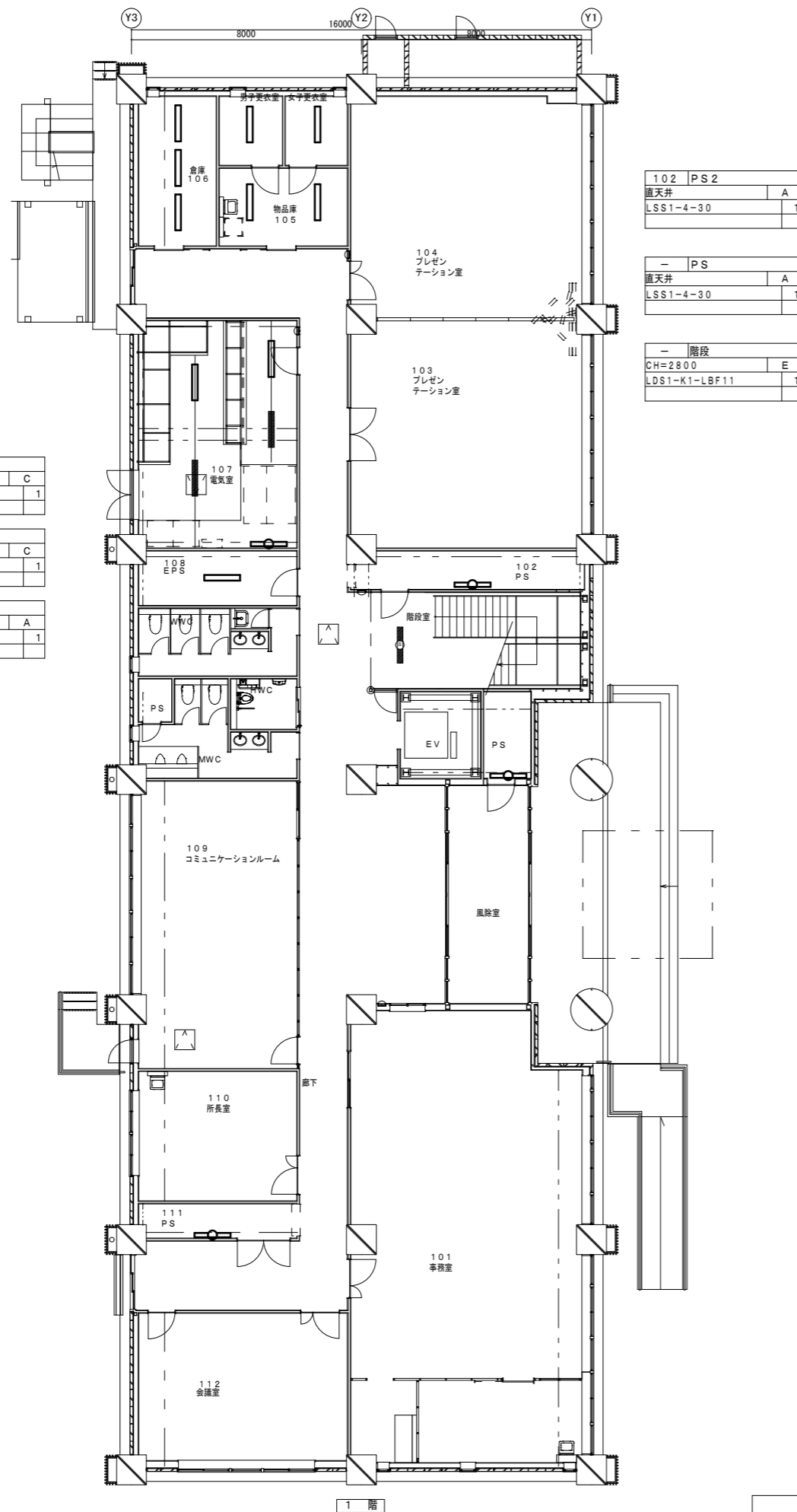
電灯分岐配線図 S=1/100
