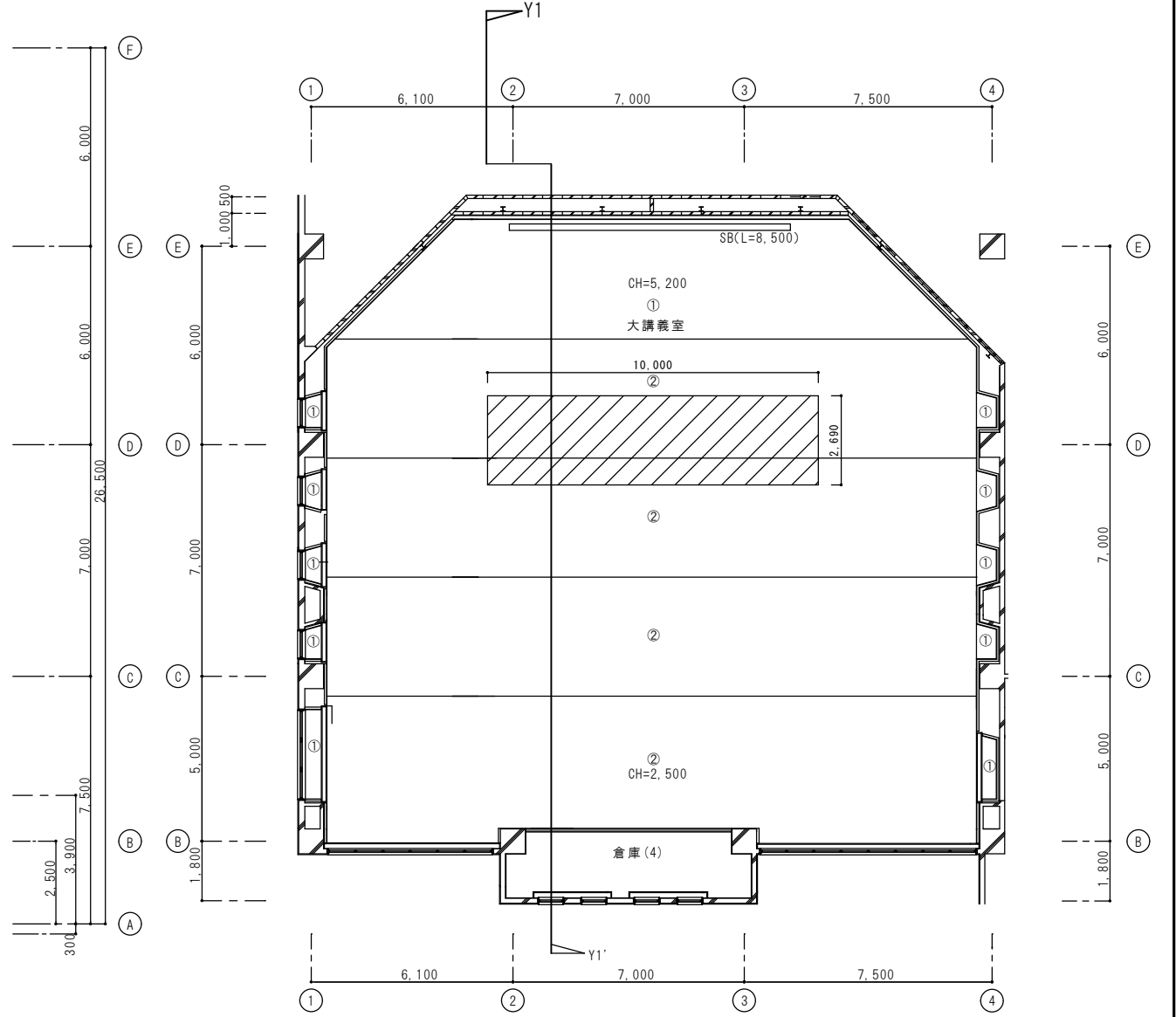
3階天井伏図 S=1/100
