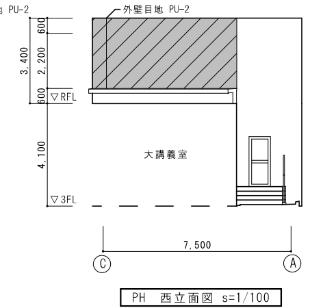
PH 西立面図 s=1/100
