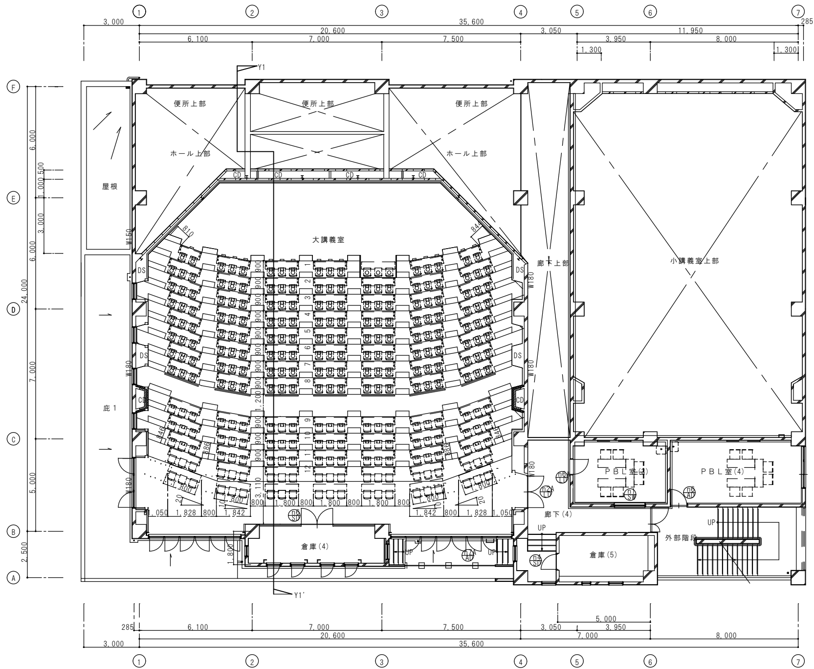
3階平面図 S=1/100 ※参考図面
