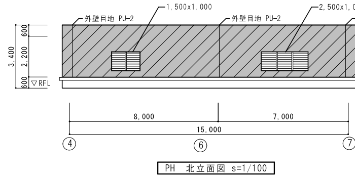
PH 北立面図 s=1/100
