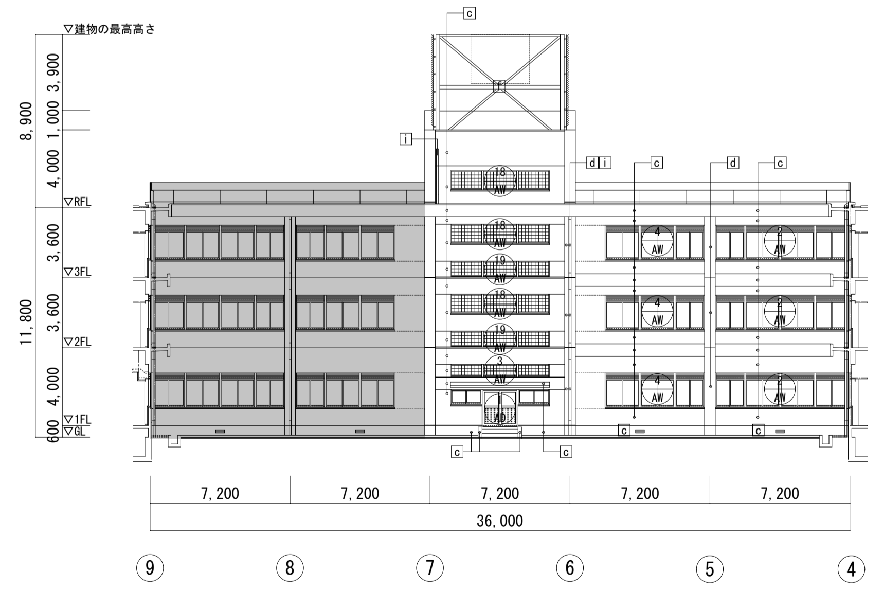
東立面図(D通り) S=1:200
