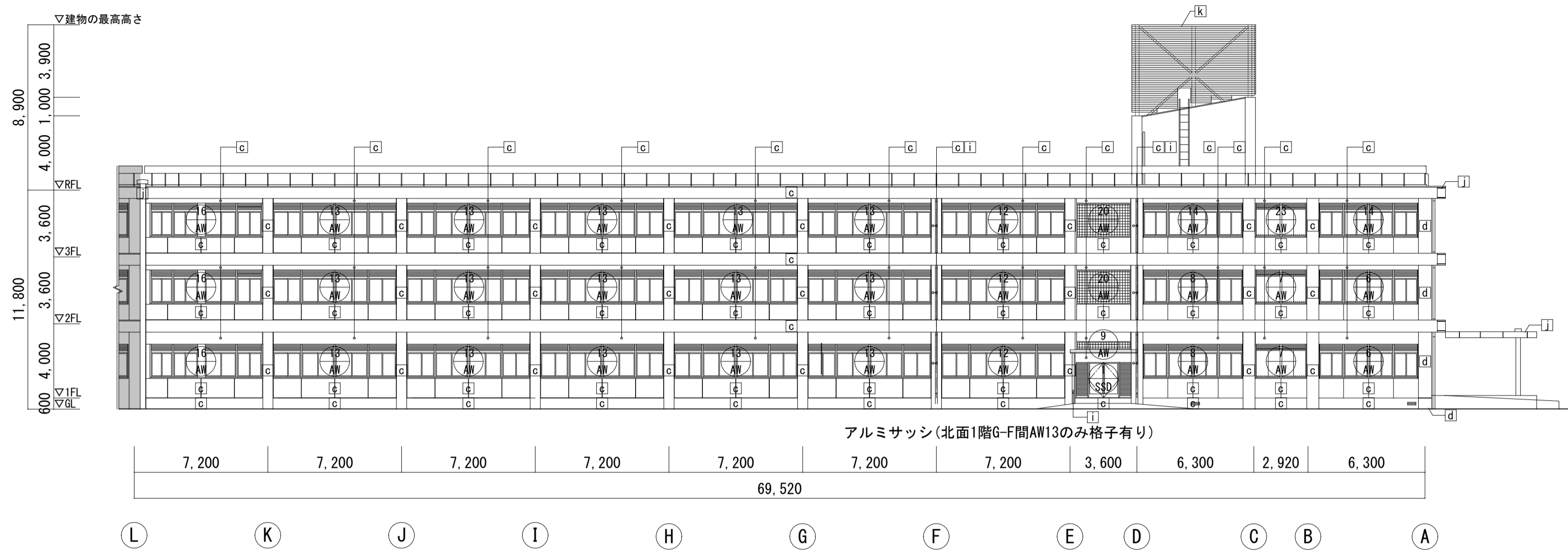
北立面図(1通り)S=1:200
