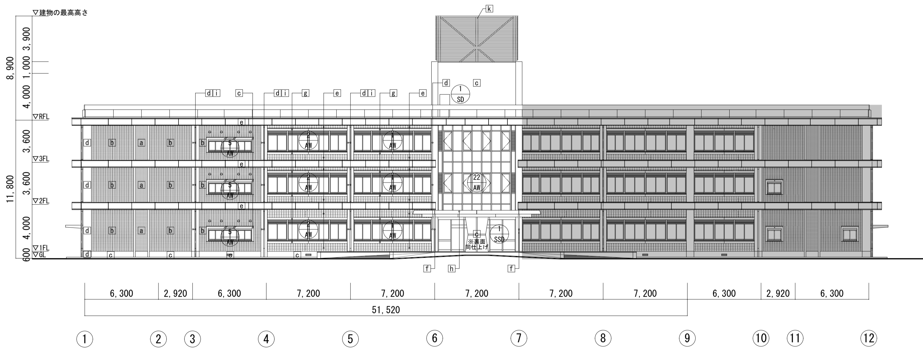
西立面図S=1:200
