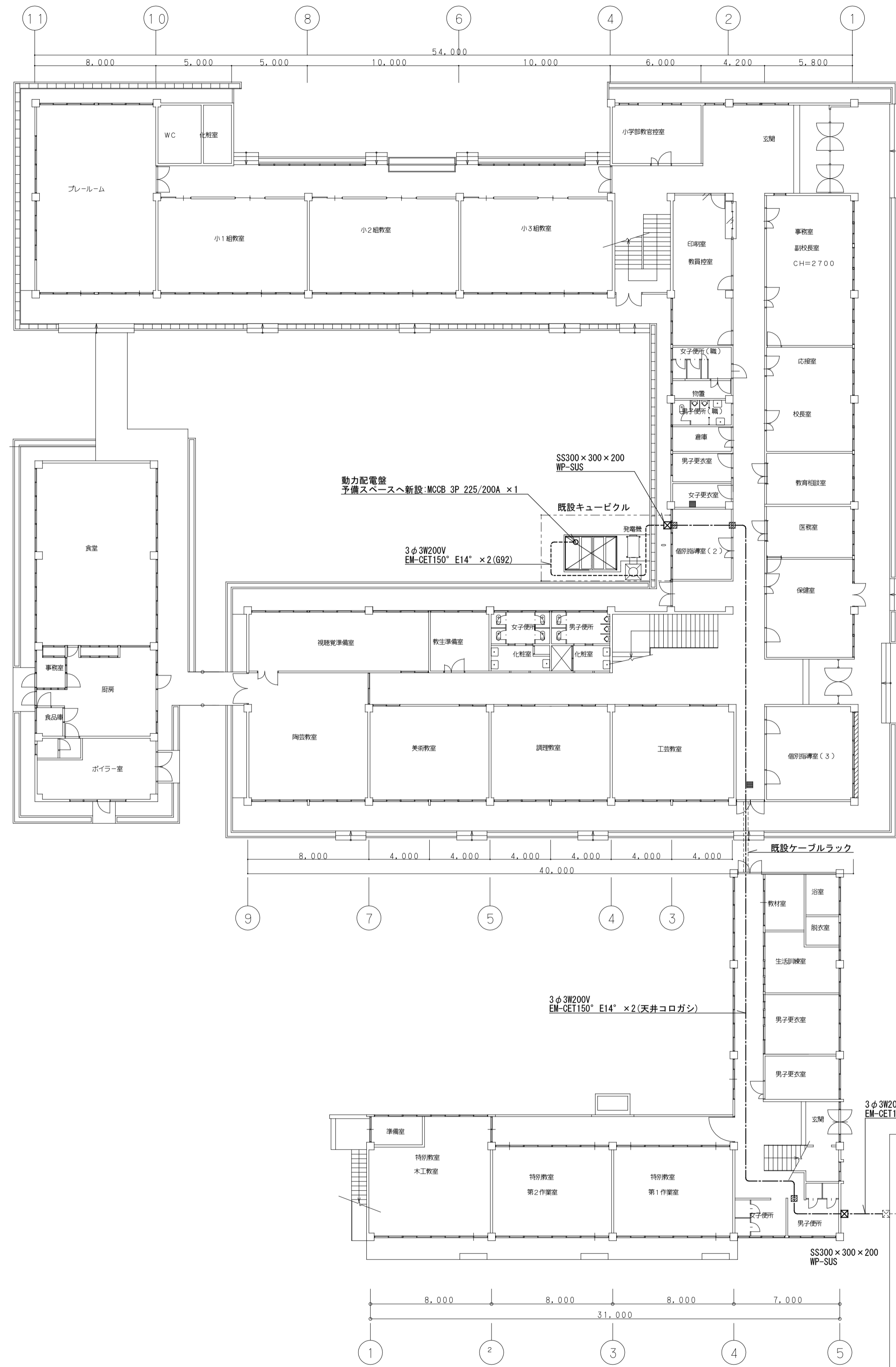
(平井) 体育館 構内配電線路図 S=1/200
