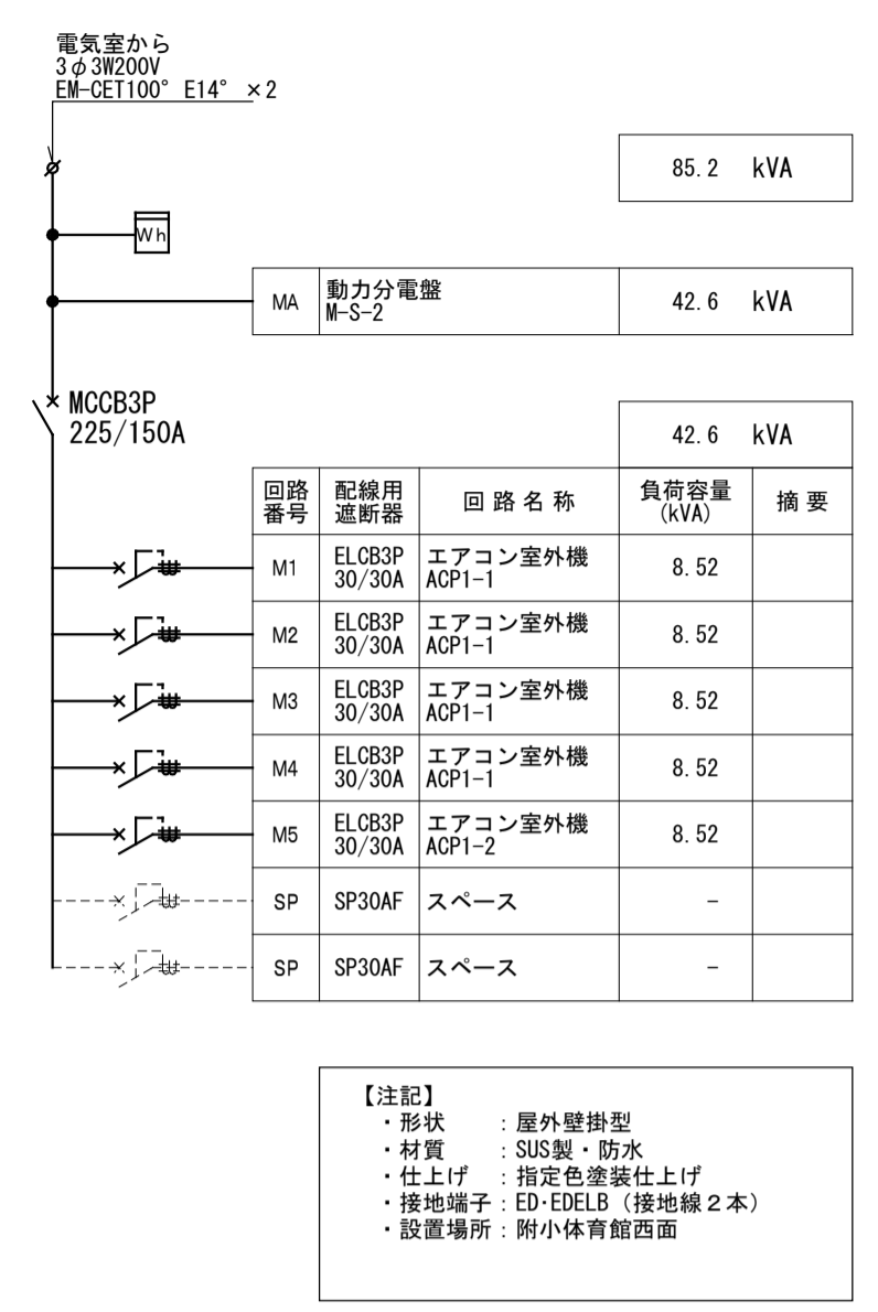
動力分電盤 (M-S-1) 結線図
