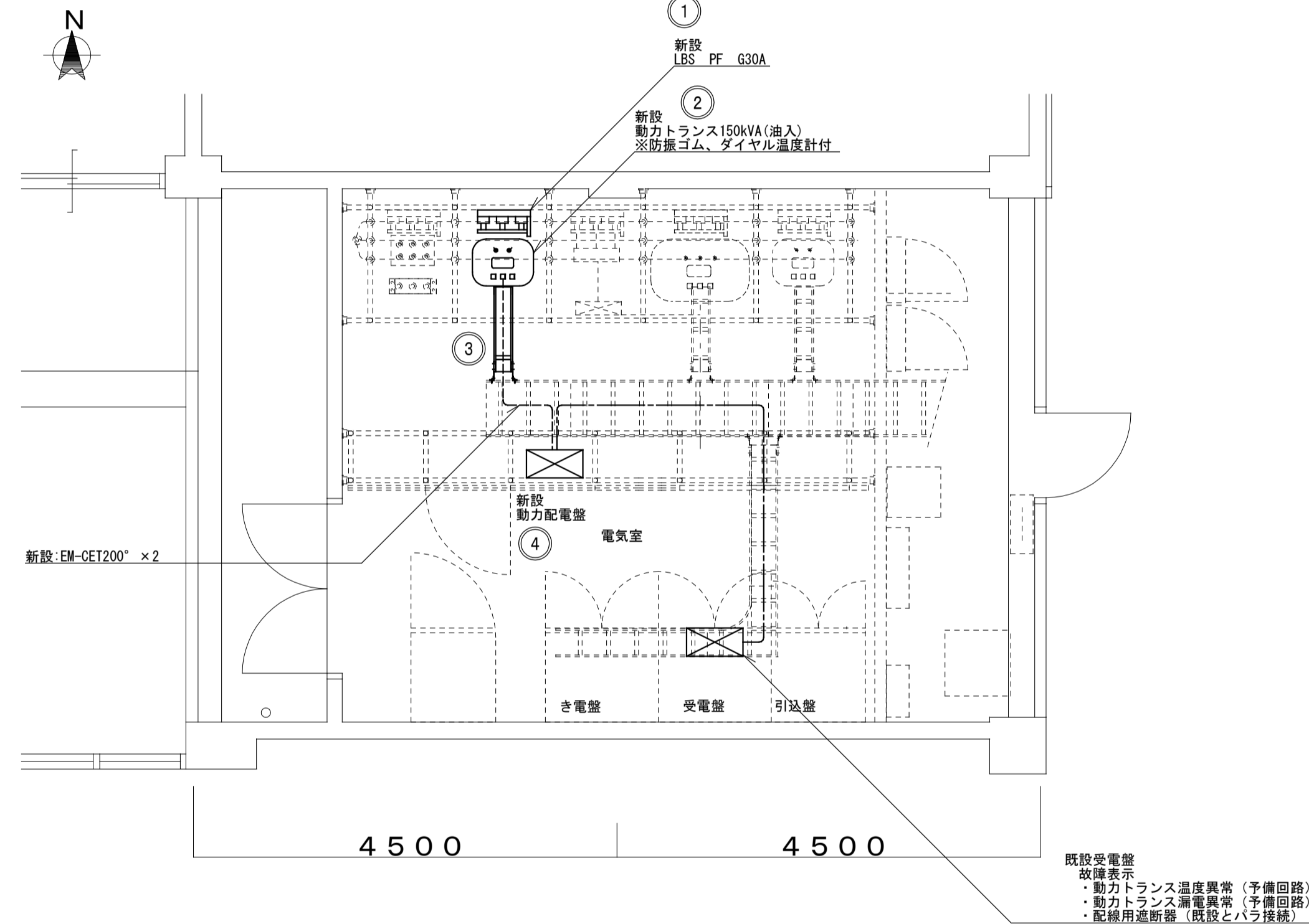
小学校校舎1階電気室 配線図 S=1/50
