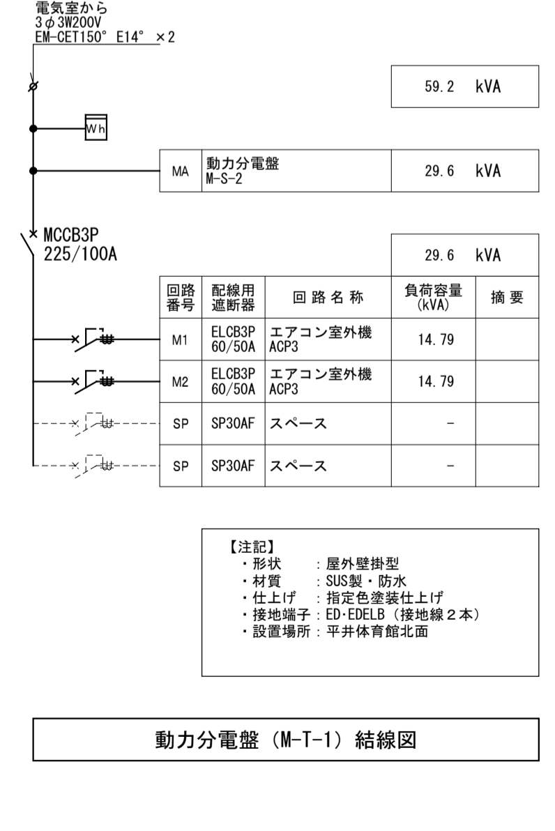
動力分電盤 (M-T-1) 結線図
