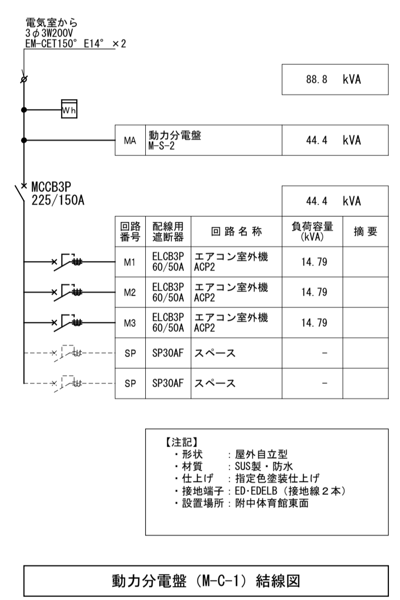
動力分電盤 (M-C-1) 結線図
