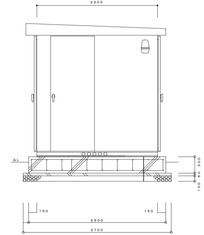
屋外キュービクル姿図
