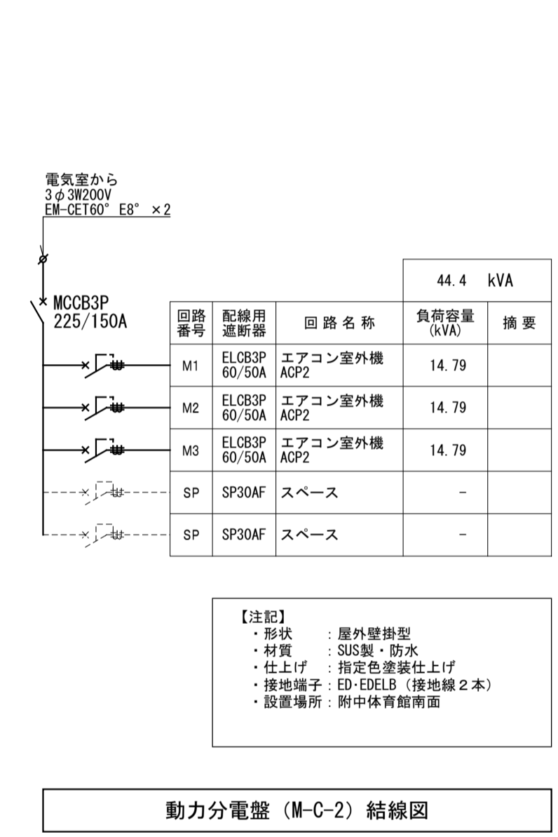
動力分電盤 (M-C-2) 結線図
