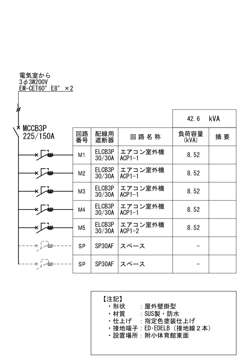
動力分電盤 (M-S-2) 結線図
