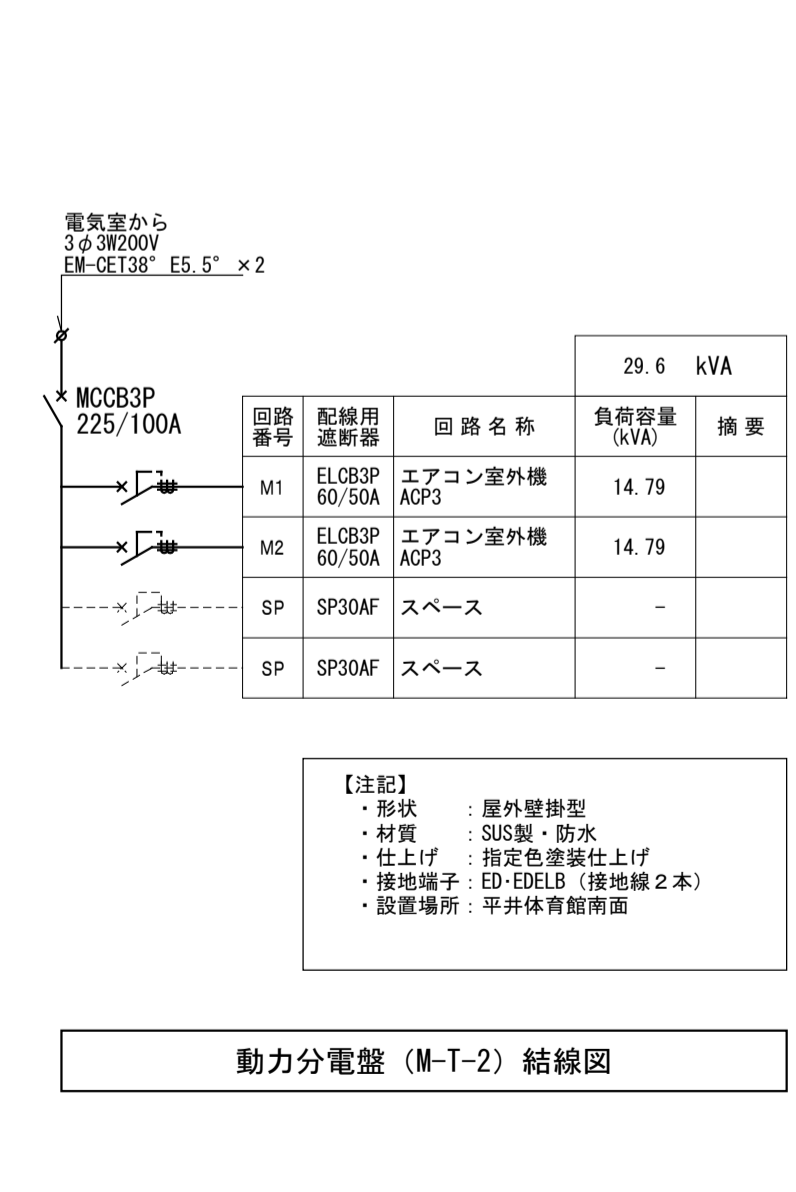
動力分電盤 (M-T-2) 結線図
