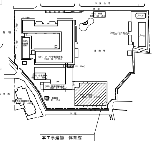
岡山大学平井団地配置図
