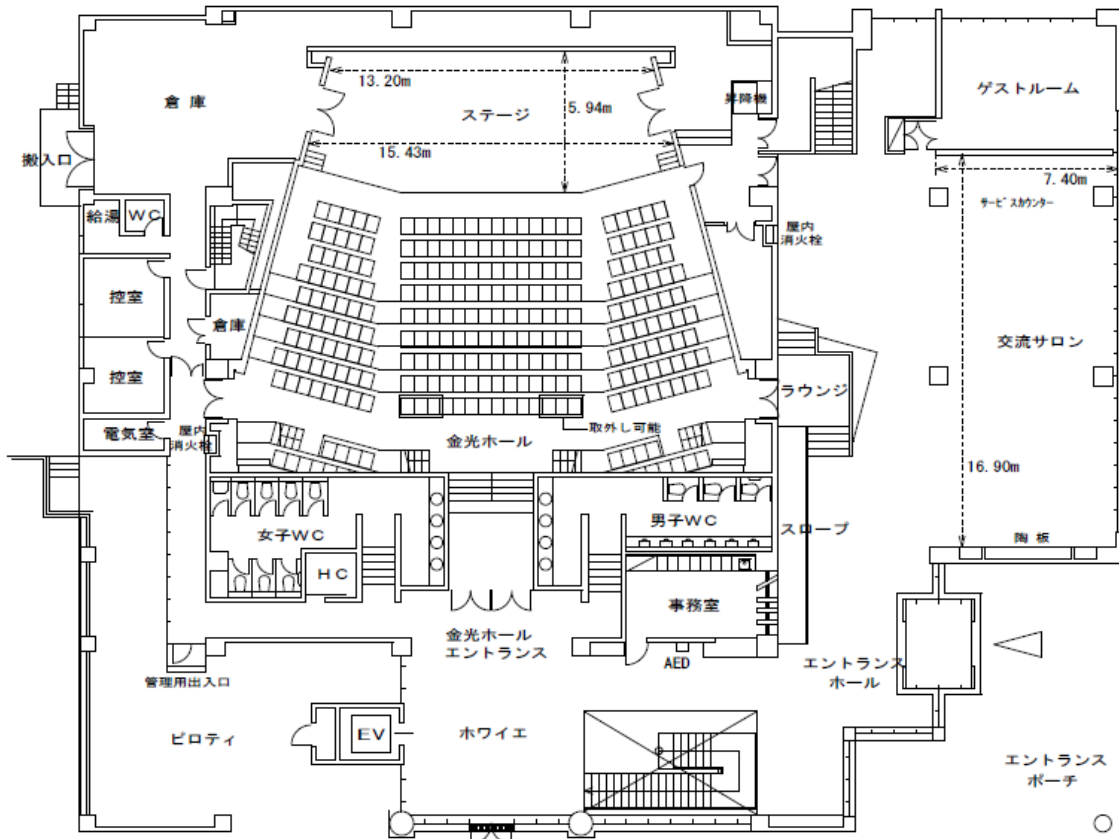
1 F 平面図
