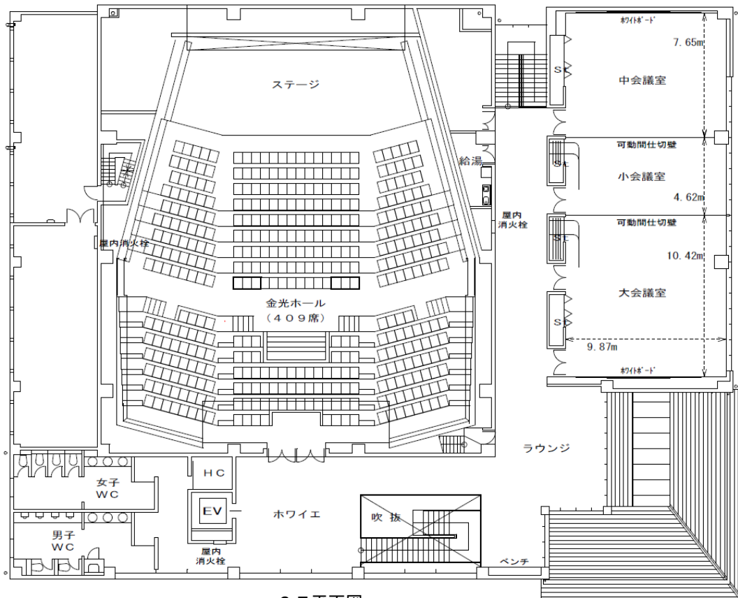
2 F 平面図
