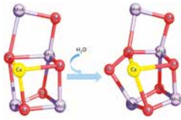
S 1 状態 S 3 状態 Mn 4 CaO 5 クラスターの S 1 - S 3 状態遷移に伴う構造変化 Structural changes of the Mn 4 CaO 5 -cluster during the S 1 -S 3 state transition
