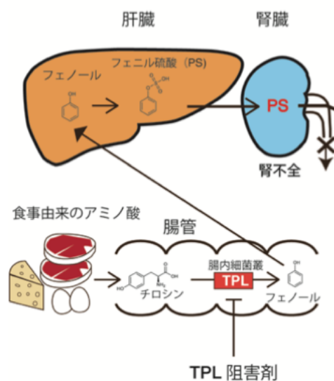
図 1. 食事から摂取するチロシンを原料にフェニル硫酸 (PS) が産生されるまでの経路、および腎臓でのポドサイト障害、TPL 阻害剤の作用点。
