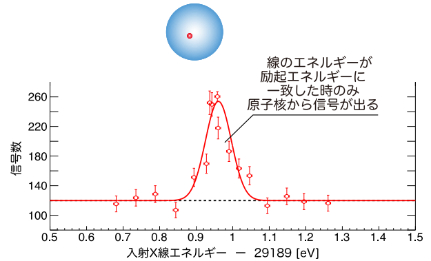
図2 共鳴曲線(原子核共鳴散乱法によるトリウム 229 第二励起状態への遷移を確認)
