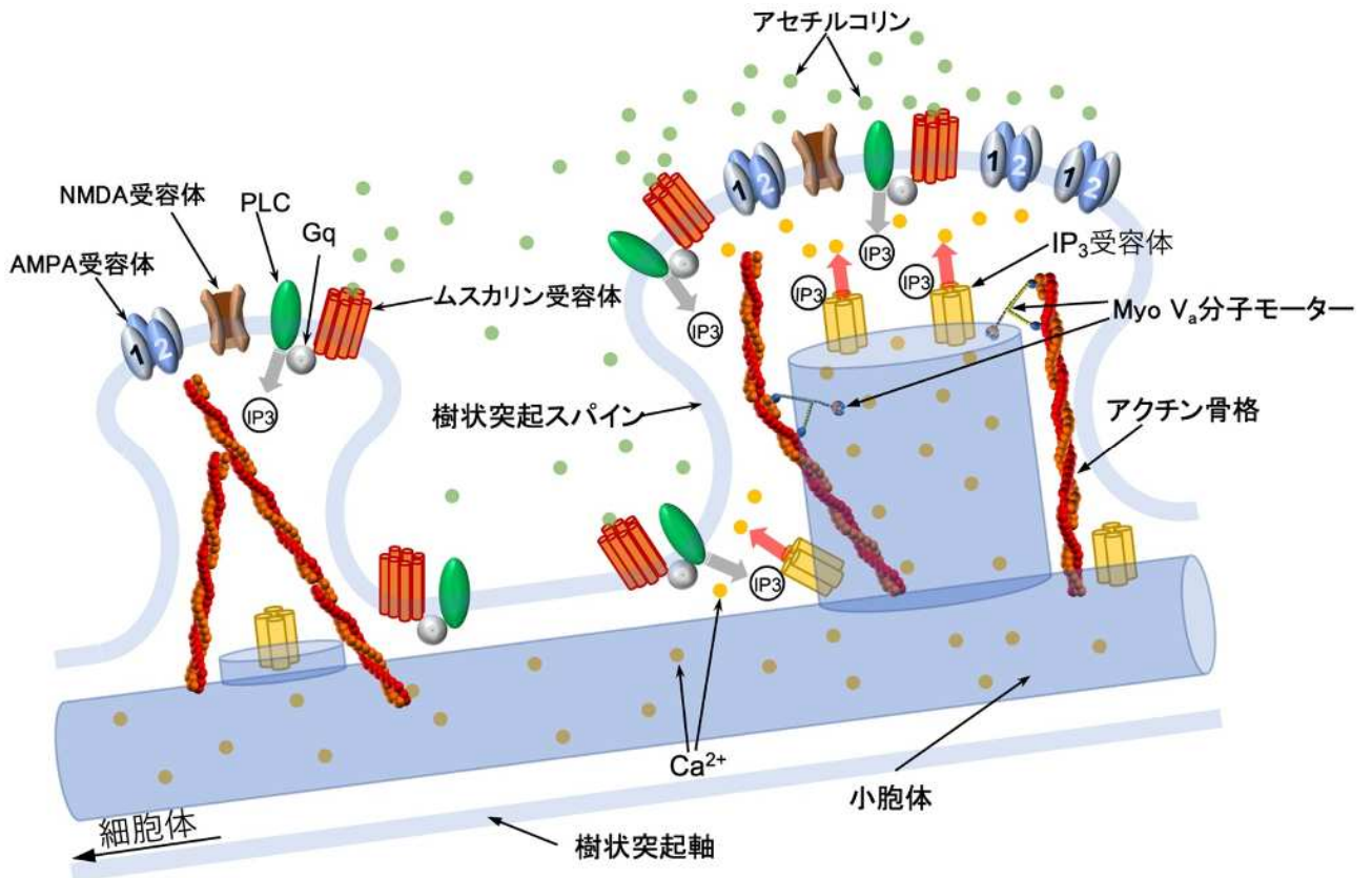
図 1. 海馬興奮性ニューロンの樹状突起スパインにおけるシナプス後膜に存在する神経伝達物質受容体及びシナプス関連分子。細胞体まで繋がっている小胞体を、分子モーターミオシン V o がアクチン骨格上を二足歩行しながら、活性の高い樹状突起スパイン先端まで牽引し、小胞体内 Ca 2+ イオンをスパイン細胞質へ効率的に放出するのをアシストする。
