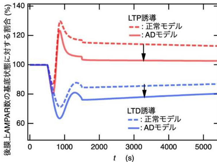
図 3. アルツハイマー(AD)モデルによる LTD 誘導の増強及び LTP 誘導の減弱によるシナプス伝達の低下。AD モデルでは、LTD 誘導において、シナプス後膜上 AMPAR 数の減少が促進し長期抑制が強まり、LTP 誘導においては、AMPAR 数の増加が抑制され長期増強が弱まる。
