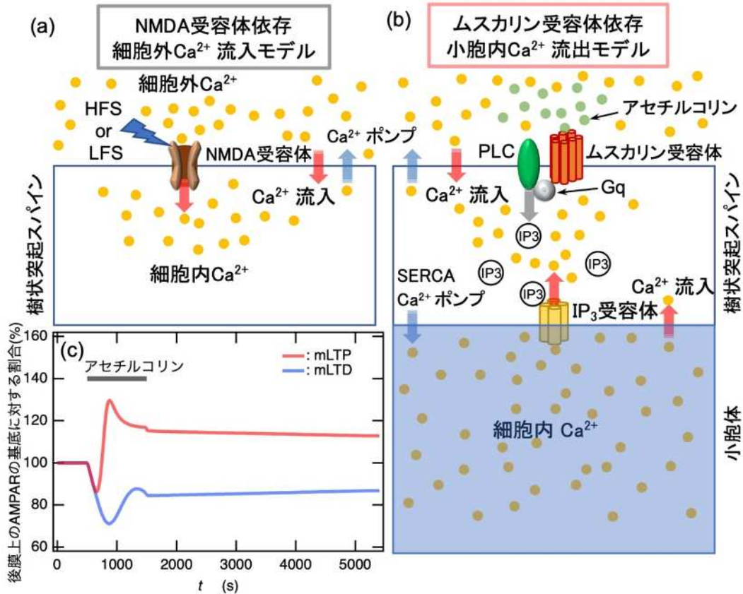
図 2. NMDA 型グルタミン酸受容体(NMDAR)及びムスカリン性アセチルコリン受容体(mAChR)によって介在される樹状突起スパイン細胞質への Ca^{2+} イオンの流入。(a) NMDAR の活性化による細胞外 Ca^{2+} イオンのスパイン細胞質への流入。(b) mAChR の活性化による小胞体内に蓄えられた細胞内 Ca^{2+} イオンのスパイン細胞質への流出。(c) mAChR の活性化に伴うシナプス後膜上 AMPAR 数の、基底状態に対する割合の時間変化。
