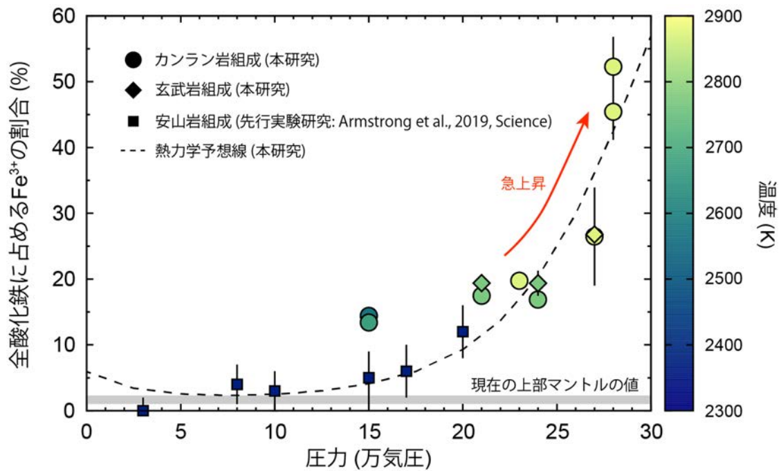
図3. 本研究から明らかとなった金属鉄共存化におけるマグマ中の酸化鉄に占めるFe 3+ の割合の変化。下部マントル圧力条件（23万気圧以上）では、2価鉄の電荷不均化反応の効率が非常に高くなる。
