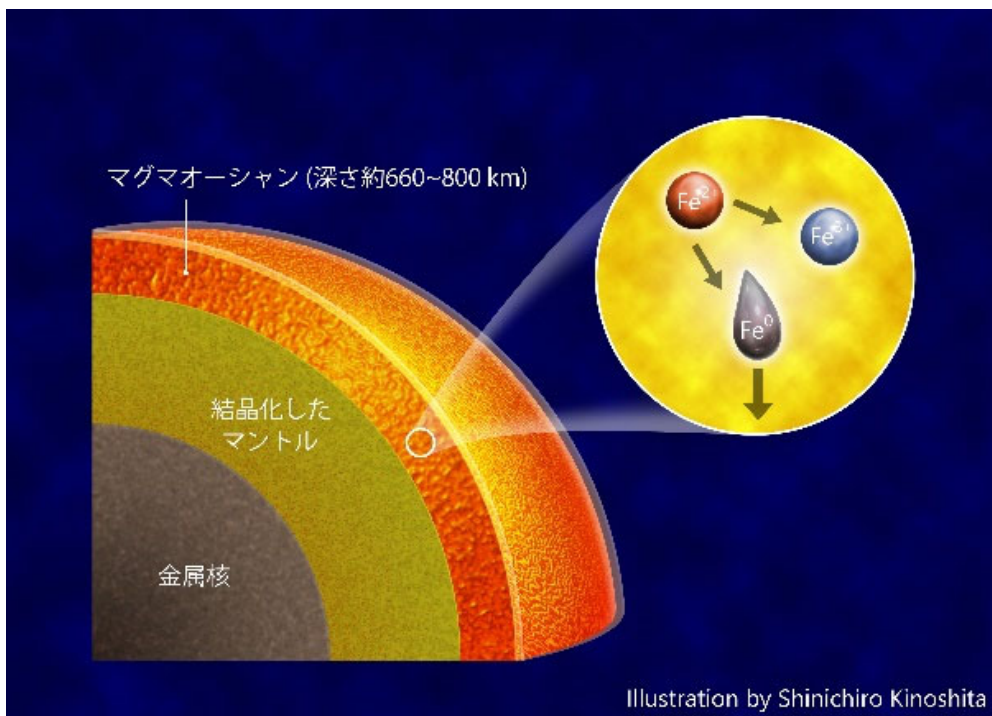
図1. 巨大天体衝突の想像図(上)と2価鉄の不均化反応によるマグマオーシャン酸化メカニズムの概要(下)。2価鉄( \text{Fe}^{2+} )の不均化反応により生成した金属鉄がマグマオーシャンから取り除かれ、3価鉄( \text{Fe}^{3+} )の割合が増加し、マントルが酸化する。
