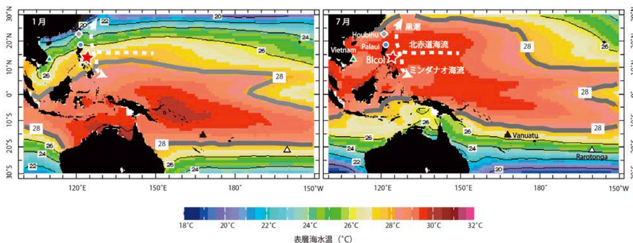
図 1：サンゴ骨格試料採取位置（赤い星印）周辺の 1 月と 7 月の表層海水温分布（1981-2010 年の平均値）。1 年を通して 28^{\circ}\text{C} で囲まれた海域が WPWP に相当する。図中の Houbihu, Palau, Vietnam は比較に用いた先行研究（Houbihu: Ramos et al., 2020; Palau: Ramos et al., 2019; Goodkin et al., 2021）が行われた地点である。Paleoceanography and Paleoclimatology 誌に掲載された図を改変。
