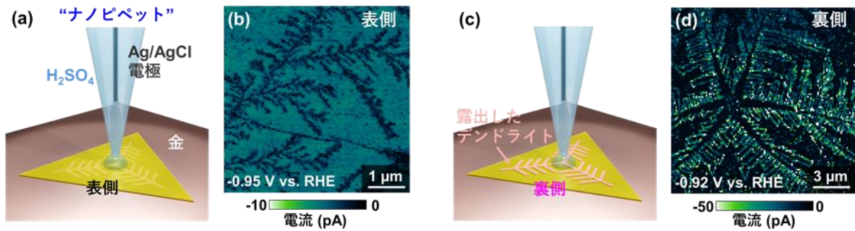
図 2. (a,c) WS 2 結晶の(a,b) 表側と(c,d) 裏側の(a,c) SECCM 測定の模式図と(b,d) 電流マップ。
