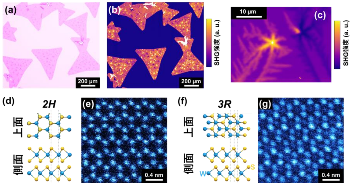
図 3. WS_2 結晶の(a) 光学顕微鏡と(b) 大面積 SHG マップ。(c) 異なる SHG 強度をもつ二つのデンドライトの SHG マップ。2H および 3R 積層した二層 WS_2 の(d,f) 結晶モデルと(e,g) 高分解 STEM 像。
