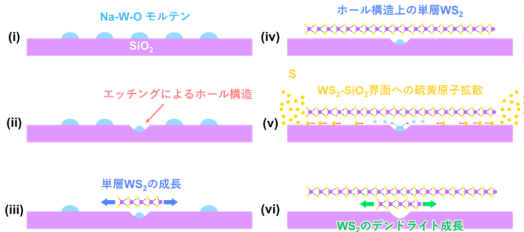
図 4. WS_2 デンドライトの界面成長のモデル。
