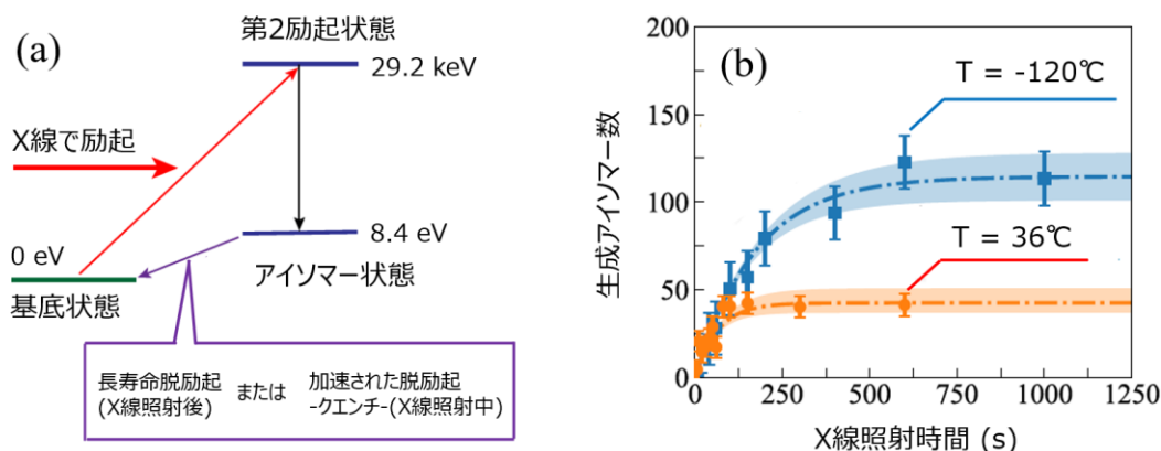
図 1 (a) トリウム 229 準位図（関係する基底状態及び励起状態）。(b) X 線照射時間に対する生成アイソマー数の増加の測定データ。室温( 36^{\circ}\text{C} )と低温( -120^{\circ}\text{C} )の比較。
