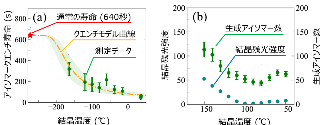
図 2 (a) アイソマークエンチの寿命と温度の関係。(b) 生成アイソマー数および結晶残光強度と結晶温度との関係。
