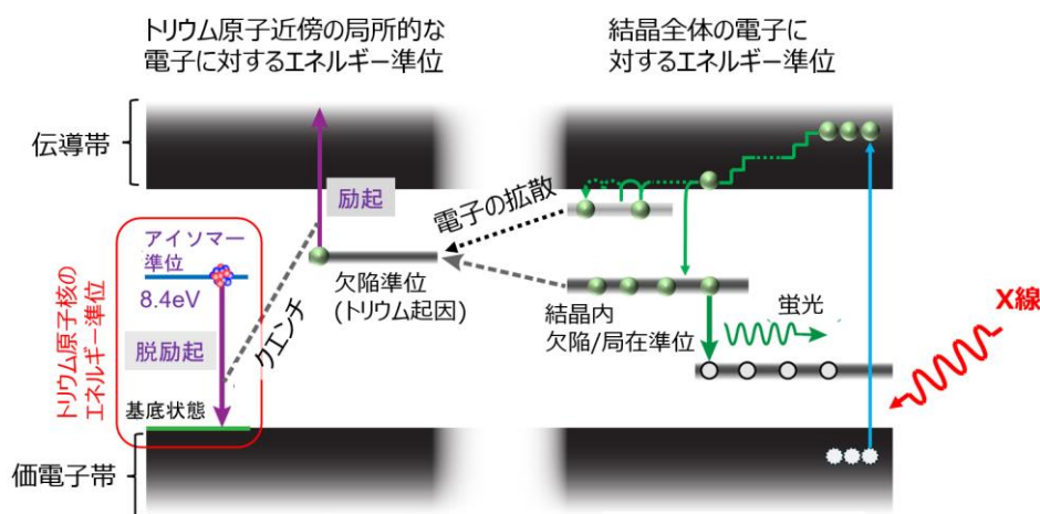
図 3 得られた測定データをもとに構築したアイソマーのクエンチモデル。結晶に X 線を入射して励起された電子が \text{CaF}_2 結晶中を拡散し、その一部がトリウム近傍の欠陥準位にトラップされてトリウム 229 アイソマーにある原子核と相互作用してクエンチが生じる。
