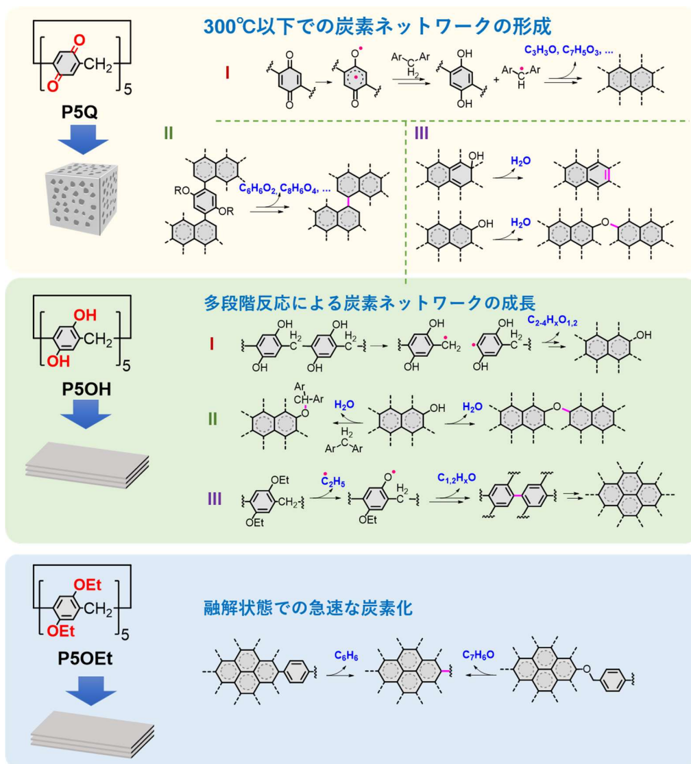
図2. 各ピラーアレーンの炭素化挙動
