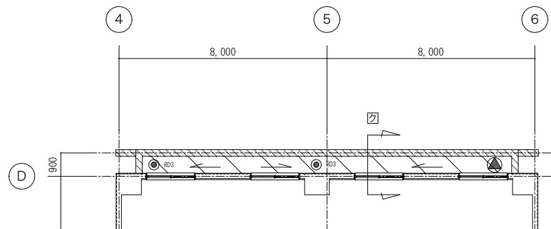
1階パラベット平面図 1/100
