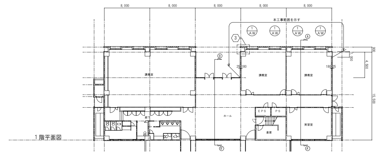
各階平面図 S=1/200
