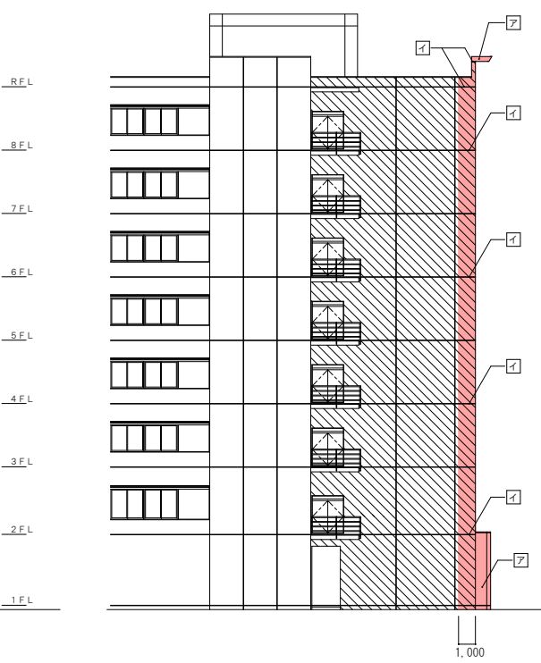
東立面図 S=1/200
