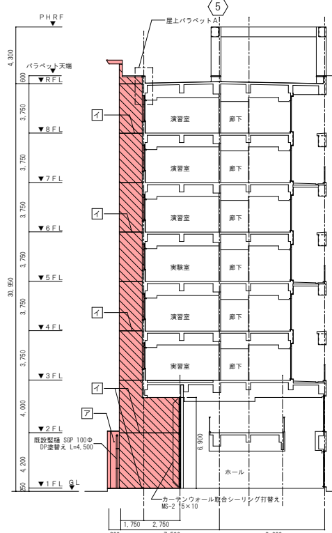
⑤-② 断面図 S=1/200
