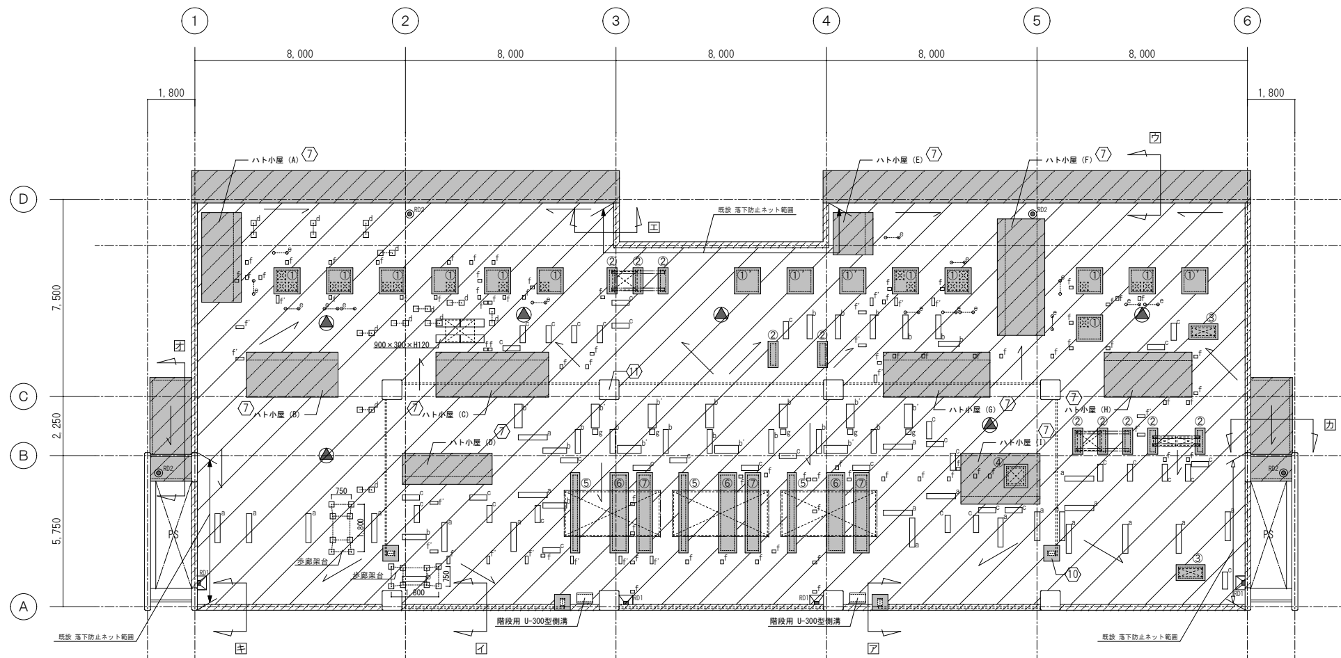
屋上平面図 1/100
