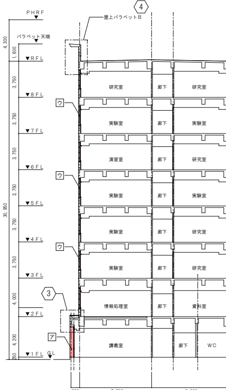
④-① 断面図 S=1/200
