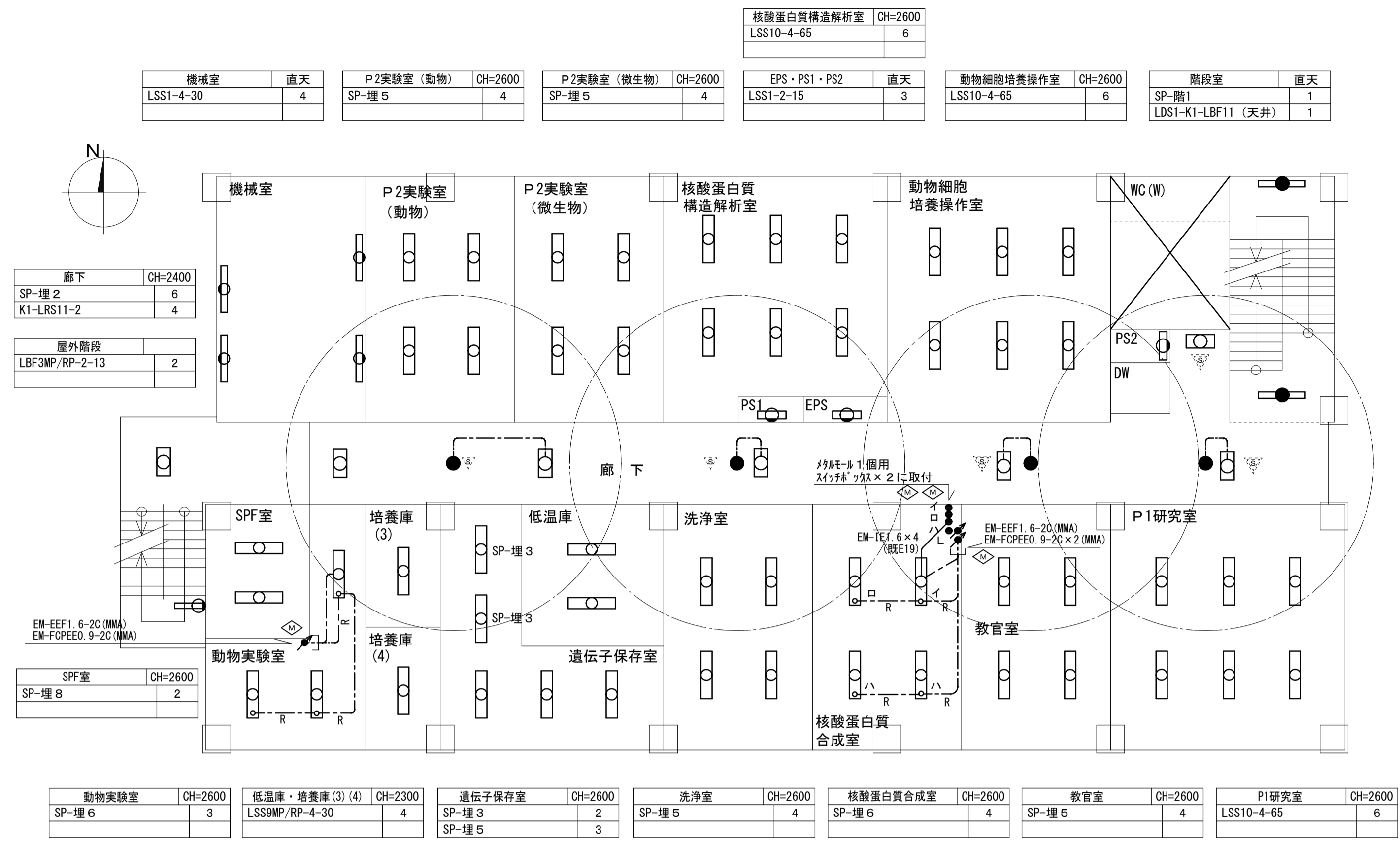
ゲノム・プロテオーム解析部門2階 電灯分岐設備 改修配線図 S=1/100
