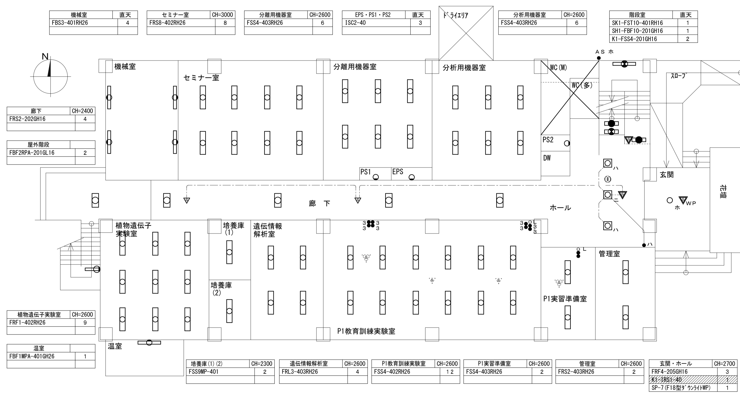
ゲノム・プロテオーム解析部門1階 電灯分岐設備 撤去配線図 S=1/100
