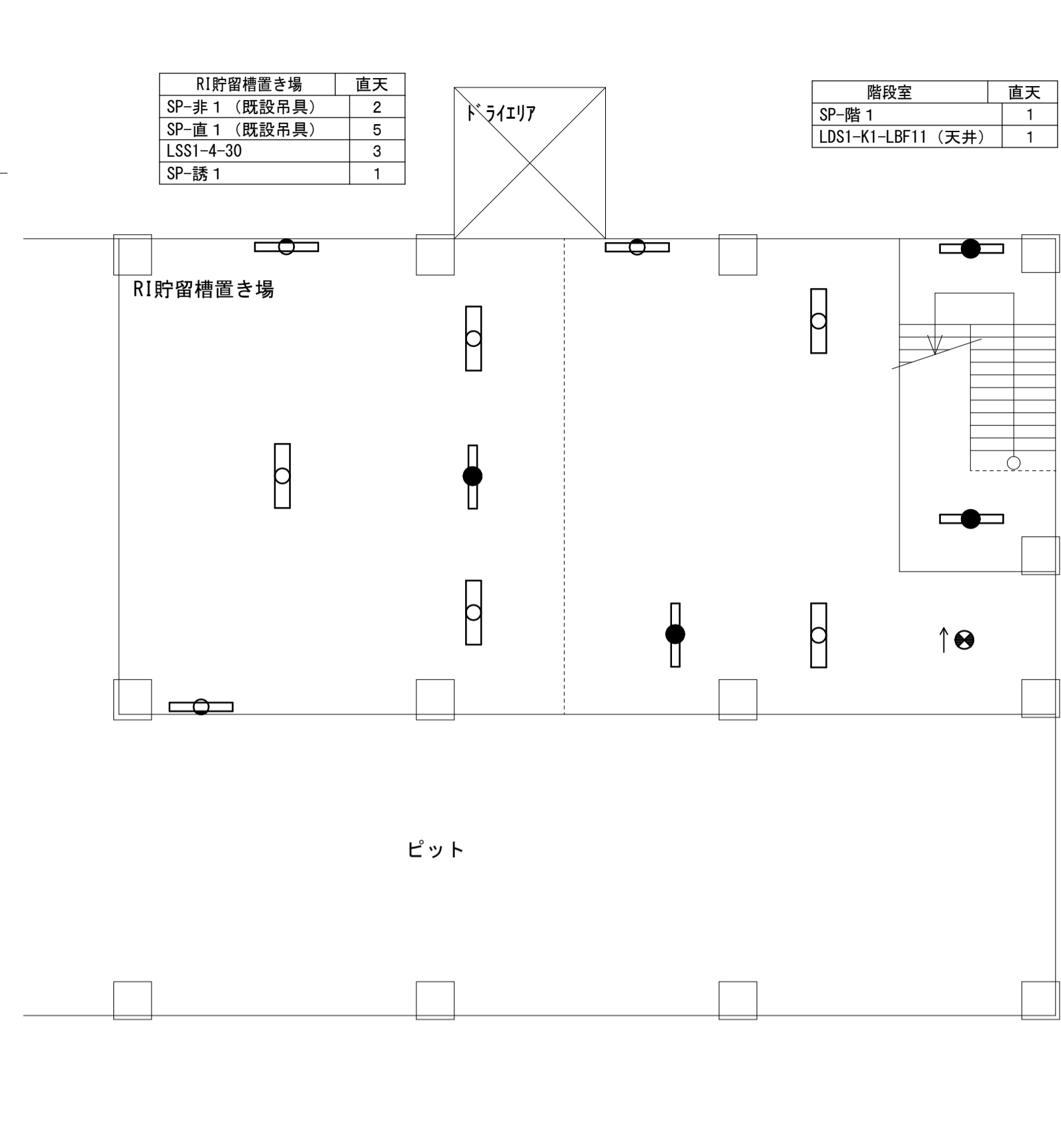
ゲノム・プロテオーム解析部門ピット階 電灯分岐設備 改修配線図 S=1/100
