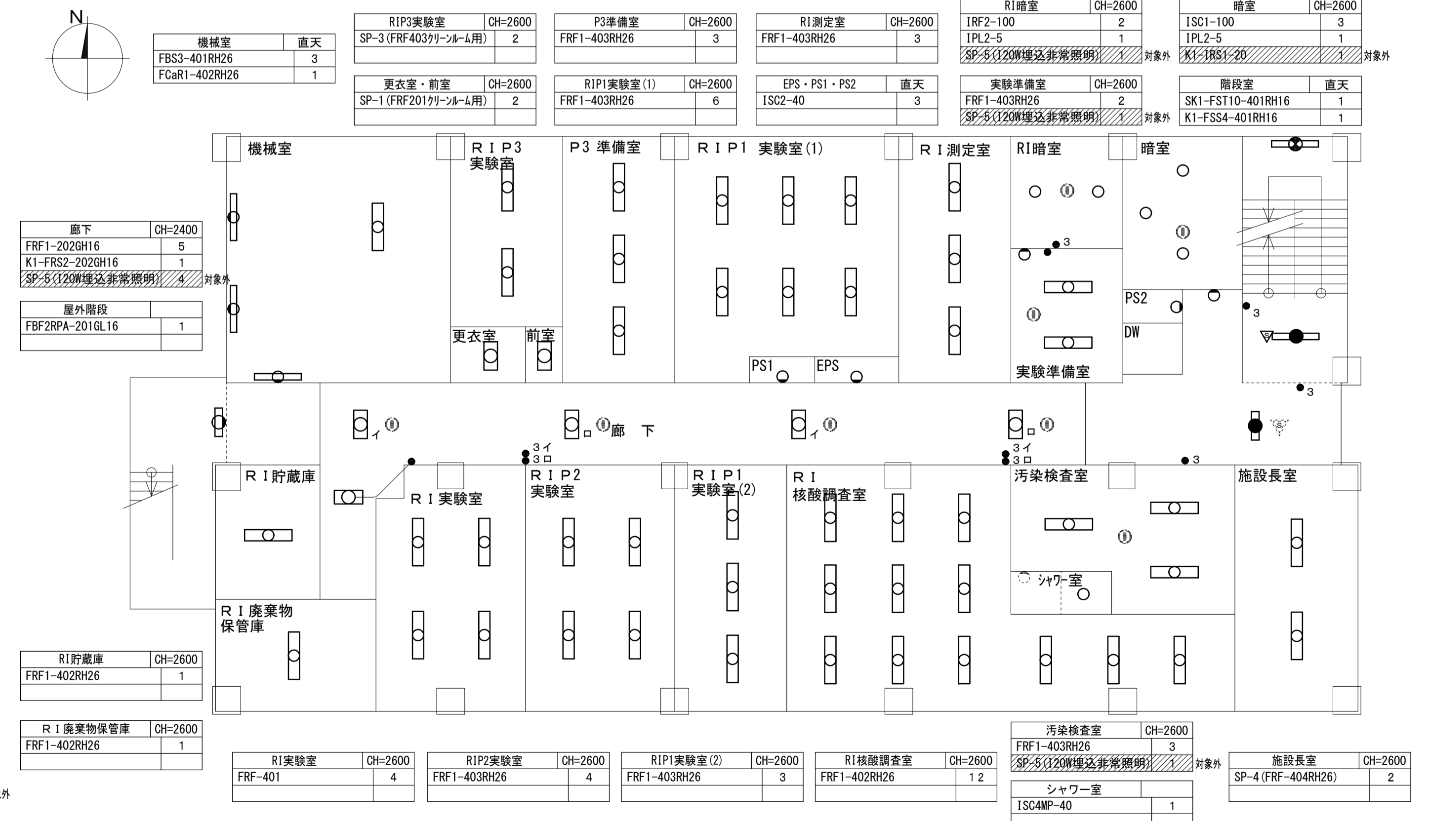
ゲノム・プロテオーム解析部門3階 電灯分岐設備 撤去配線図 S=1/100
