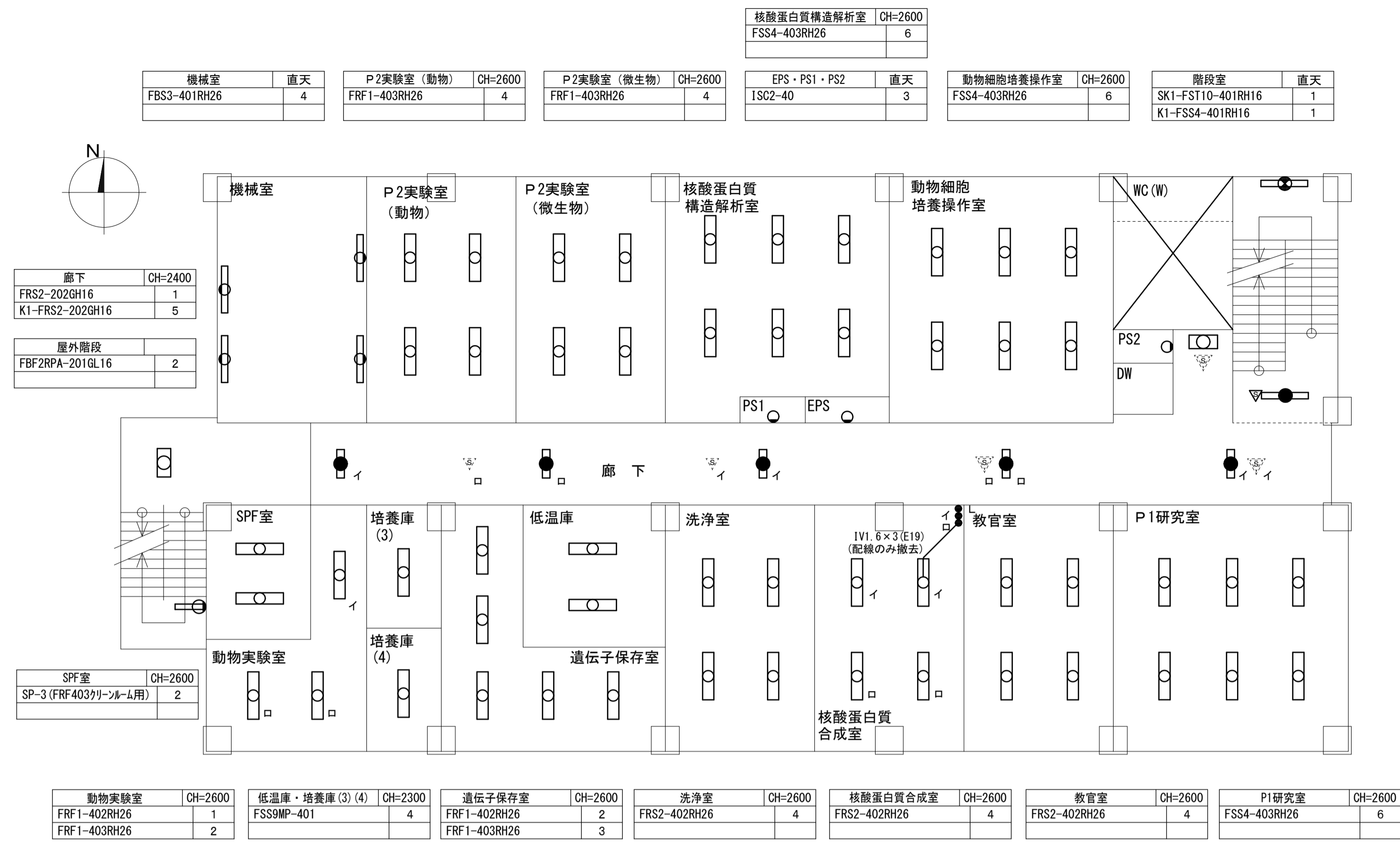
ゲノム・プロテオーム解析部門2階 電灯分岐設備 撤去配線図 S=1/100
