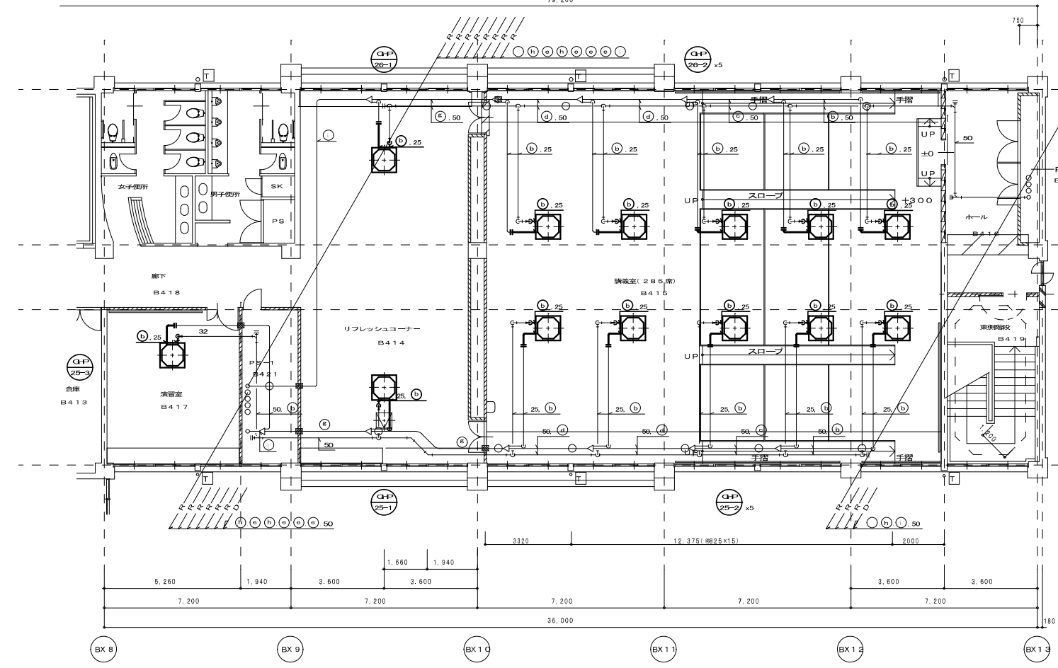
空調設備 4階平面図(改修後) S-1/100
