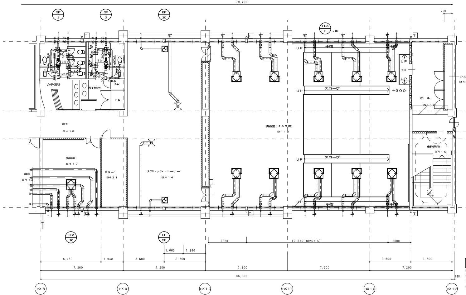
換気設備 4階平面図 (改修後) S-1/100 ※1. 太線は新設を示し、細線は既設を示す。 2. 配線図の再確認を行うこと。 ※全熱交換機後長期間換気ダクト 共通200φ ※天井取 表示無き場合は換気ダクト150φ ※OA取入れダクト 共通200φ
