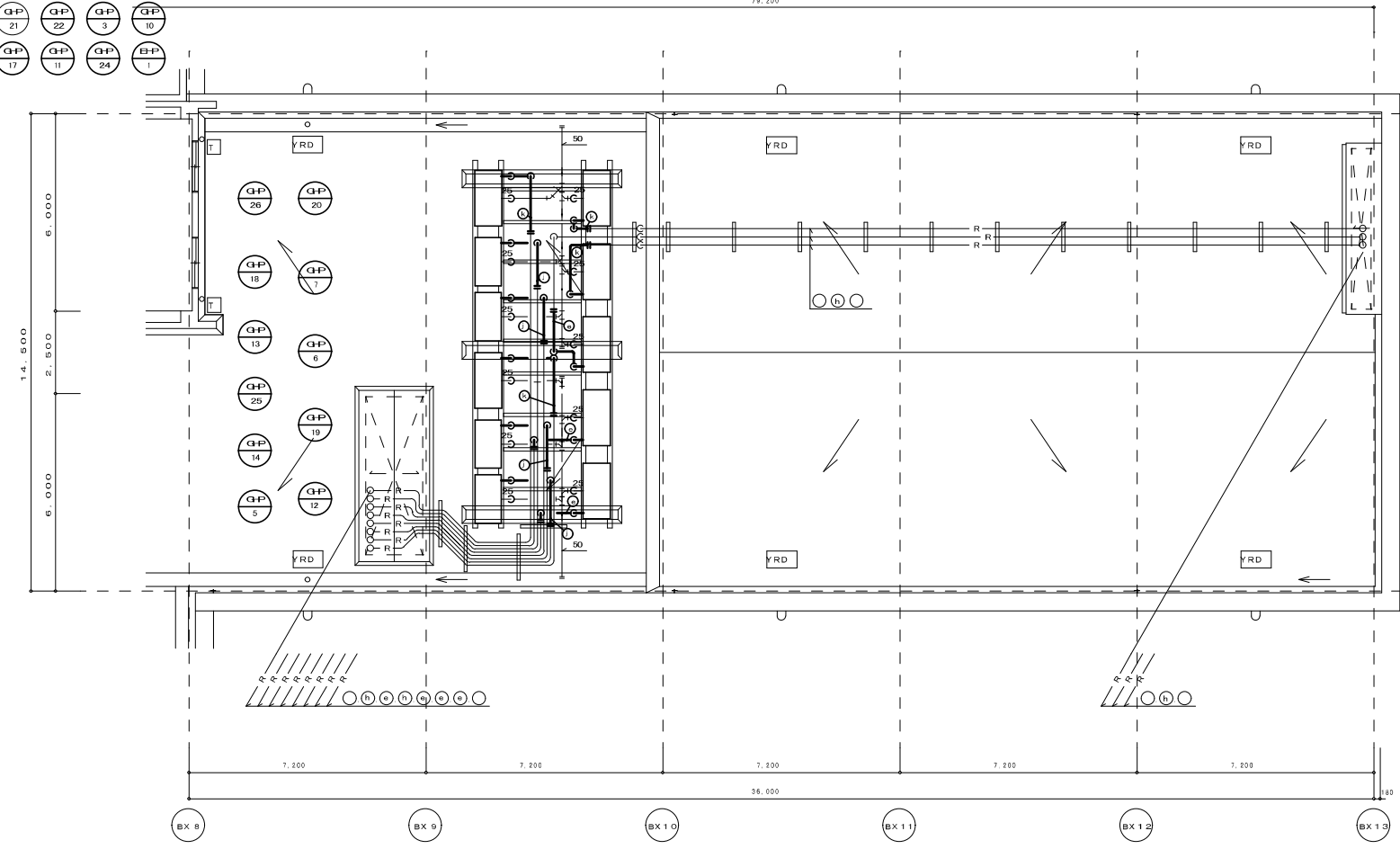
空調設備 R階平面図 (改修後) S-1/100
