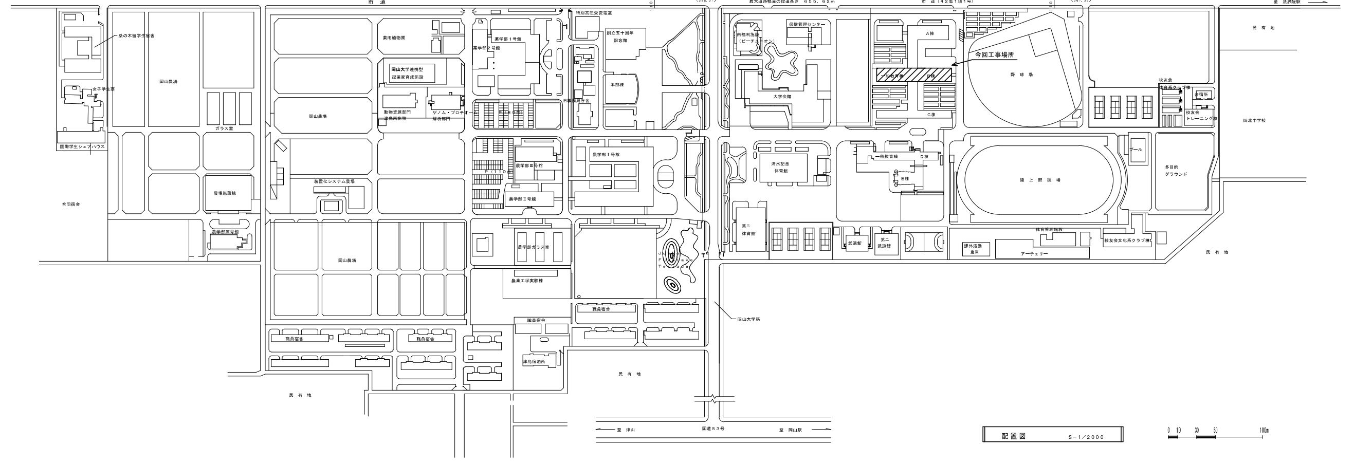
附近見取図
