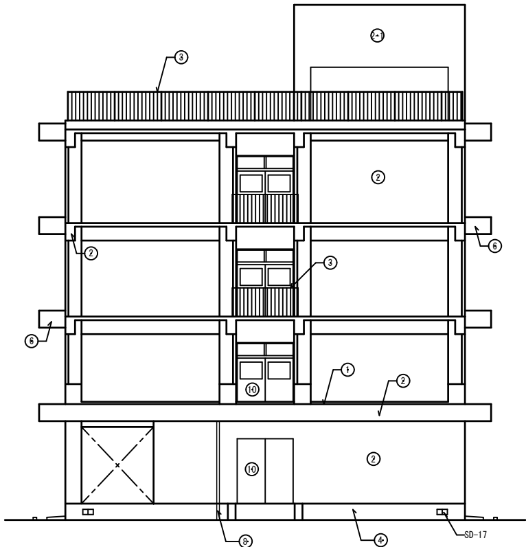
改修前 東立面図 S=1/100
