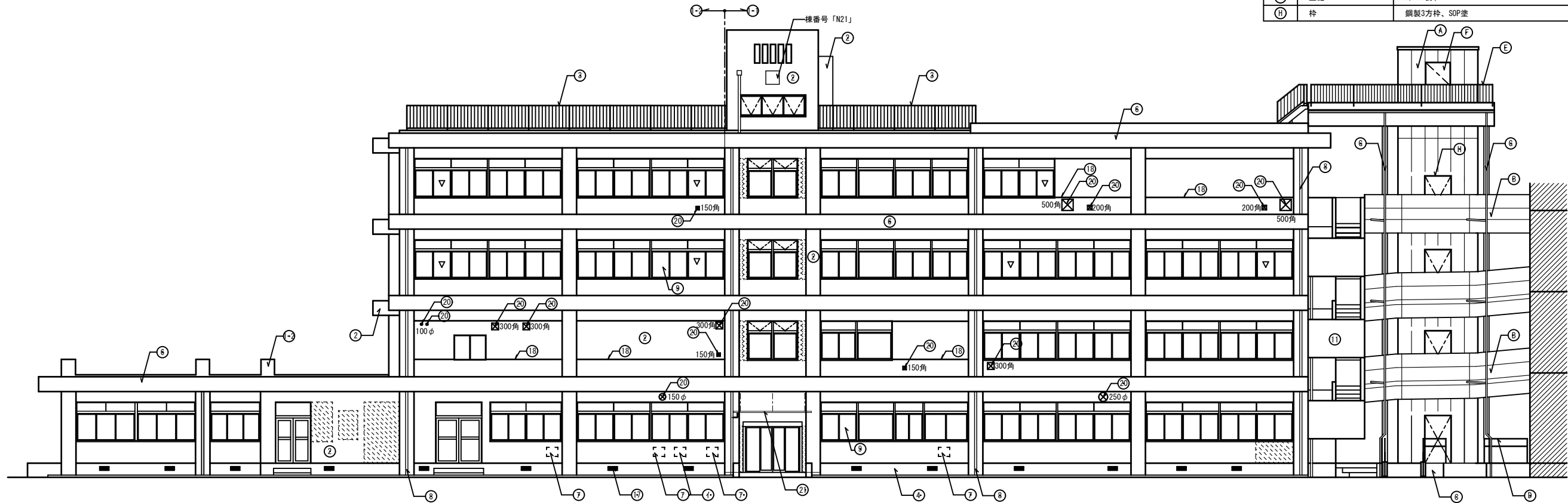
改修後 北立面図 S=1/100
