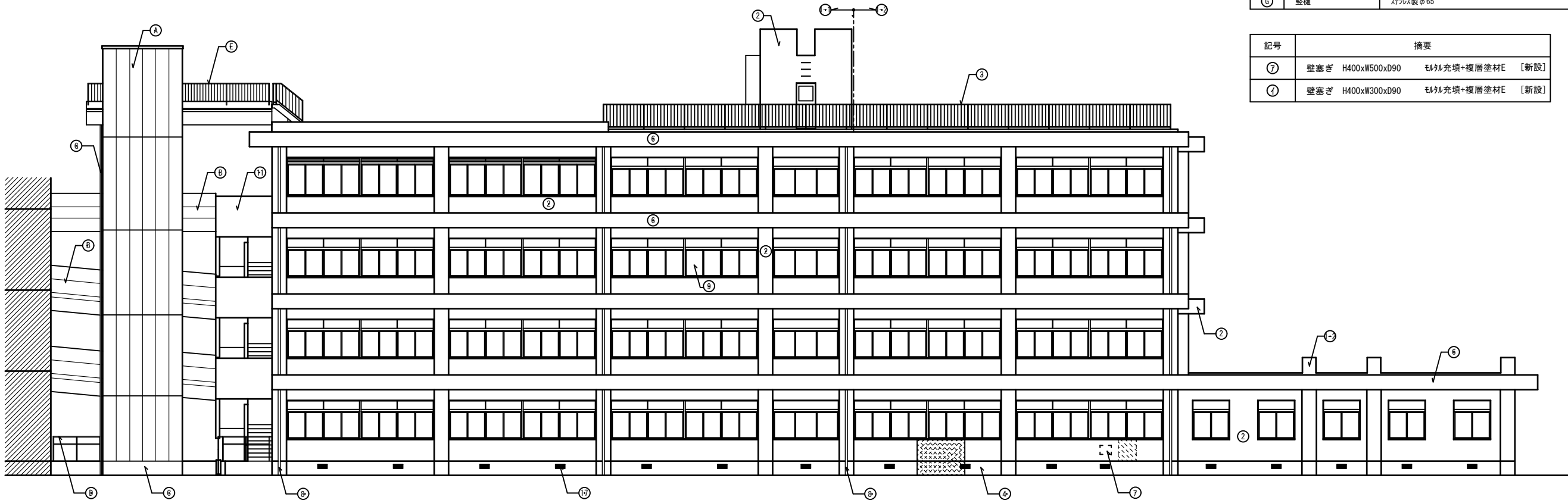
改修後 南立面図 S=1/100
