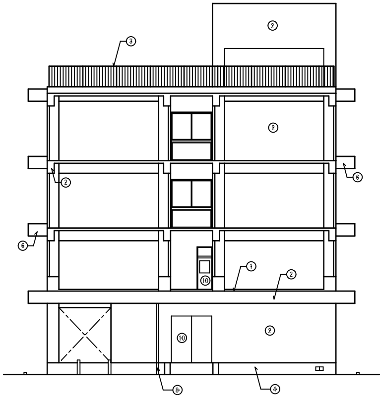
改修後 東立面図 S=1/100
