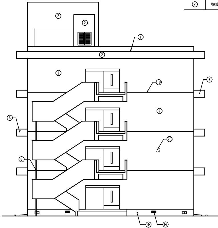
改修後 西立面図 S=1/100
