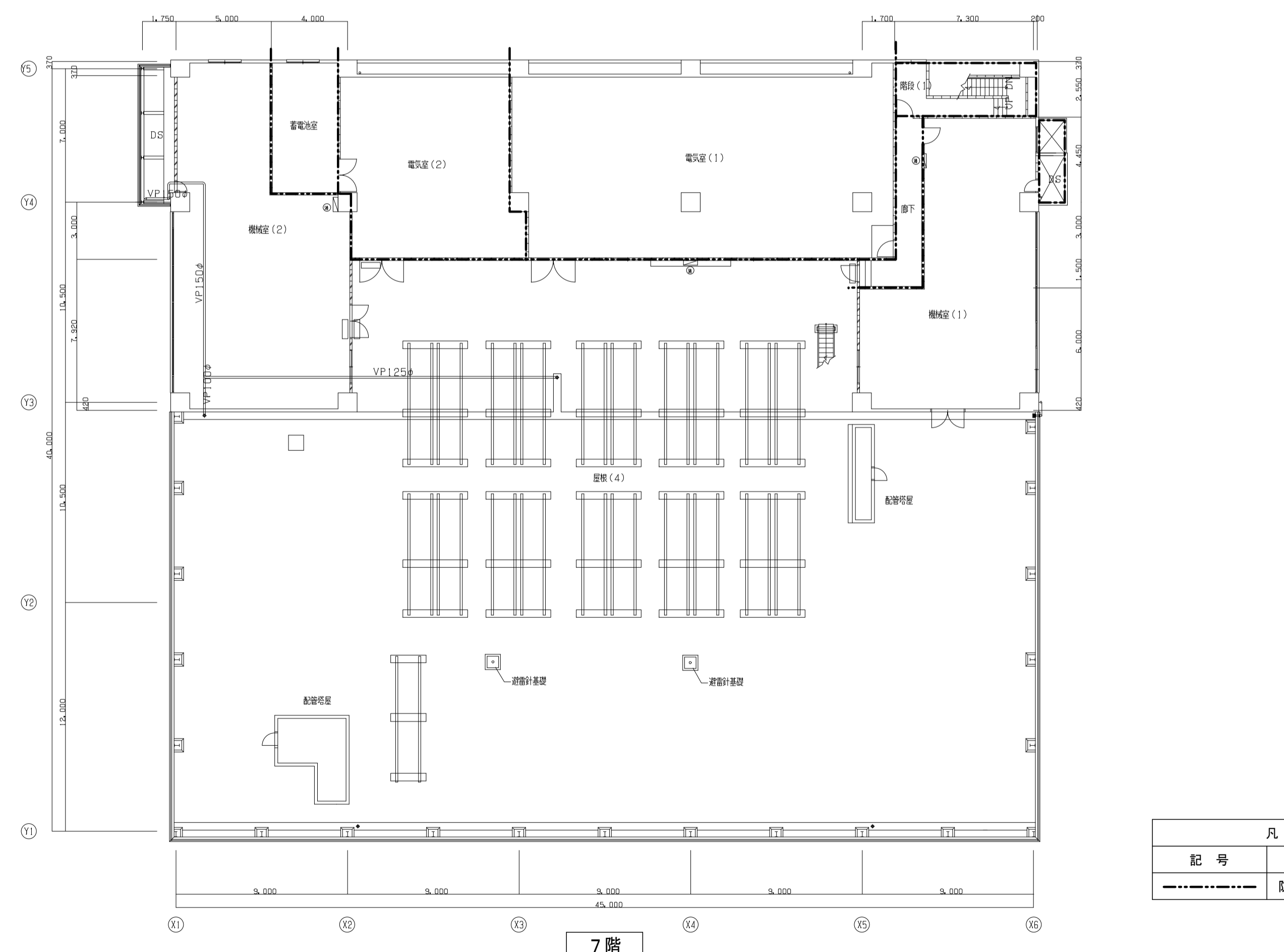
防火区画図 S=1/300
