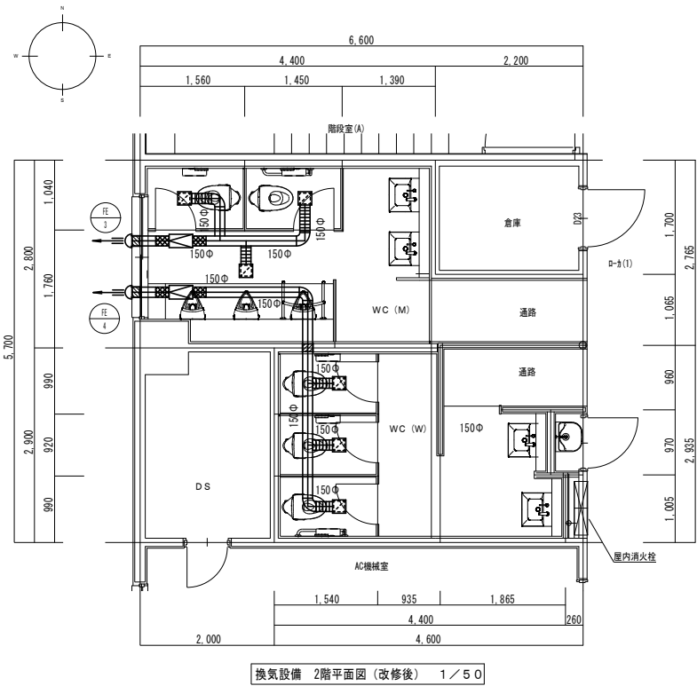
換気設備 2階平面図 (改修後) 1 / 5 0
