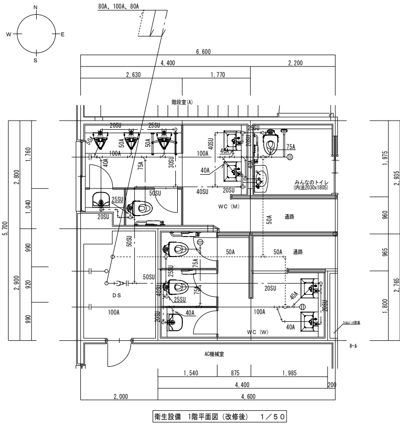
衛生設備 1階平面図 (改修後) 1/50
