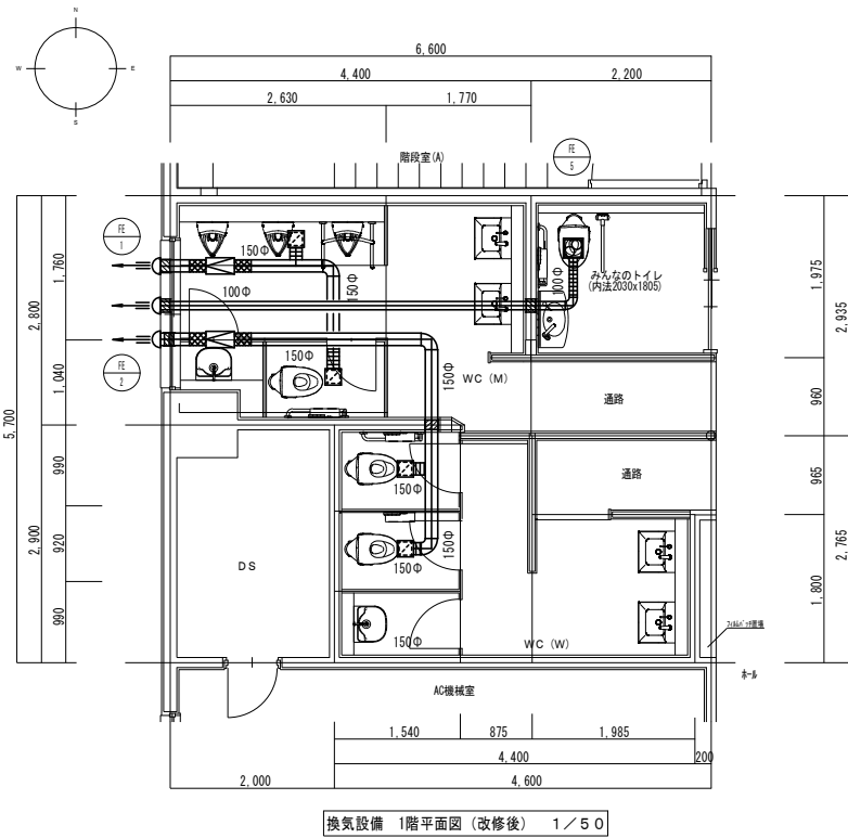
換気設備 1階平面図 (改修後) 1 / 5 0
