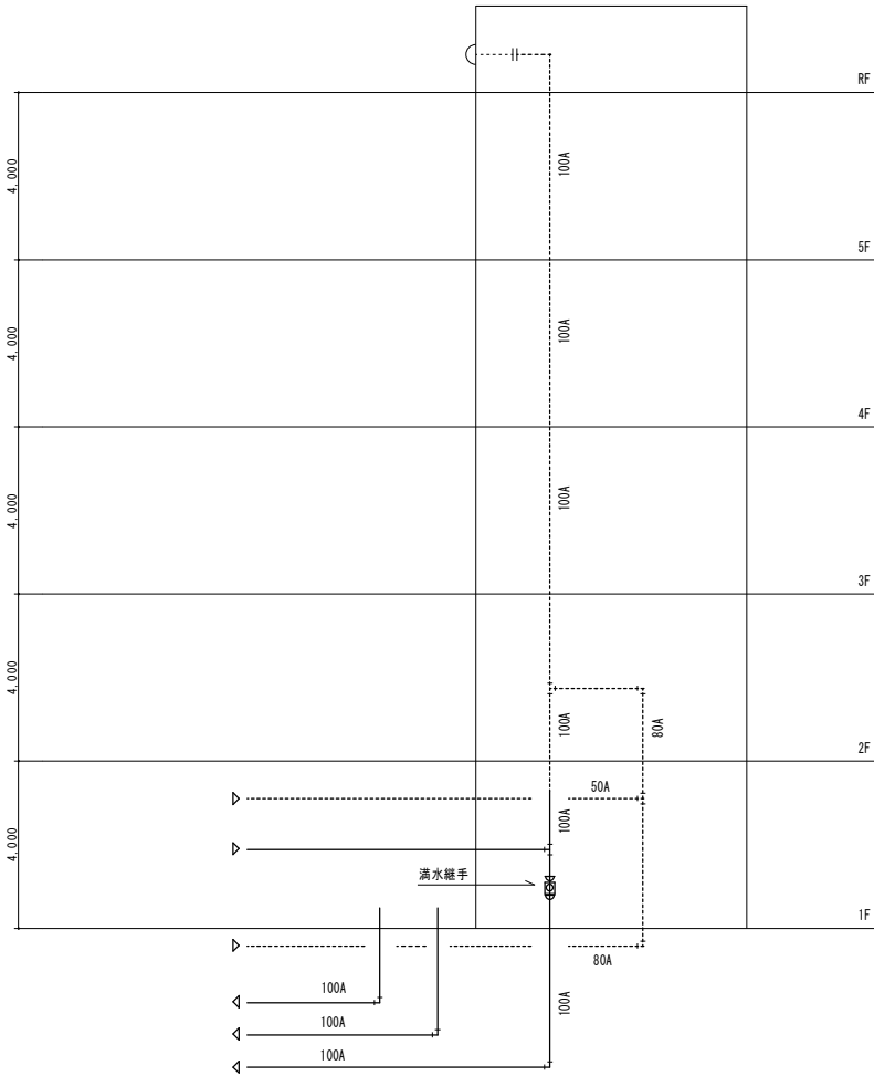
衛生設備 系統図
