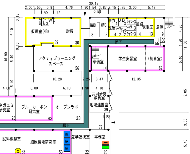
2階平面図 (改修後) 床面積 234㎡ S=1/400
