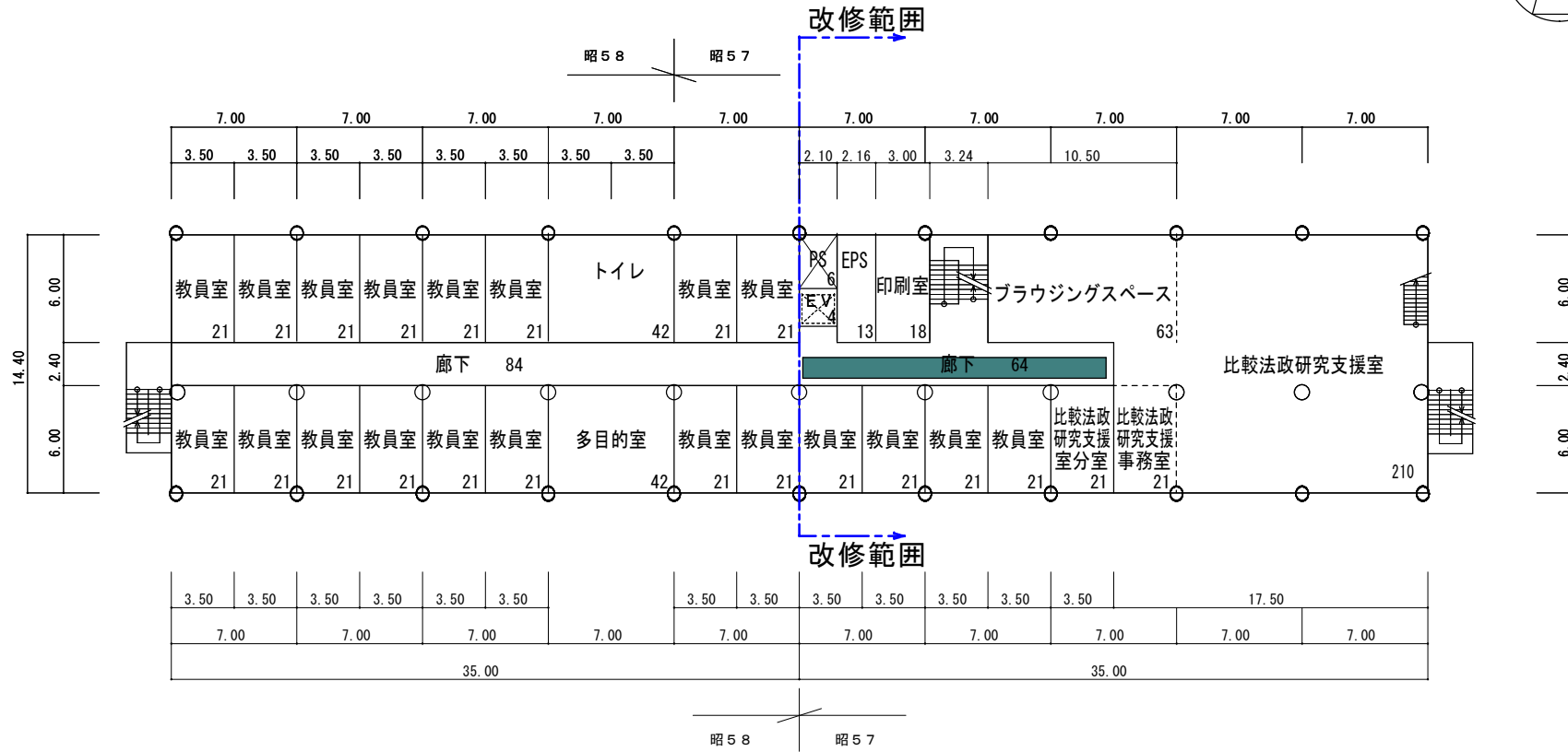
3階平面図 床面積 1008㎡ S=1/400
