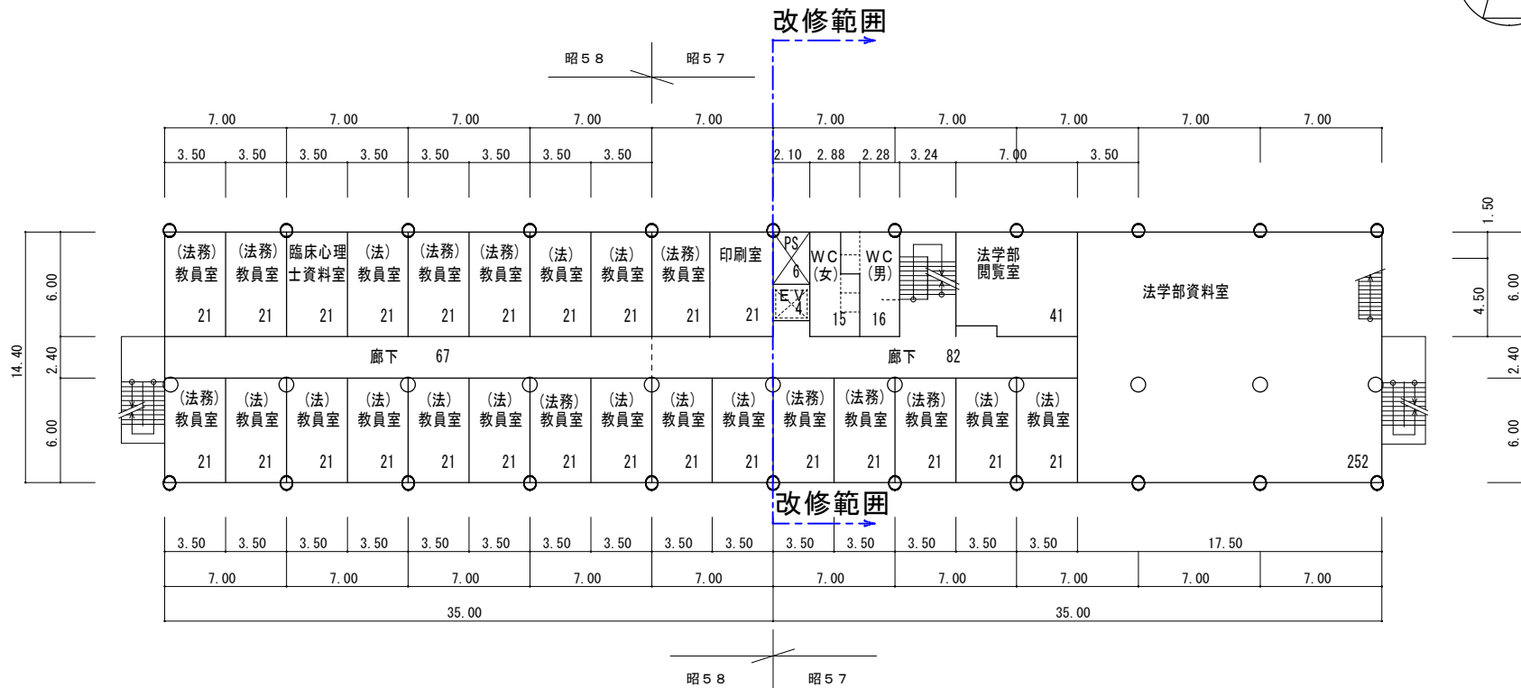
3階平面図 床面積 1008㎡ S=1/400
