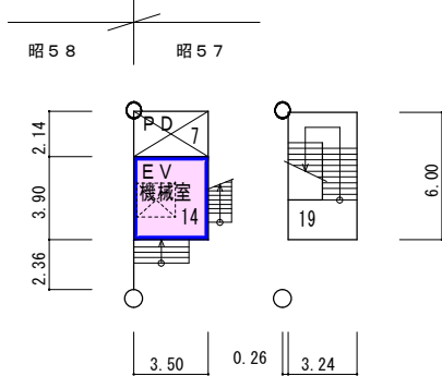
5階平面図 床面積 1008㎡ S = 1/400
