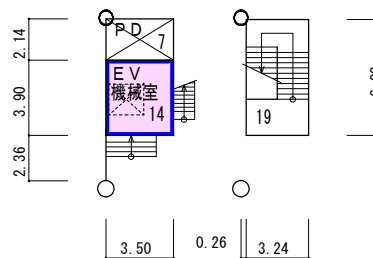
5階平面図 床面積 1008m 2 S = 1 / 400
