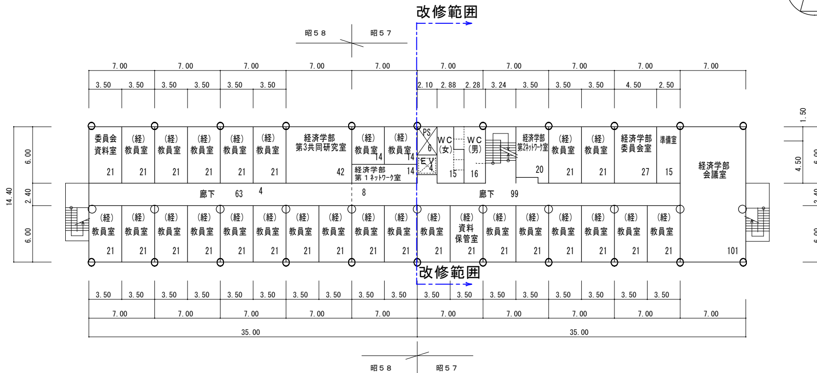
5階平面図 床面積 1008m 2 S = 1 / 400
